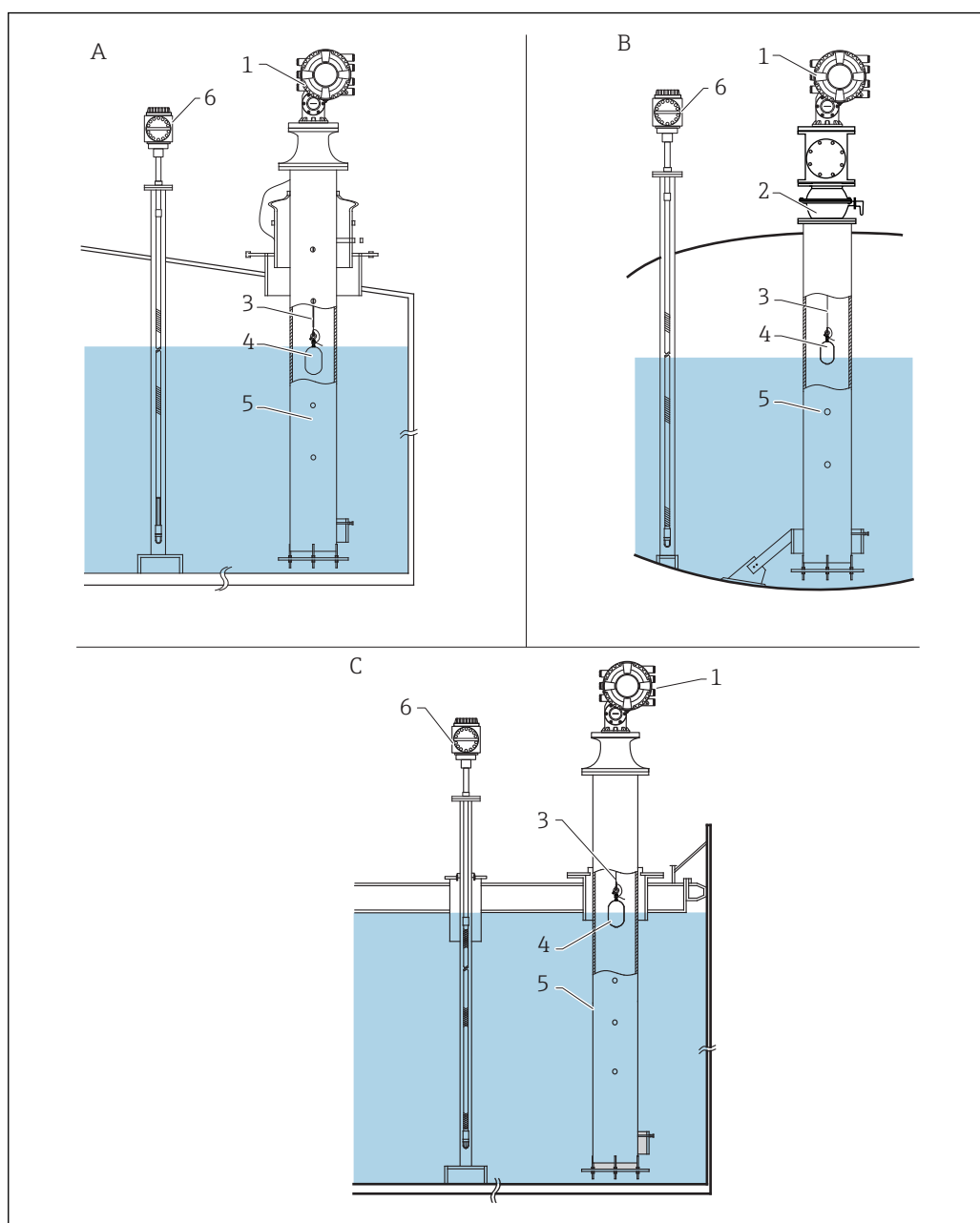
5 Типовой монтаж в резервуаре
