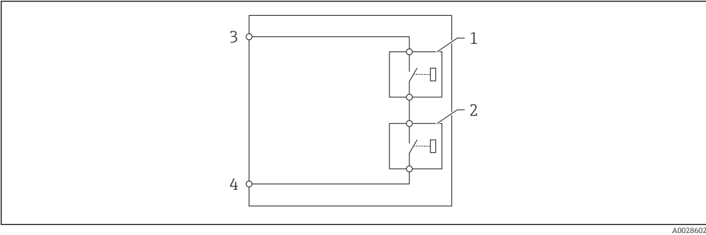
87 Два реле цифрового выхода
