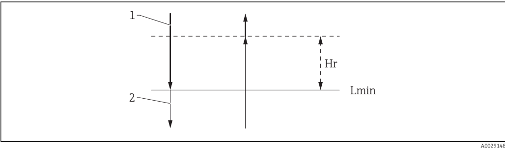
93 Гистерезис функции HTMS 1 Расчетное значение 2 Удерживаемое/введенное вручную значение L_{min} Минимальный уровень (→ 288) H_r Гистерезис (→ 289)
