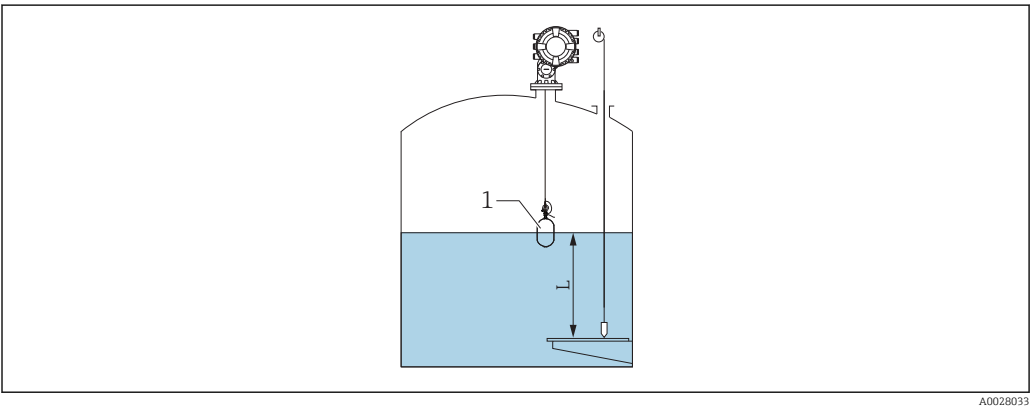
49 Установка уровня для открытого резервуара
