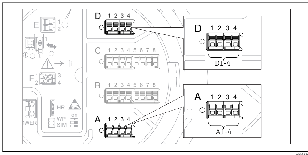
72 Возможное расположение модулей WM550 (примеры); в зависимости от исполнения прибора эти модули также могут находиться в гнезде В или С → 49.
