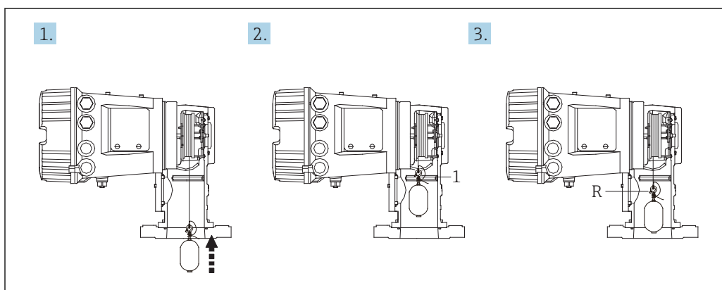
45 Последовательность калибровки начального уровня
