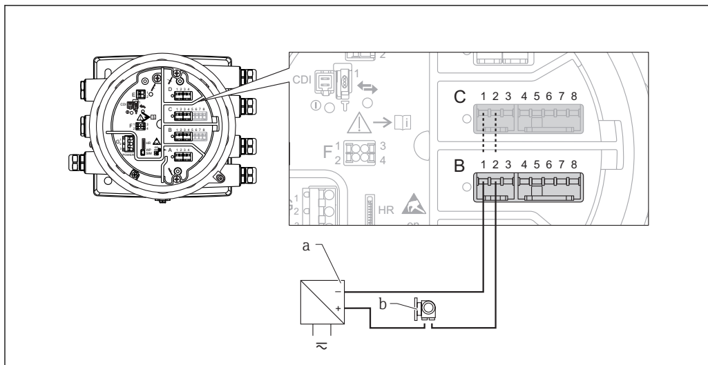
23 Использование модуля аналогового ввода/вывода в режиме пассивного входа
