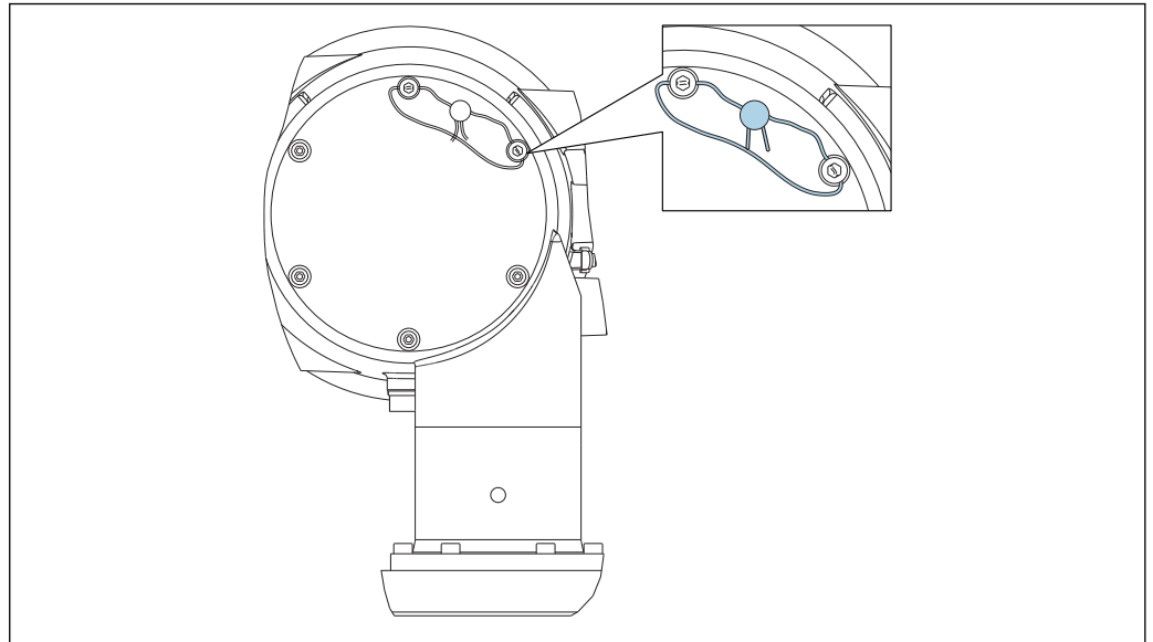
36 Пломбирование задней крышки (на примере NMS80)
