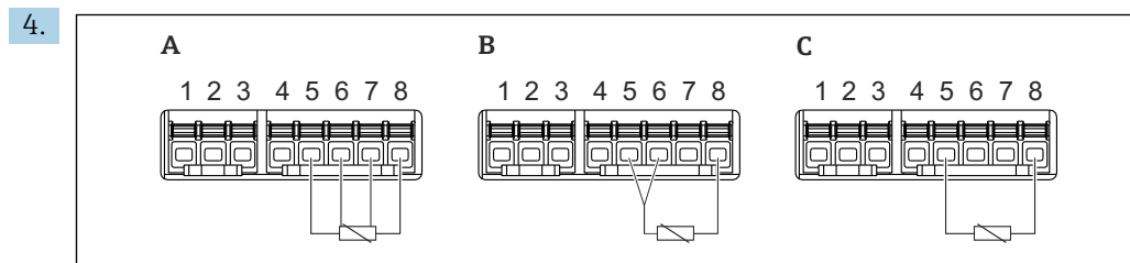
63 Типы подключений RTD
