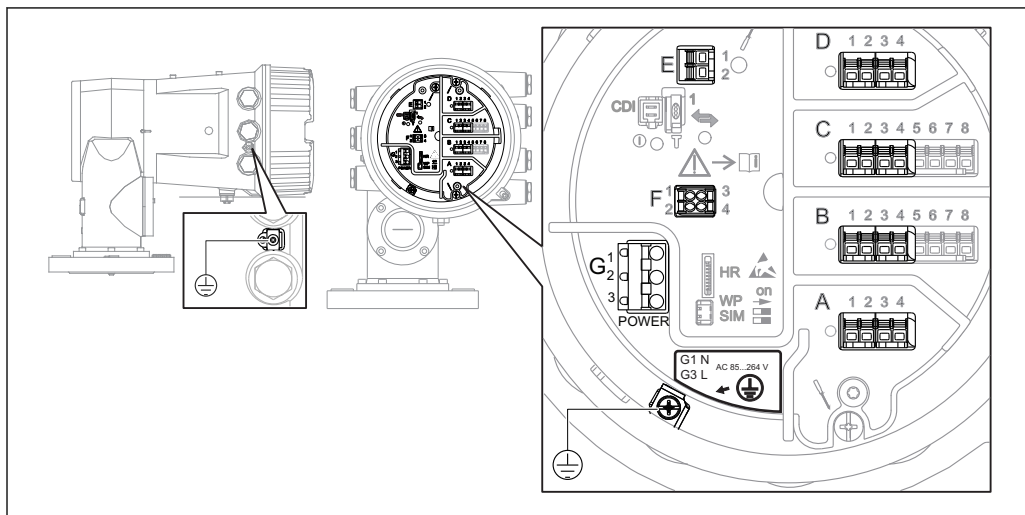
18 Клеммный отсек (типовой пример) и клеммы заземления
