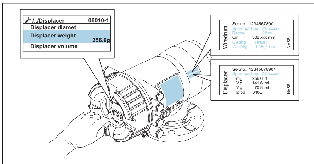
42 Подтверждение данных
