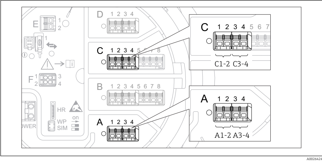
85 Обозначение цифровых входов и выходов (примеры)
