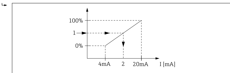
68 Масштабирование переменной резервуара в соответствии с выходным током
