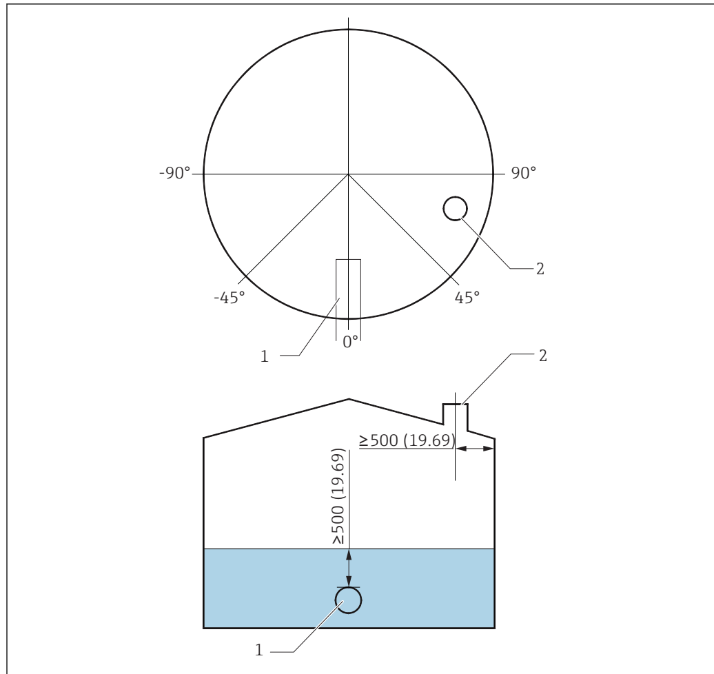
13 Рекомендуемое положение для монтажа прибора NMS8x и минимальный измеряемый уровень, размеры в мм (дюймах)
