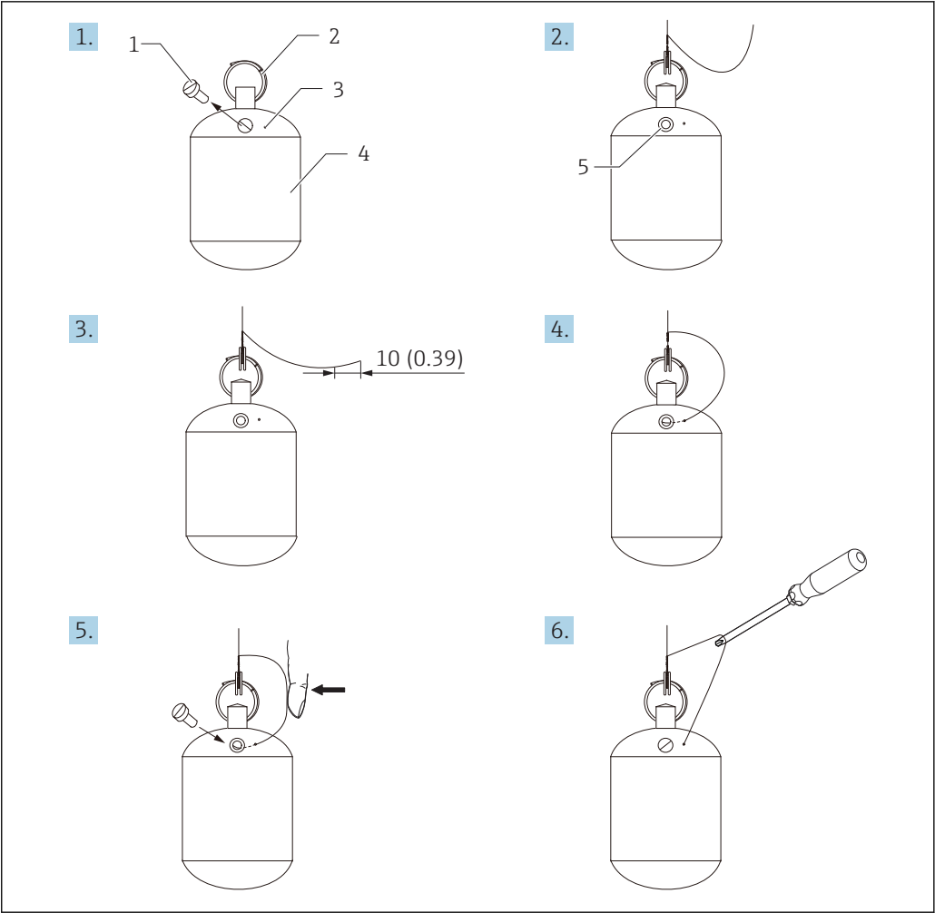
17 Монтаж буйка из ПТФЭ. Размеры даны в мм (дюймах)
