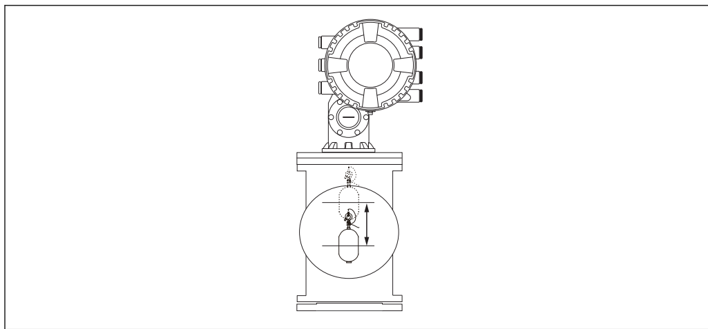
43 Перемещение буйка
