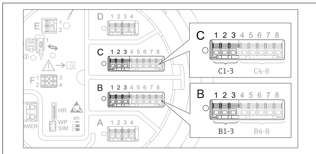
67 Возможное расположение аналоговых модулей ввода/вывода, которые могут использоваться в качестве выхода 4–20 мА. Код заказа прибора зависит от того, какие из этих модулей фактически присутствуют в приборе → 49
