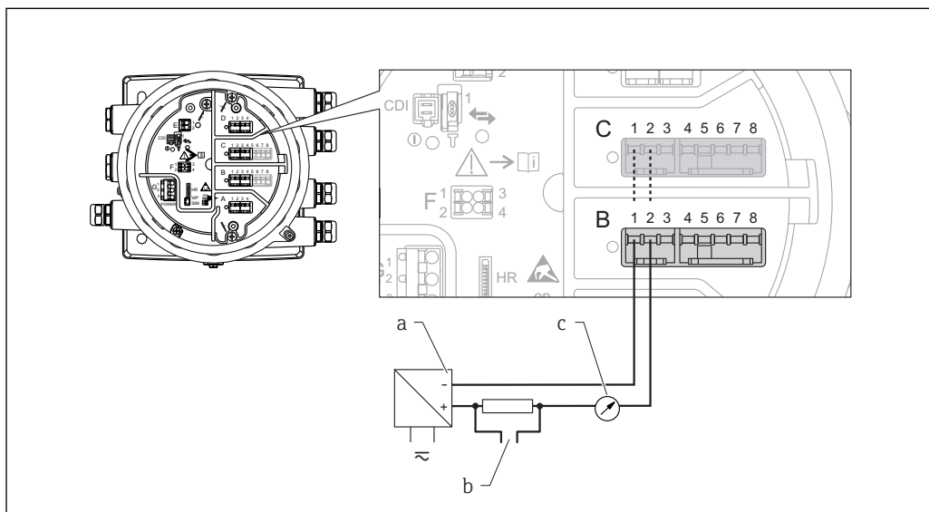
22 Использование модуля аналогового ввода/вывода в режиме пассивного выхода
