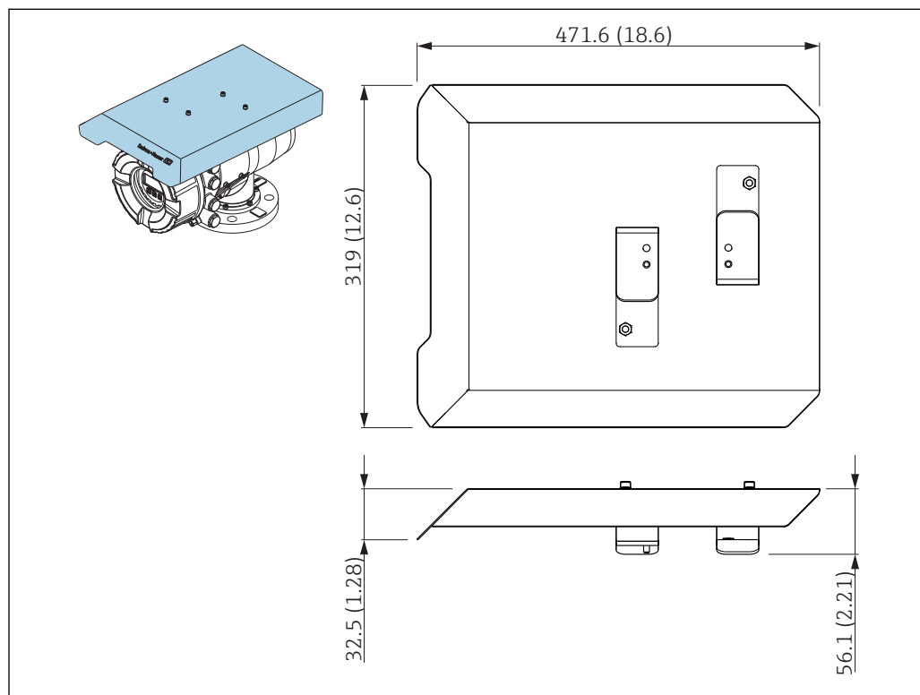
77 Защитный козырек от атмосферных явлений; размеры: мм (дюймы)
