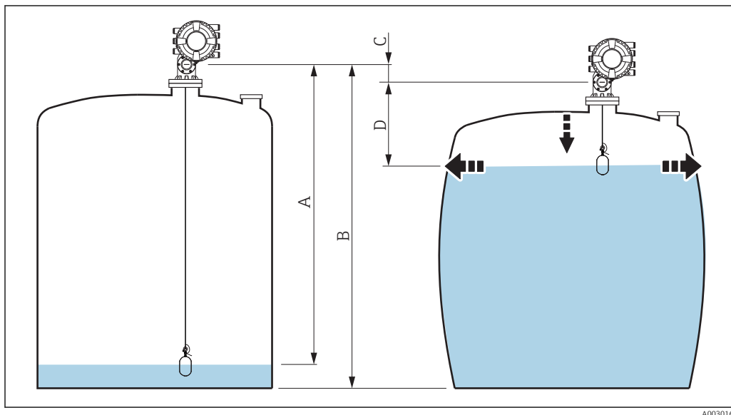
65 Коррекция гидростатической деформации резервуара (HyTD)
