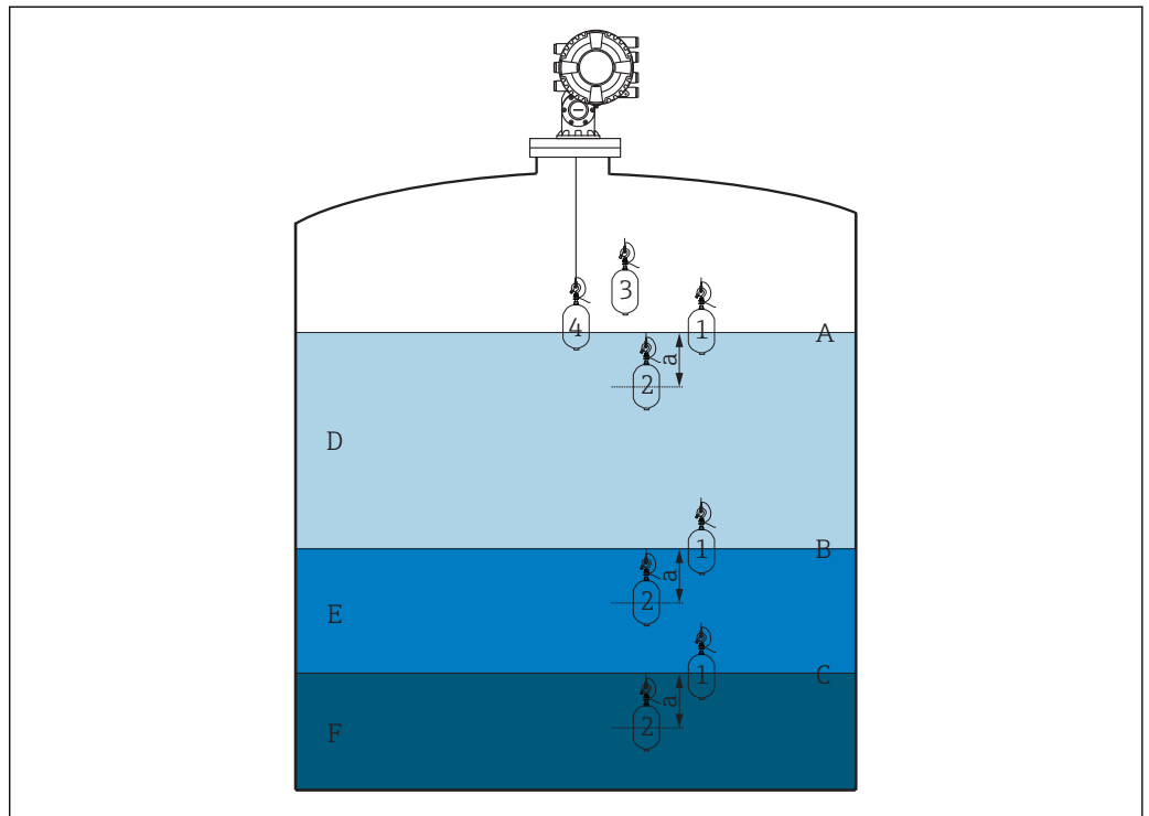
53 Точечная плотность (числа обозначают последовательность движения буйка)
