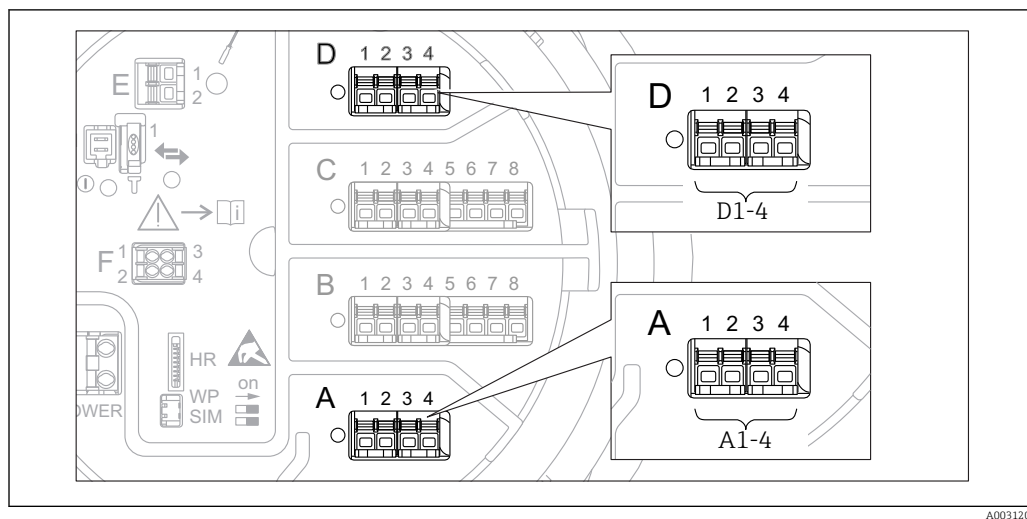
71 Возможное расположение модулей V1 (примеры); в зависимости от исполнения прибора эти модули также могут находиться в гнезде В или С → 49.
