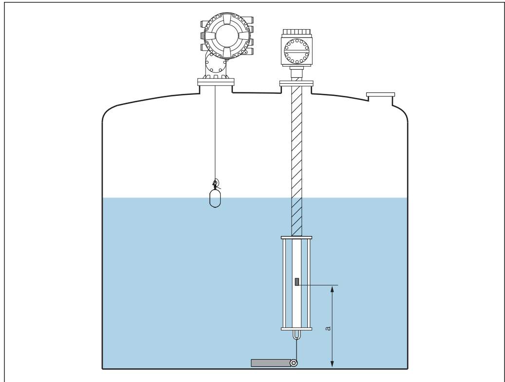
59 Position de l'élément de température du fond
