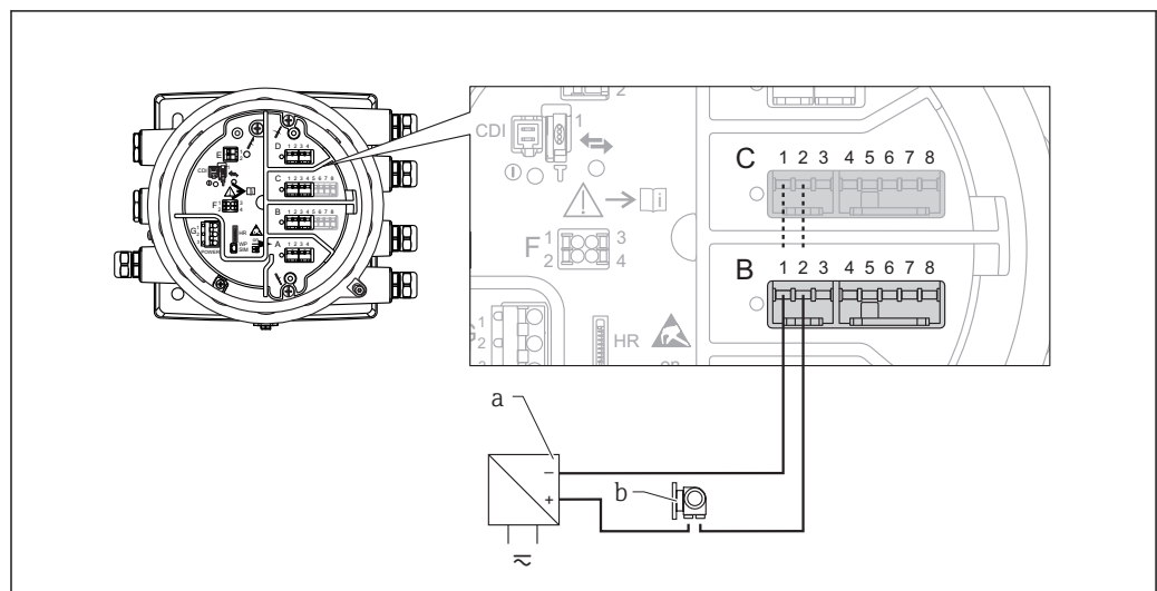
23 Utilisation passive du module Analog I/O en mode entrée
