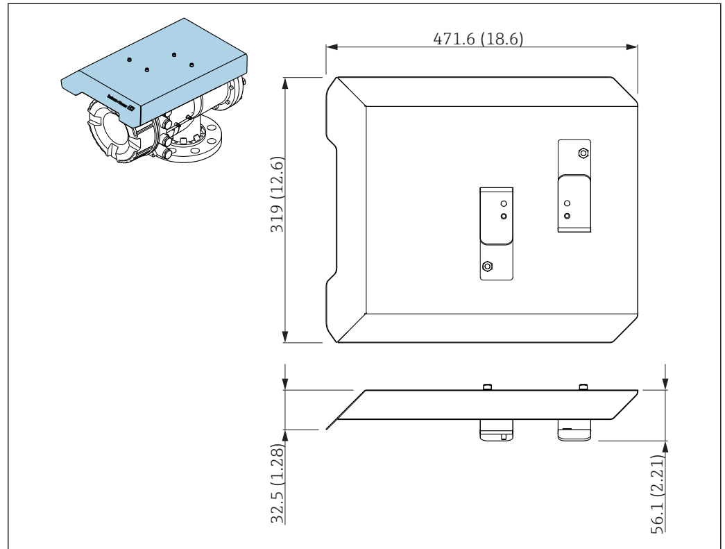
77 Capot de protection climatique ; unité de mesure : mm (in)
