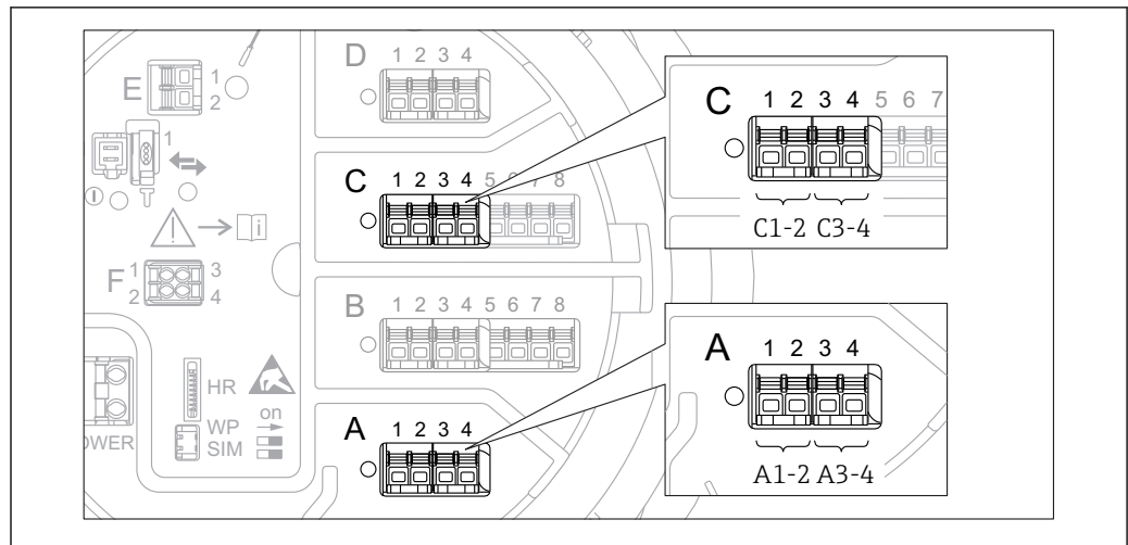
73 Emplacements possibles des modules Digital I/O (exemples) ; la référence de commande détermine le nombre et l'emplacement des modules Digital I/O → 48.
