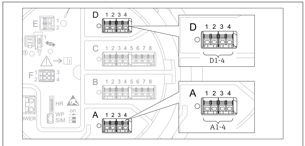
71 Emplacements possibles des modules V1 (exemples) ; selon la version d'appareil, ces modules peuvent également se trouver dans les slots B ou C → 48.
