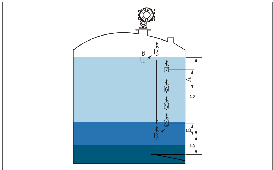
57 Mouvement du profil manuel (les numéros indiquent l'ordre des mouvements du déplacer.)
