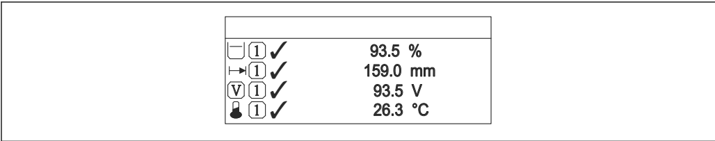
99 "Format d'affichage" = "4 valeurs"
