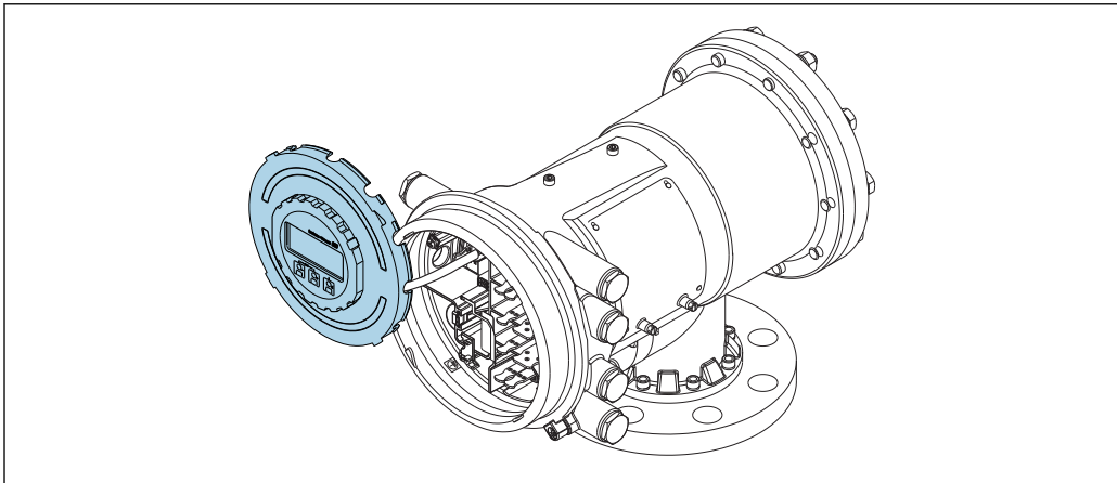
37 NMS81 : Module d'affichage fixé au bord du compartiment de raccordement
