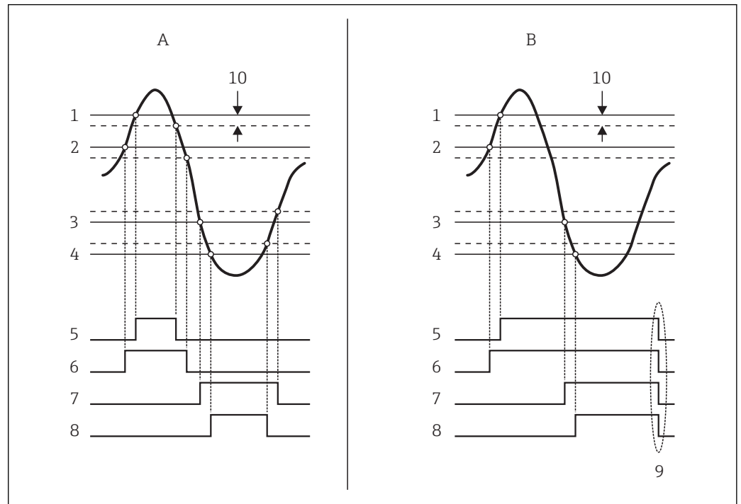
66 Principe de l'évaluation des limites
