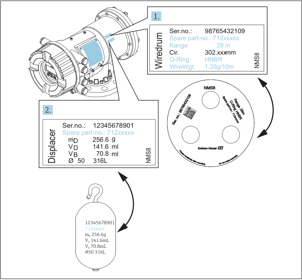
14 Vérification du displacer et du tambour de fil
