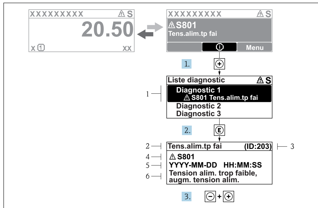
76 Message relatif aux mesures correctives
