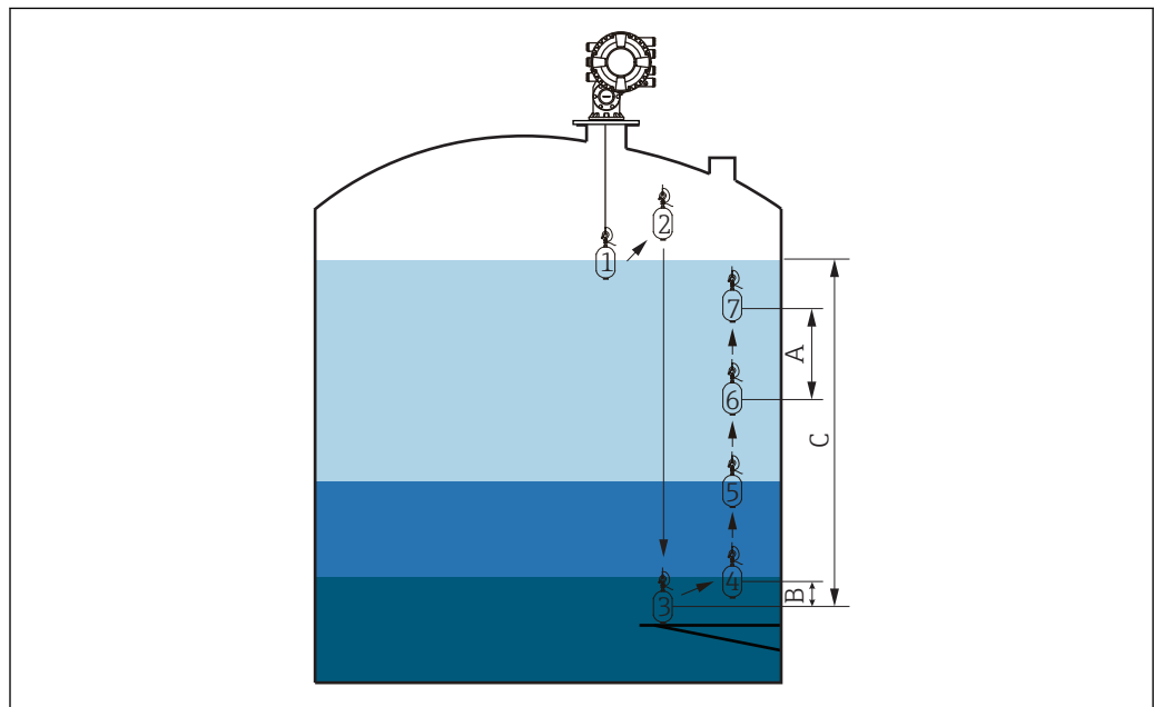
55 Mouvement du profil de cuve (les numéros indiquent l'ordre des mouvements du déplacer.)
