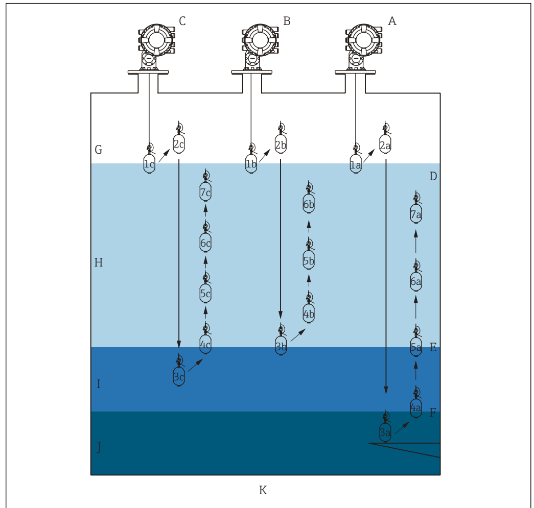
54 Aperçu du profil de densité (1a, 2a, 3a... montrent l'ordre des mouvements du déplacer.)
