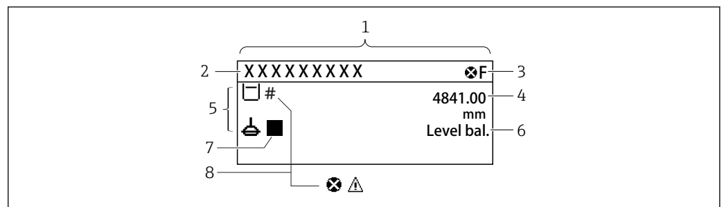
75 Apparence typique de la vue standard (affichage des valeurs mesurées)
