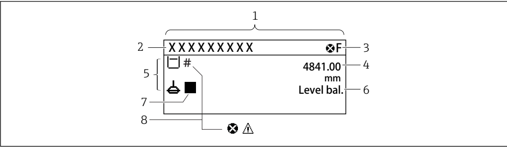
30 Apparence typique de la vue standard (affichage des valeurs mesurées)
