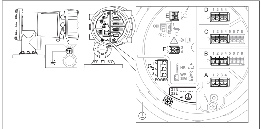
18 Compartiment de raccordement (exemple typique) et bornes de terre
