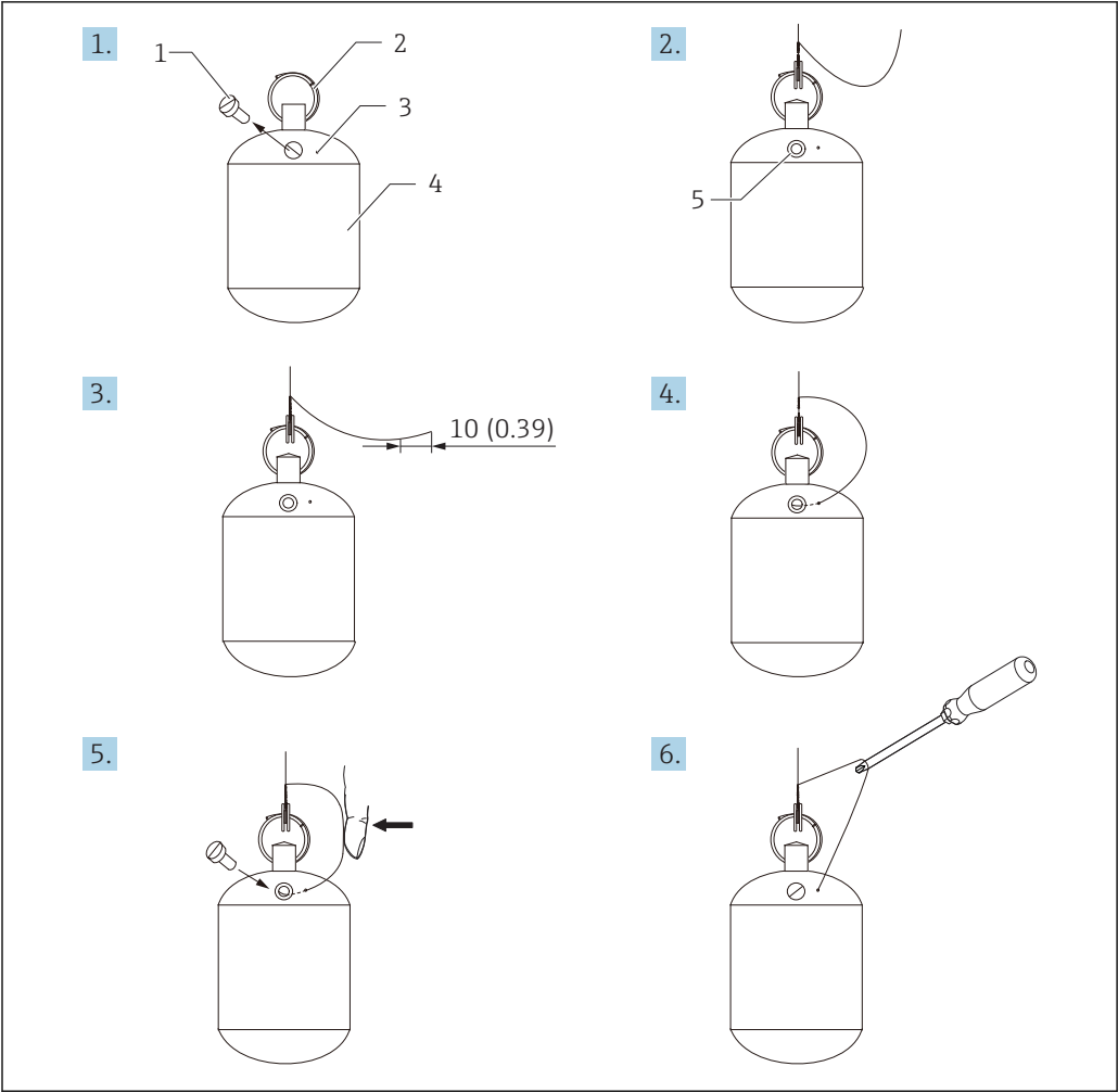
17 Installation du displacer PTFE ; dimensions mm (in)
