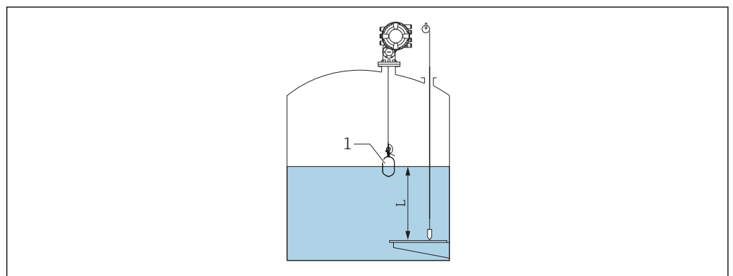
49 Valeur de niveau réglée pour une cuve ouverte
