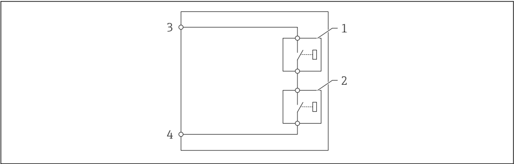
87 Les deux relais d'une sortie numérique 1/2 Les relais 3/4 Les bornes de la sortie numérique
