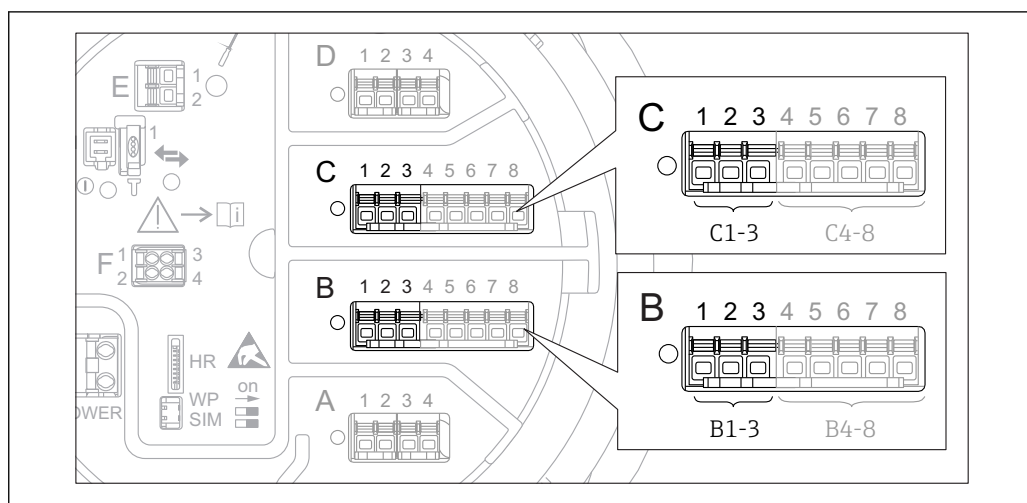
60 Emplacements possibles des modules Analog I/O, pouvant être utilisés comme entrée 4-20 mA. La référence de commande de l'appareil détermine le module réellement présent → 48.
