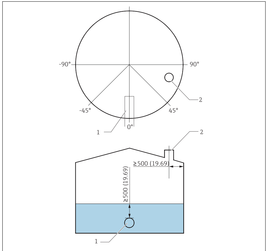
13 Position recommandée pour le montage du NMS8x et le niveau de mesure minimum ; dimensions mm (in)
