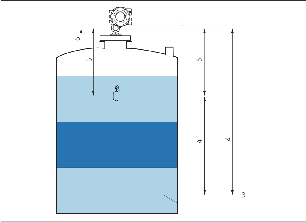
82 Displacer attendant que le niveau du liquide monte lors de la commande de jaugeur Standby level 1 Niveau de référence 2 Empty 3 Plaque de niveau de référence 4 Standby level 5 Standby distance 6 Position de référence
