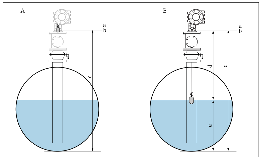
52 Réglage du niveau dans le cas de "Empty" (NMS80/81)
