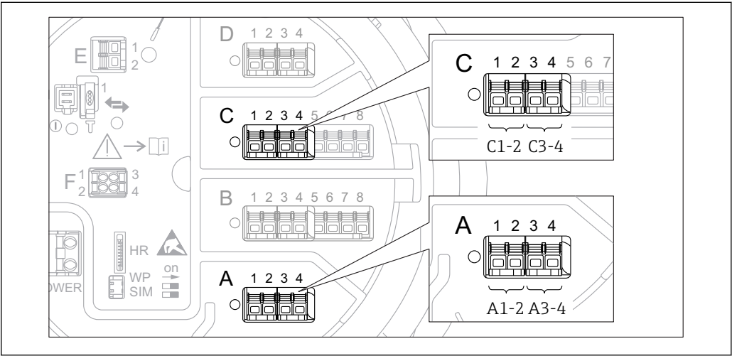
85 Désignation des entrées ou sorties numériques (exemples)
