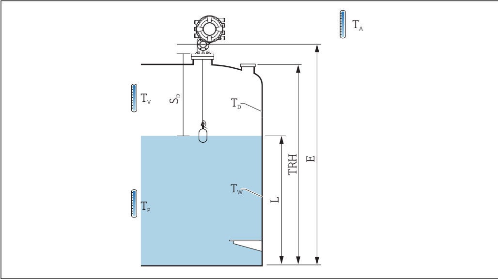
91 Paramètres pour le calcul CTSh
