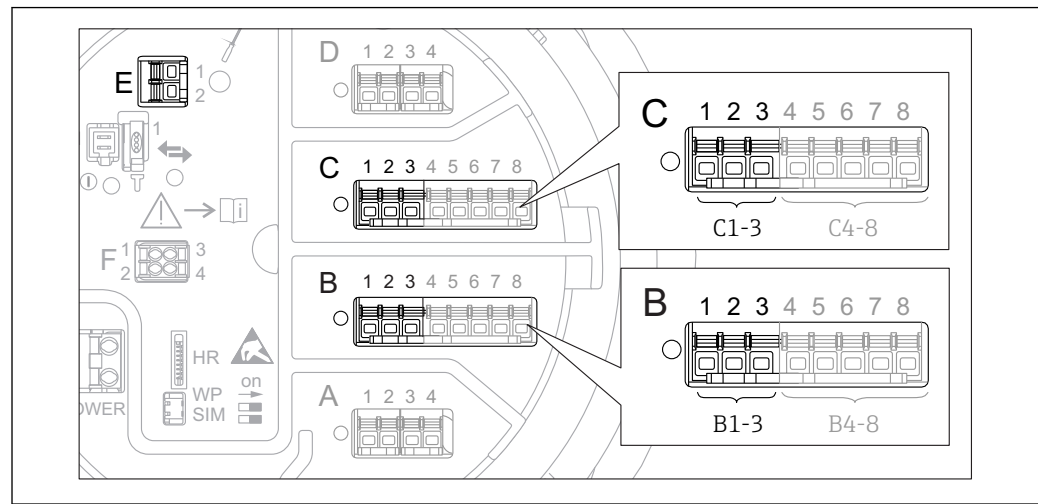
58 Bornes possibles pour les boucles HART
