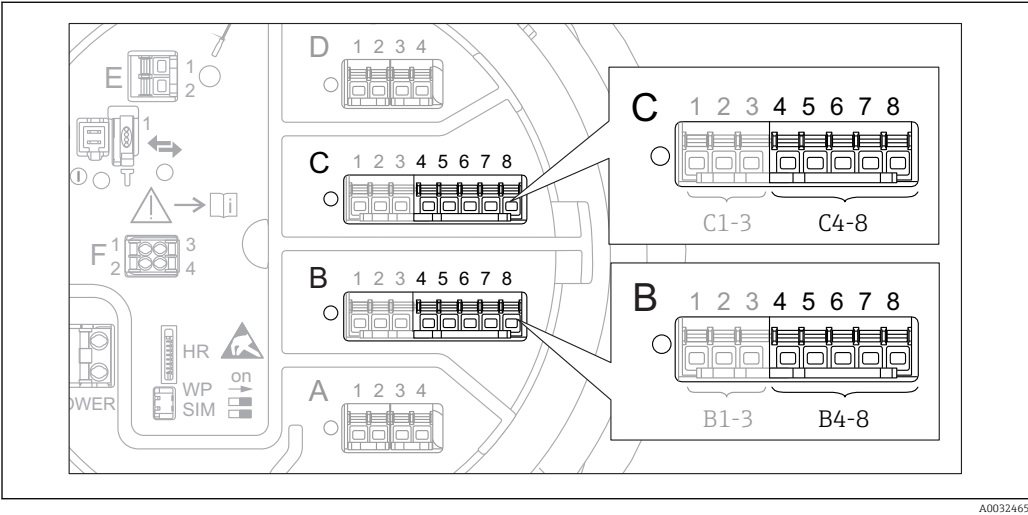
83 Bornes pour le sous-menu "Analog IP" ("B4-8" ou "C4-8", respectivement)
