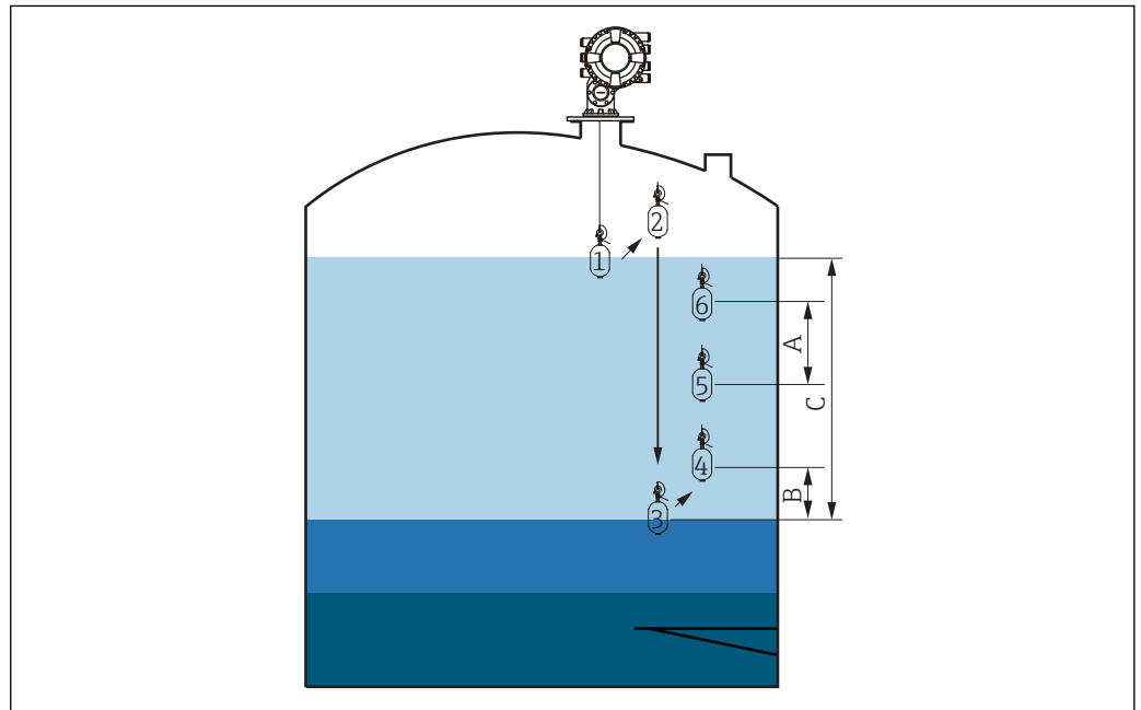
56 Mouvement du profil d'interface (les numéros indiquent l'ordre des mouvements du déplacer.)
