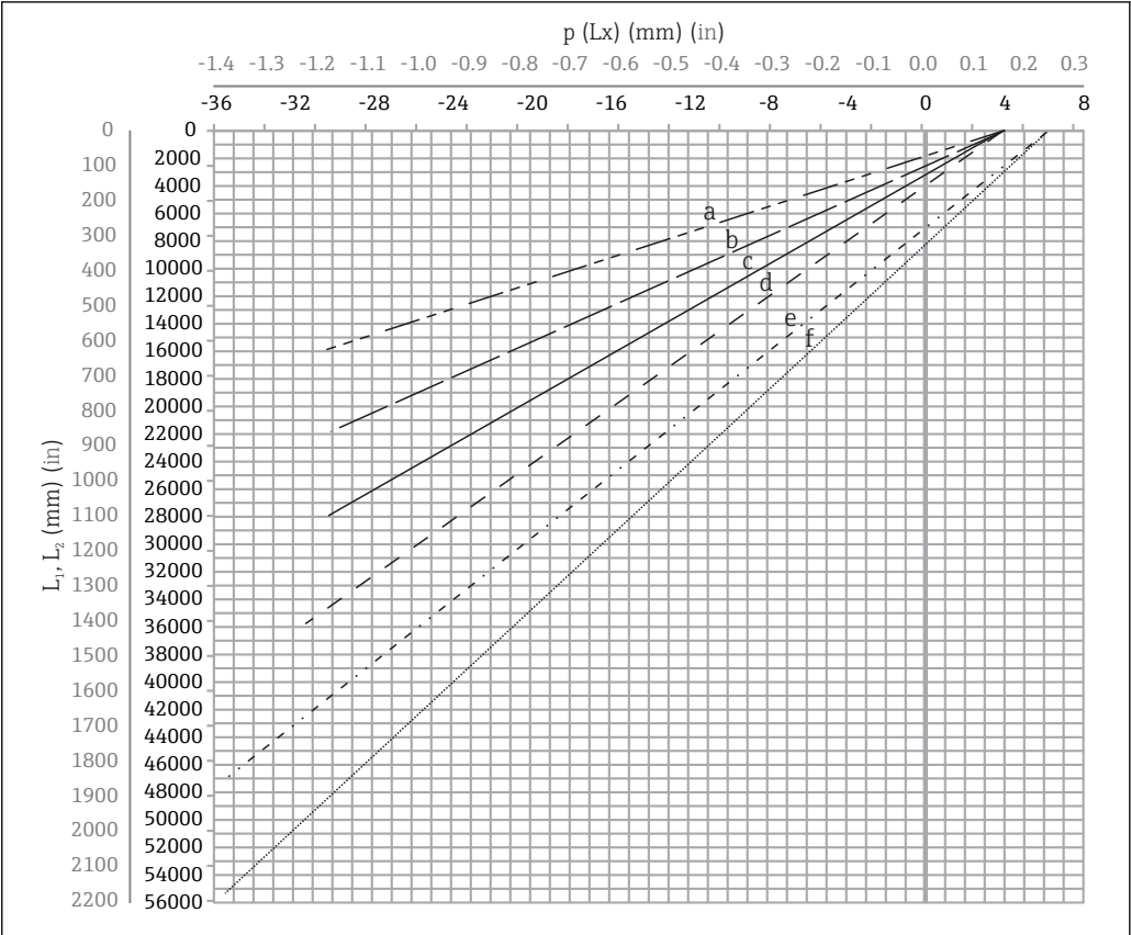
9 Décalage latéral du displacer en fonction de la gamme de mesure
