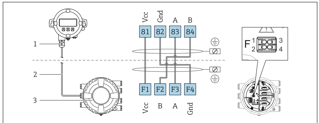
20 Raccordement du module d'affichage et de configuration séparé DKX001 à l'appareil de jaugeage de cuves (NMR8x, NMS8x ou NRF8x)
