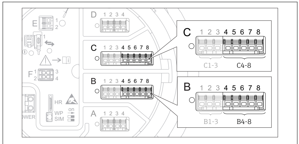
62 Emplacements possibles des modules Analog I/O, auxquels une thermorésistance peut être raccordée. La référence de commande de l'appareil détermine le module réellement présent → 48.
