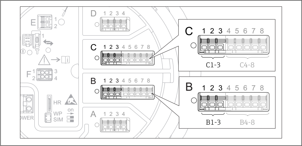
84 Bornes pour le sous-menu "Analog I/O" ("B1-3" ou "C1-3", respectivement)
