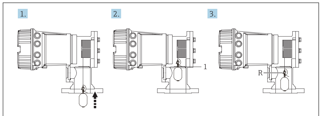
45 Séquence d'étalonnage de référence
