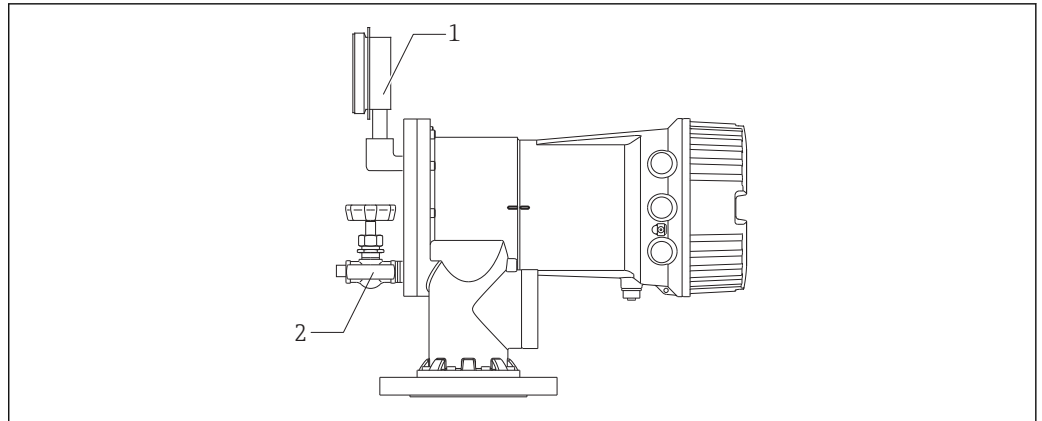
80 Position de montage de la soupape de décharge et du manomètre
