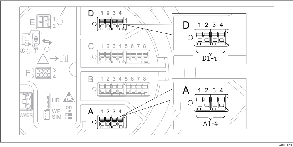
88 Désignation des modules "Modbus", "V1" ou "WM550" (exemples) ; selon la version d'appareil, ces modules peuvent également se trouver dans les slots B ou C.
