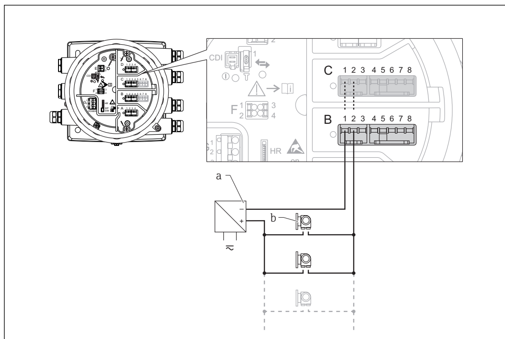
24 Utilisation passive du module Analog I/O en mode maître HART
