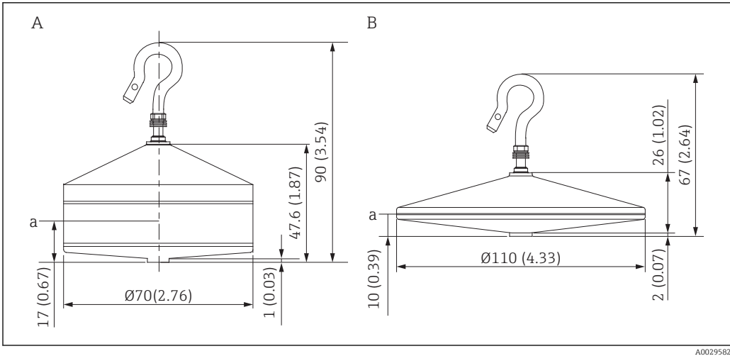
A Displacer conique Ø70 mm (2,76 in), 316L B Displacer conique Ø110 mm (4,33 in), 316L a Point d'immersion
