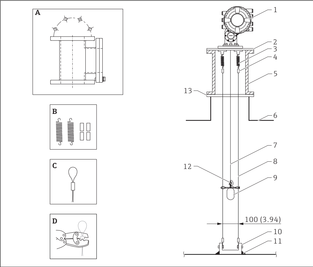
10 Fil guide ; dimensions mm (in)
