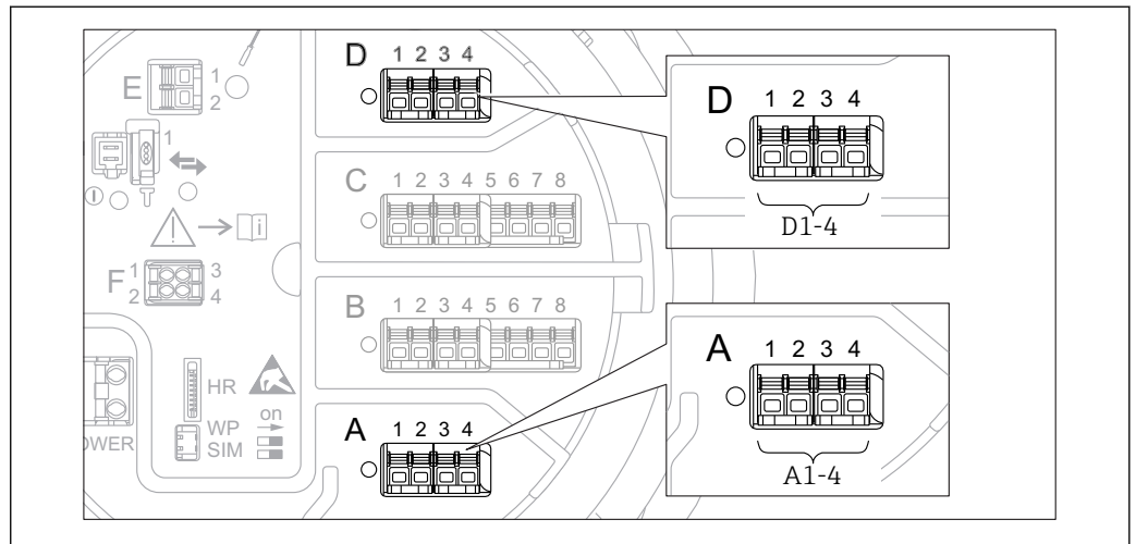
21 Désignation des modules "Modbus", "V1" ou "WM550" (exemples) ; selon la version d'appareil, ces modules peuvent également se trouver dans les slots B ou C.
