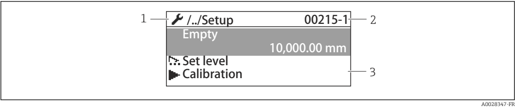
31 Vue navigation 1 Sous-menu ou assistant actuel 2 Code d'accès rapide 3 Zone d'affichage pour la navigation
