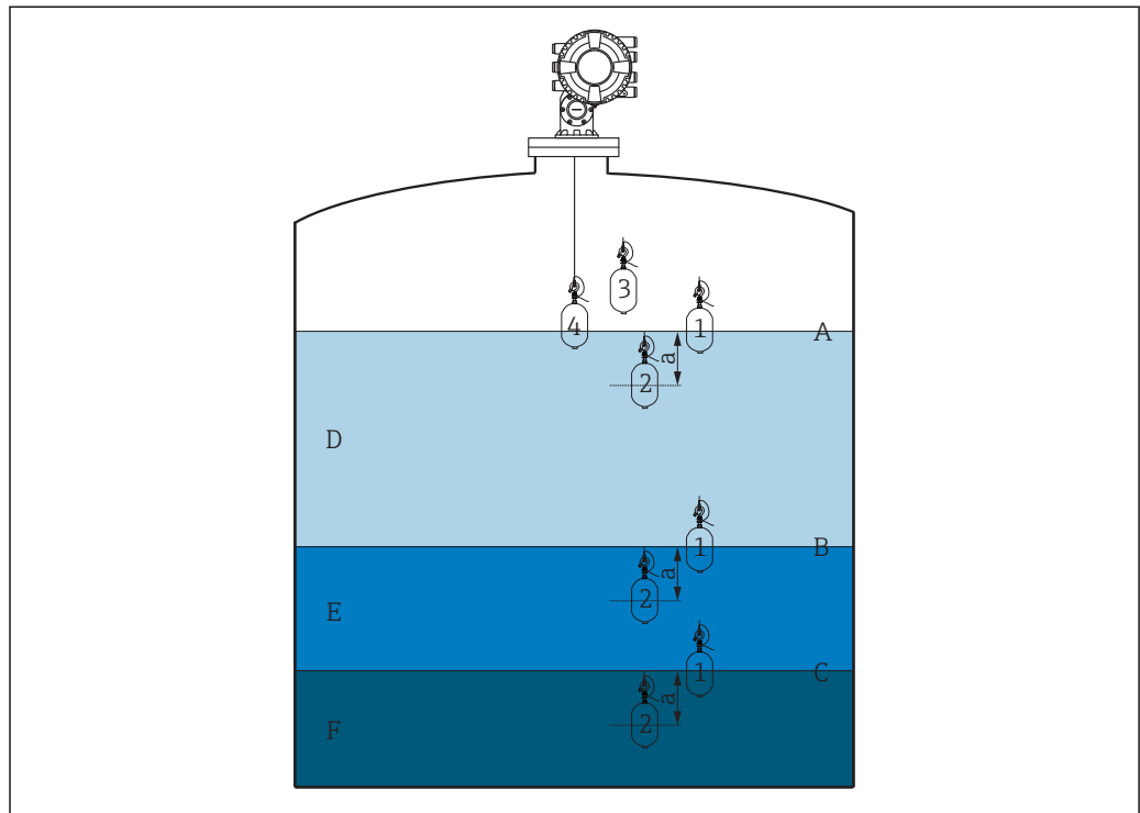
53 Densité instantanée (les numéros indiquent l'ordre du mouvement du déplacer.)
