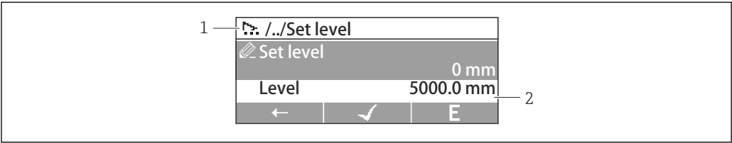
32 Vue assistant du module d'affichage
