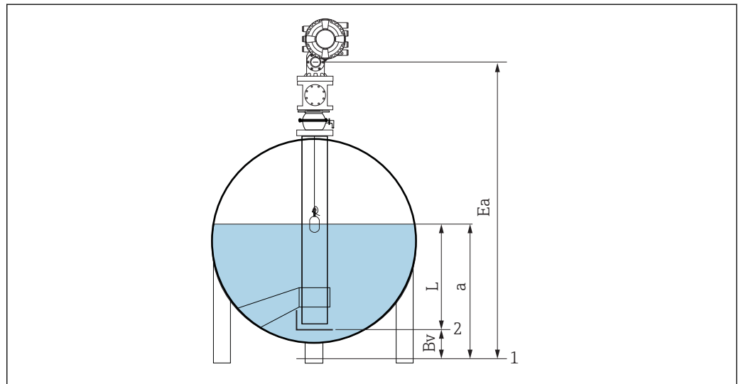
51 Cuve fermée pour NMS80 et NMS81
