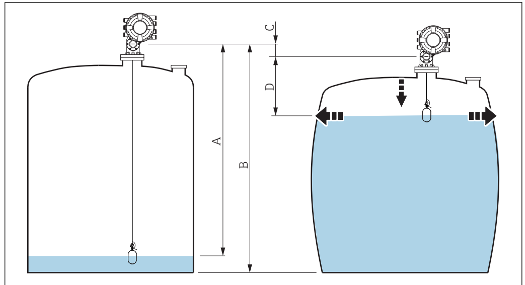
65 Correction de la déformation hydrostatique du réservoir (HyTD)
