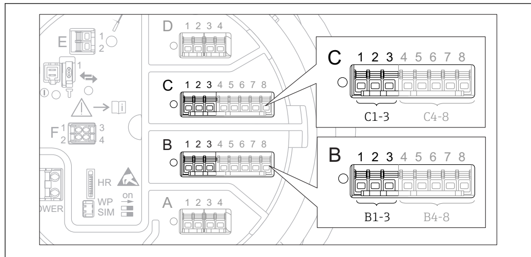
67 Emplacements possibles des modules Analog I/O, pouvant être utilisés comme sortie 4-20 mA. La référence de commande de l'appareil détermine le module réellement présent → 48.
