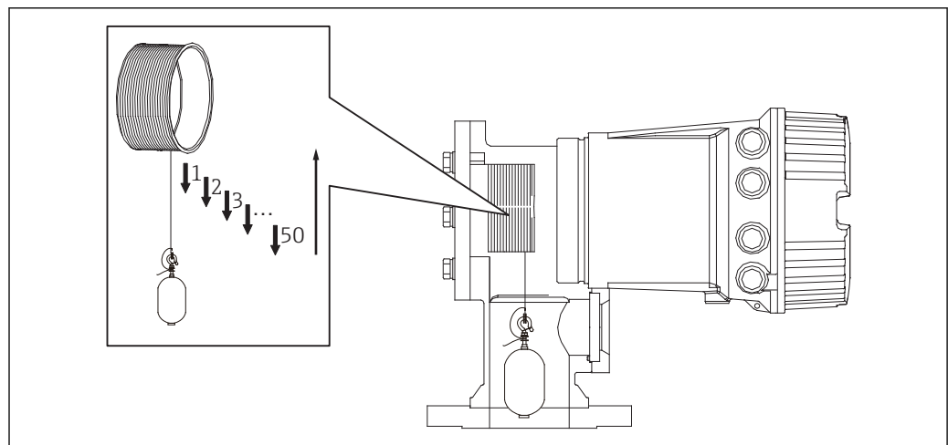
46 Création d'un tableau du tambour
