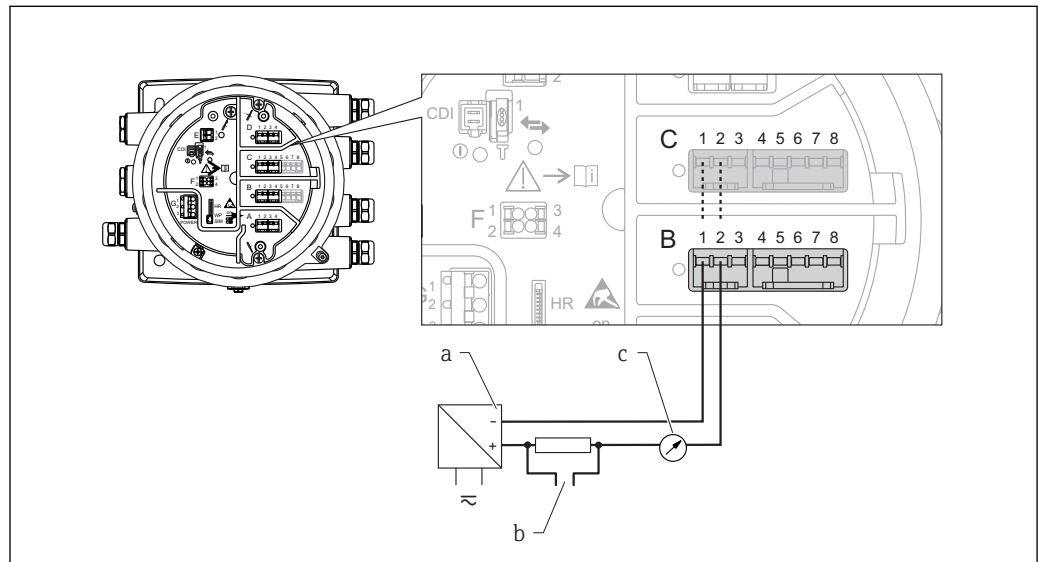
22 Utilisation passive du module Analog I/O en mode sortie
