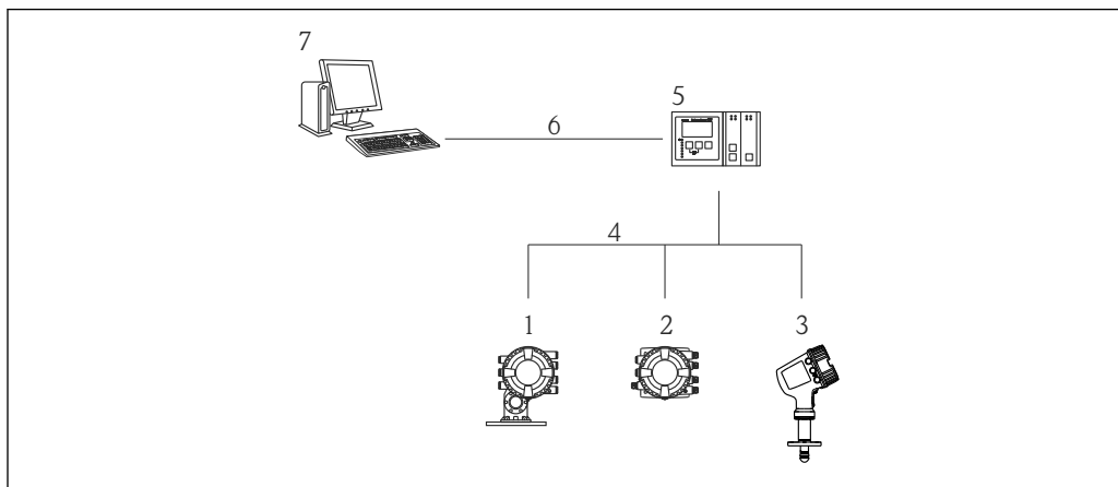
40 Raccordement des appareils de jaugeage de cuves à FieldCare via le Tankvision Tank Scanner NXA820
