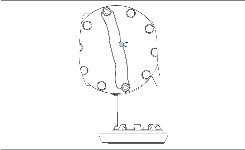
36 Plombage du cache arrière (p. ex. NMS81/NMS83)
