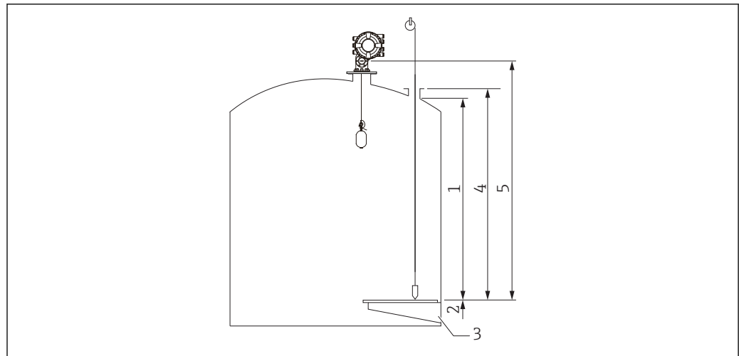
48 Hauteur de la cuve
