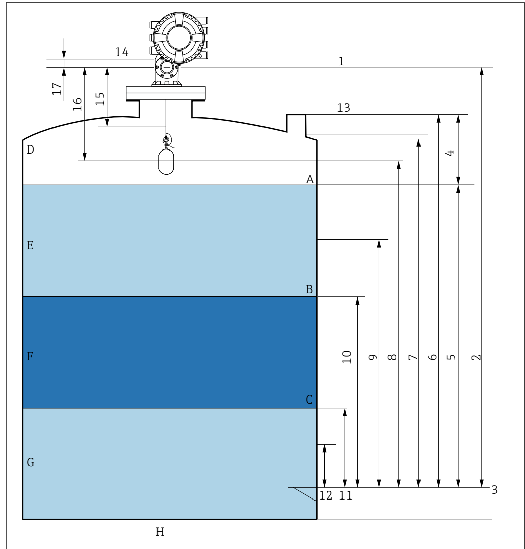
41 Termes relatifs au montage du NMS8x (p. ex. NMS81)
