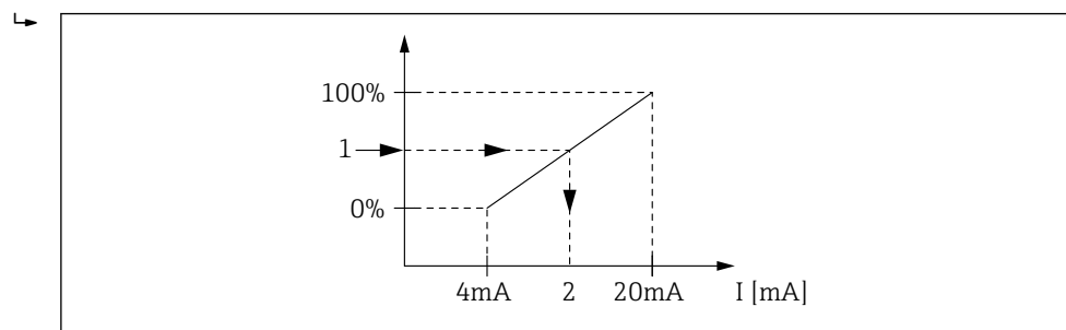
68 Mise à l'échelle de la variable de cuve en fonction du courant de sortie
