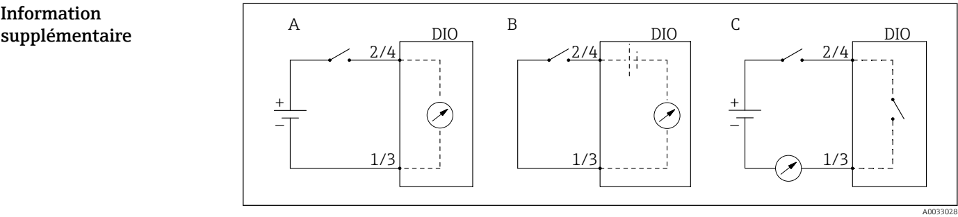
86 Modes de fonctionnement du module Digital I/O
