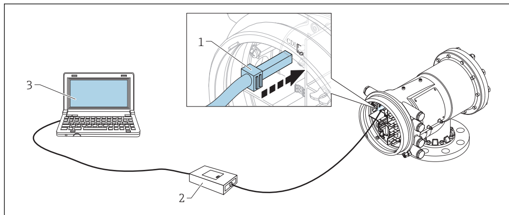
22 Configuration via l'interface service
