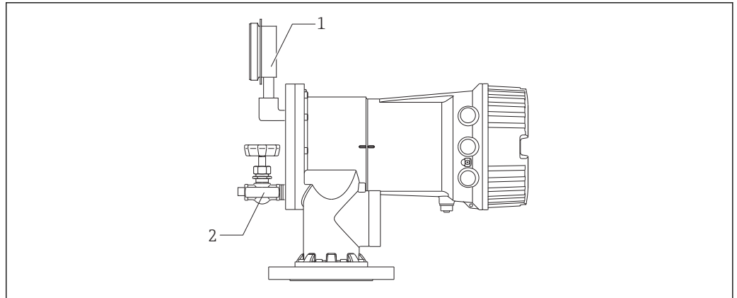
27 Position de montage de la soupape de décharge et du manomètre
