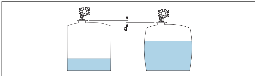
23 Mouvement \Delta x de la hauteur de référence de la cuve dû au gonflement de la paroi du réservoir engendré par la pression hydrostatique
