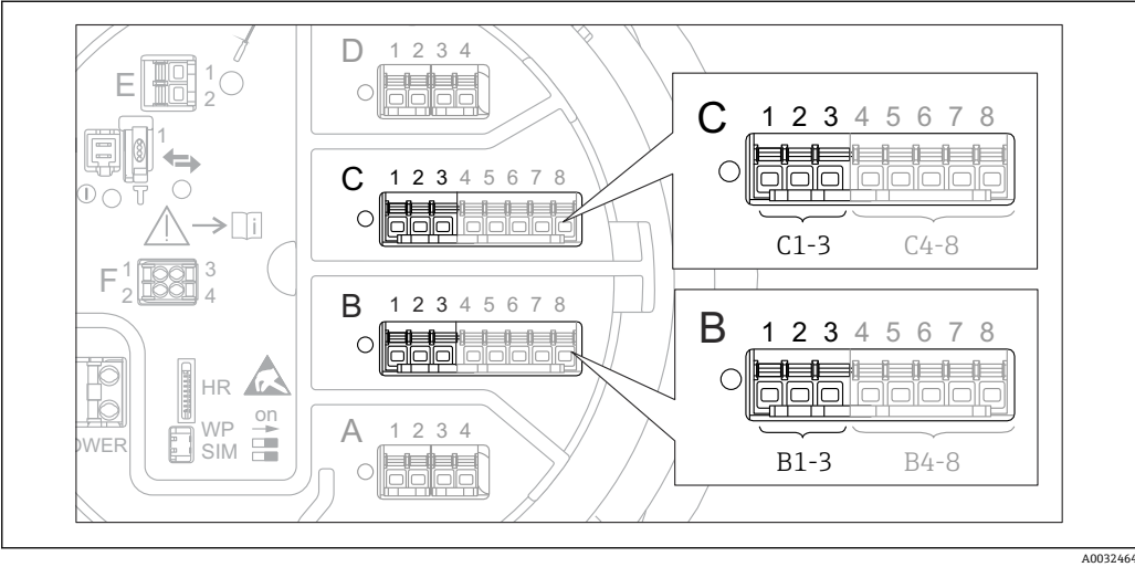
図 49 「Analog I/O」サブメニュー用端子（それぞれ「B1-3」または「C1-3」）
