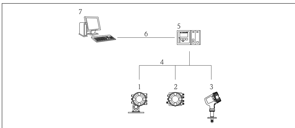
図 26 Tankvision Tank Scanner NXA820 経由でタンクゲージ機器を FieldCare に接続
