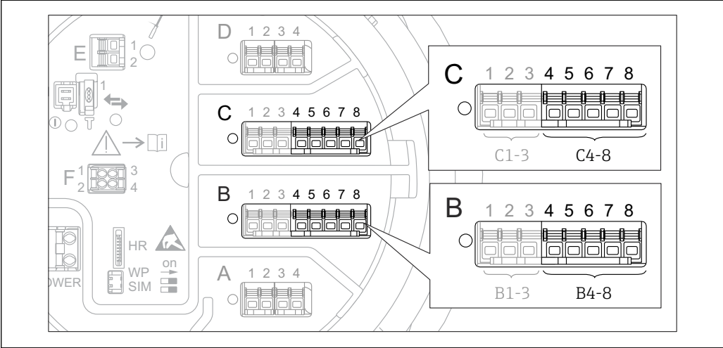
図 48 「Analog IP」 サブメニュー 用端子（それぞれ「B4-8」または「C4-8」）
