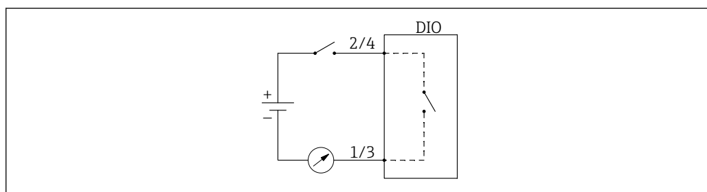
図 45 デジタル出力としてデジタル I/O モジュールの使用法
