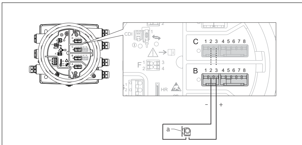
図 14 入力モードのアナログ I/O モジュールのアクティブ使用
