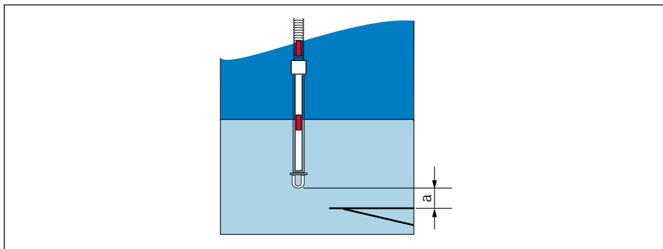
図 29 Prothermo NMT8x : プローブの物理的な終端とゼロレベル値の距離
