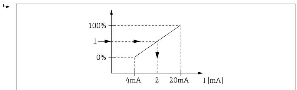
図 39 出力電流へのタンク変数のスケールリング
