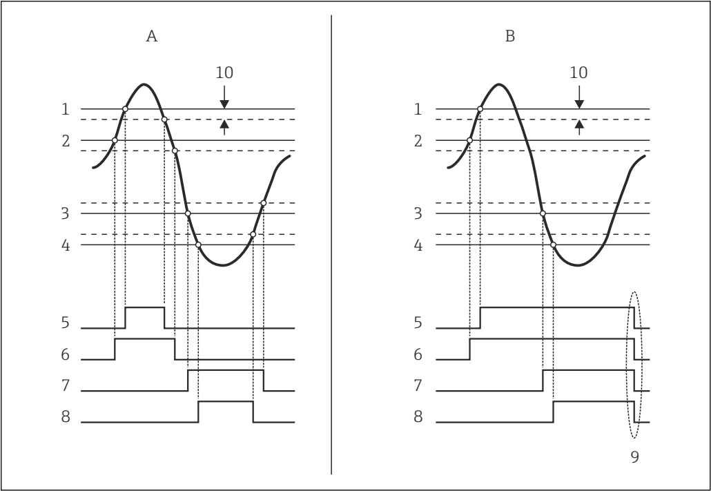
図 61 リミット評価の原理
