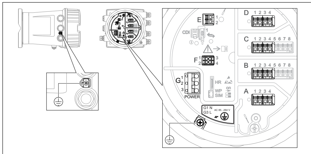
図 6 端子室（標準例）および接地端子
