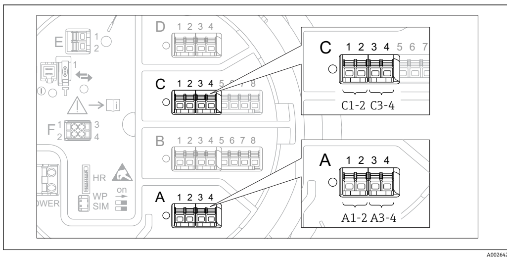
図 17 デジタル入力または出力の名称（例）
