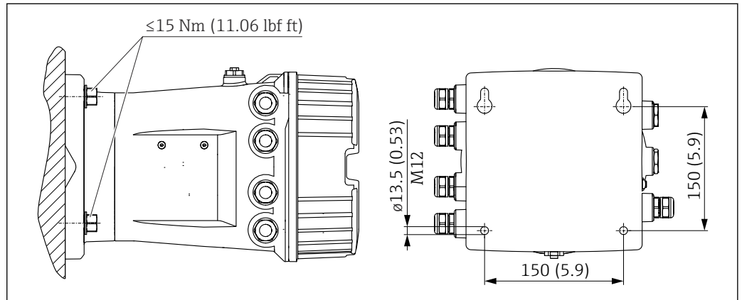
図 3 Tankside Monitor の壁取付け
