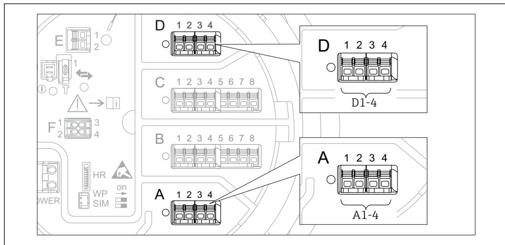
図 41 Modbus モジュールの使用可能な端子 (例)。機器バージョンに応じて、Modbus モジュールがスロット B または C に対応する場合があります → 18。
