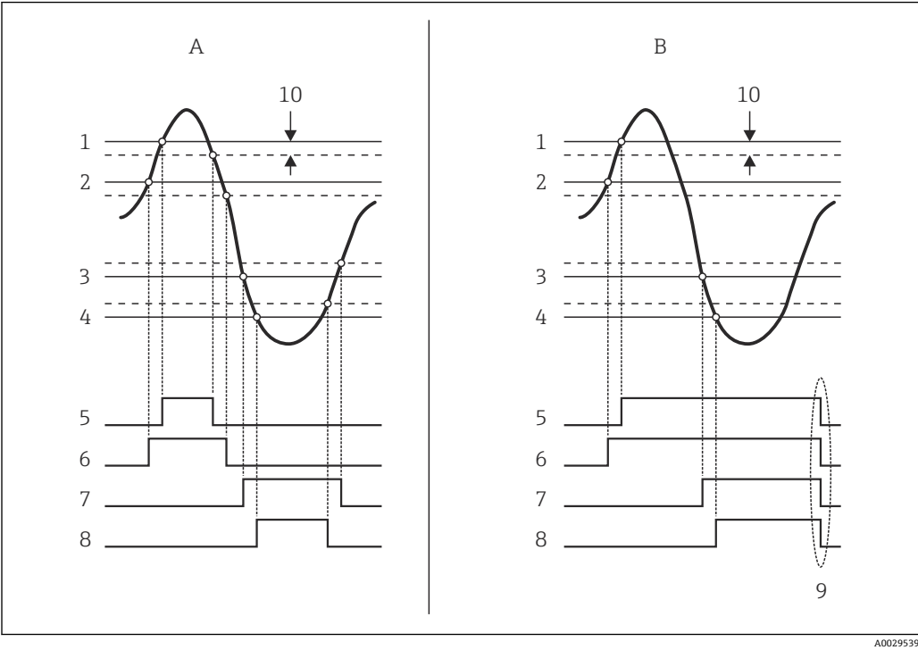
図 37 リミット評価の原理
