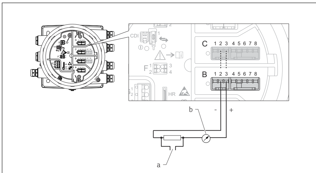
図 13 出力モードのアナログ I/O モジュールのアクティブ使用
