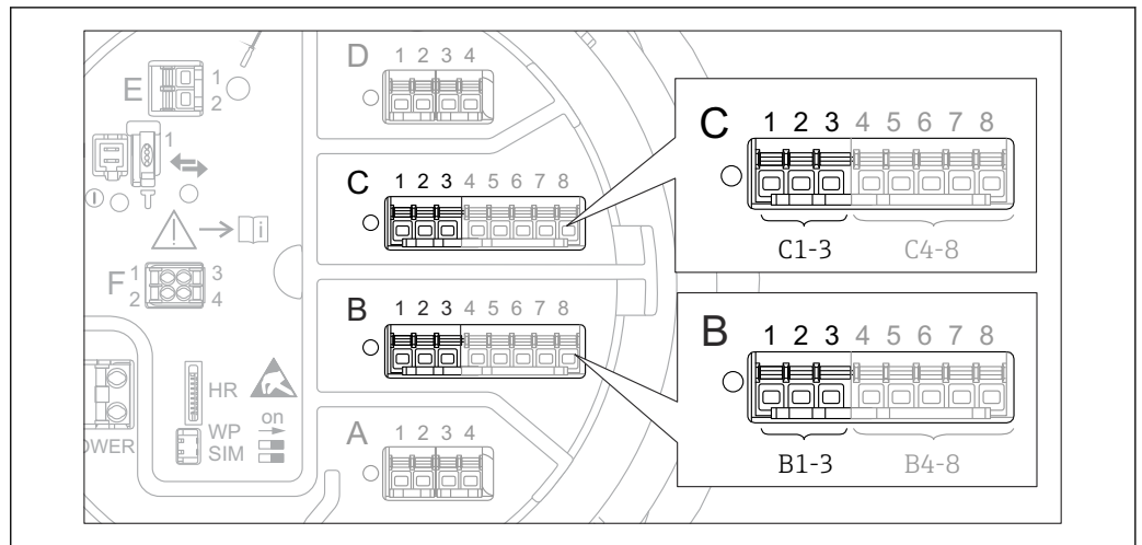
図 38 アナログ I/O モジュールの使用可能な端子。4～20 mA 出力として使用できます。機器のオーダーコードは、実際に存在するモジュールを示します → 図 18。
