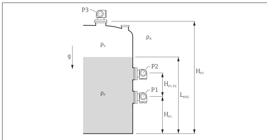
図 57 HTG パラメータ
