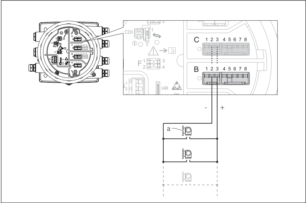
図 15 HART マスタモードのアナログ I/O モジュールのアクティブ使用
