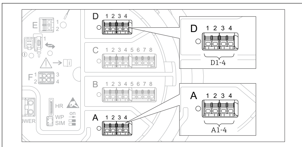
図 43 WM550 モジュールの使用可能な端子 (例)。機器バージョンに応じて、WM550 モジュールがスロット B または C に対応する場合があります→ 図 18。
