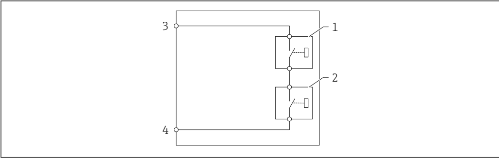
図 52 デジタル出力の 2 つのリレー
