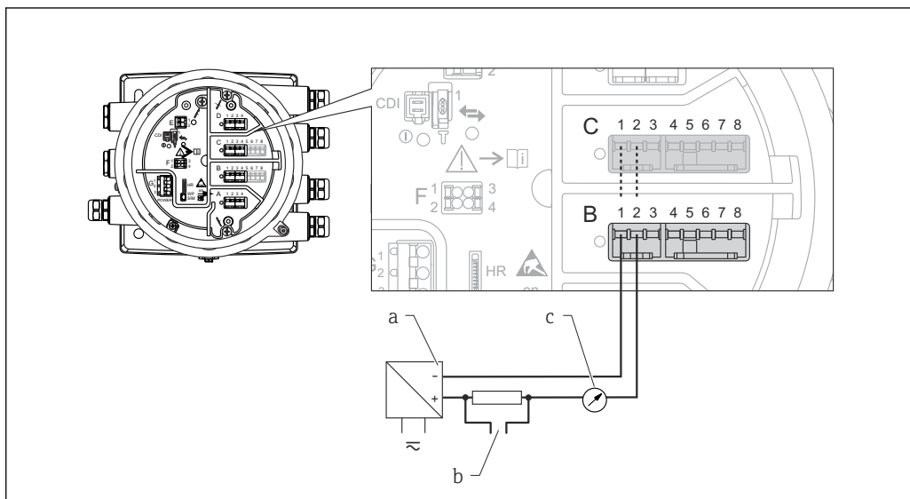
図 10 出力モードのアナログ I/O モジュールのパッシブ使用
