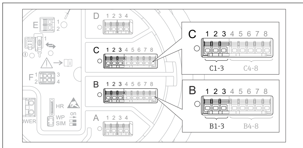
図 30 アナログ I/O モジュールの使用可能な端子。4～20 mA 入力として使用できます。機器のオーダーコードは、実際に存在するモジュールを示します → 図 18。
