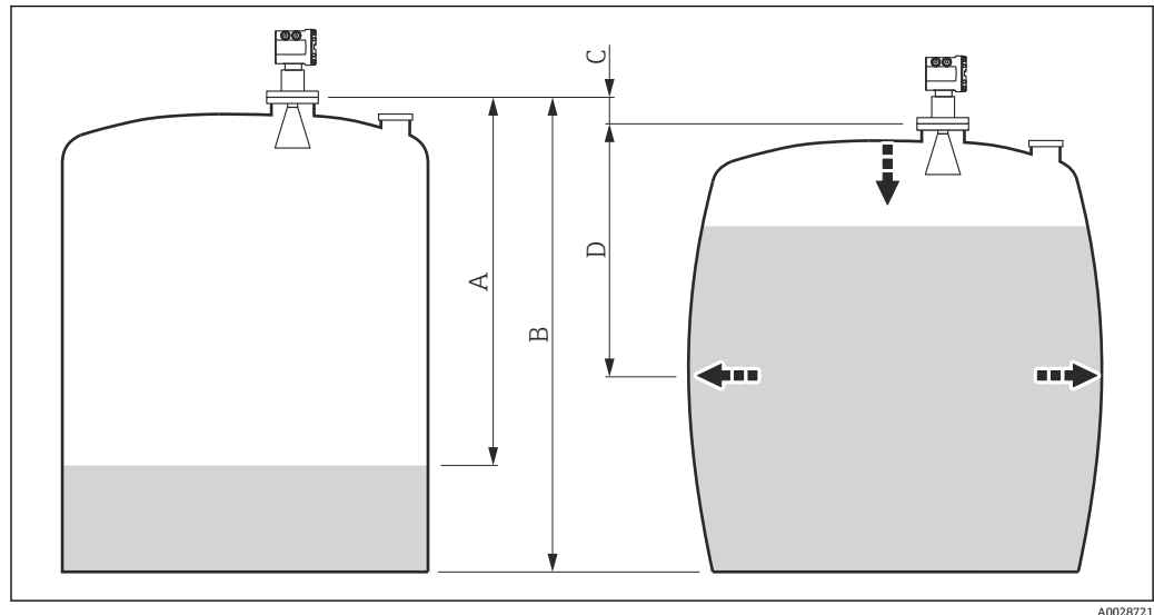
図 36 静圧タンク変形補正（HyTD）
