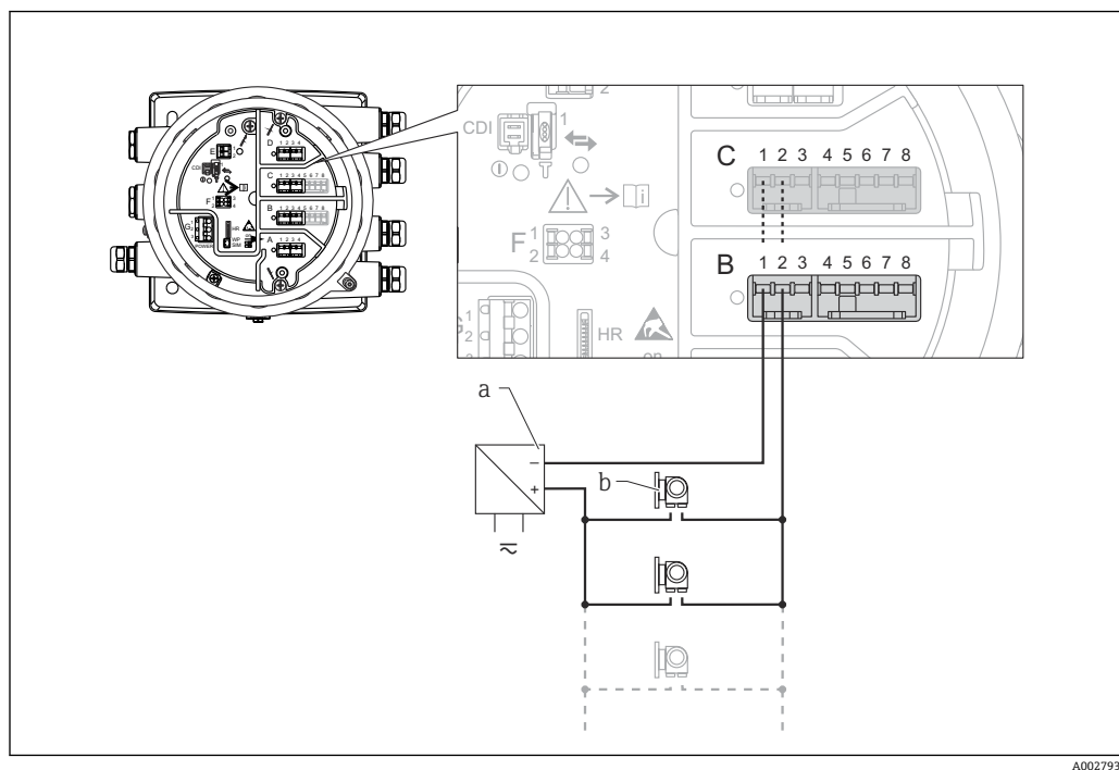
図 12 HART マスタモードのアナログ I/O モジュールのバッシブ使用
