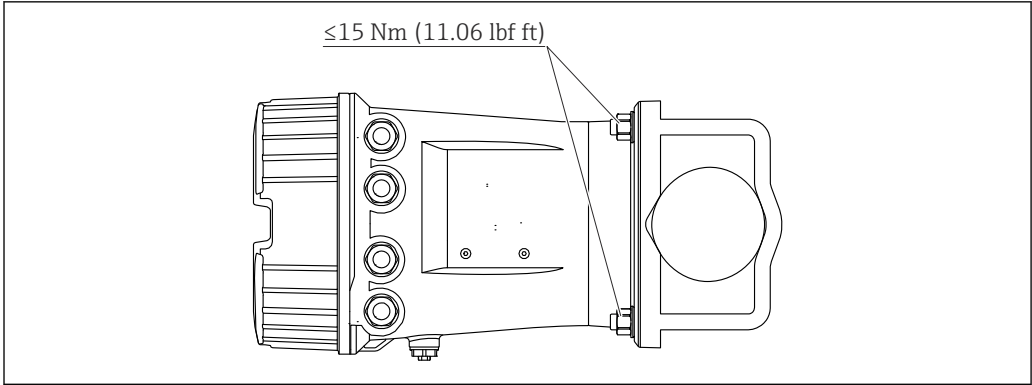
5 Tankside Monitor の水平パイプへの取付け
