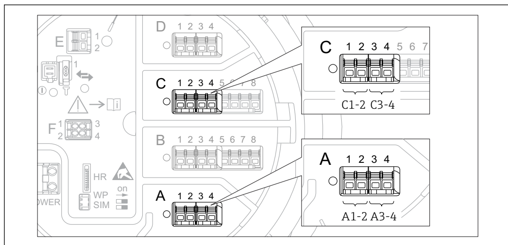
図 44 デジタル I/O モジュールの使用可能な端子（例）。オーダーコードではデジタル I/O モジュールの数と端子を指定します→ 図 18。
