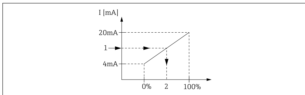
図 31 プロセス変数への 4～20 mA 入力のスケーリング
