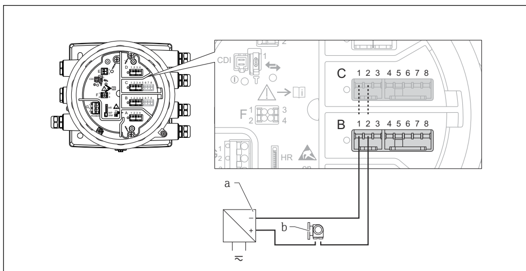
図 11 入力モードのアナログ I/O モジュールのパッシブ使用
