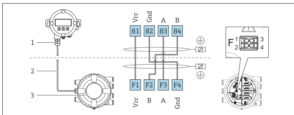
図 8 分離ディスプレイおよび操作モジュール DKX001 とタンクゲージ機器 (NMR8x、NMS8x または NRF8x) の接続
