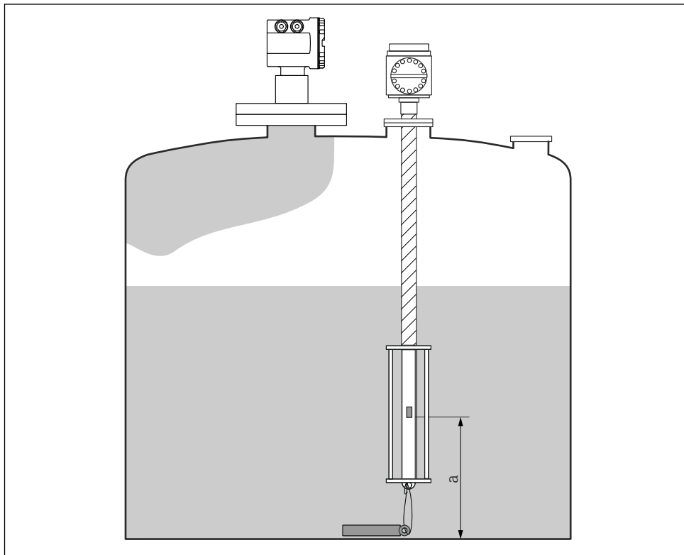
図 28 Prothermo NMT53x : ボトム温度素子の位置
