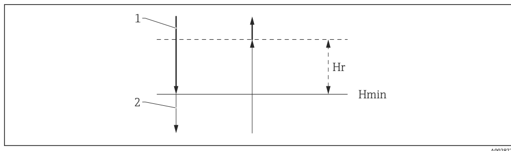
図 58 HTG ヒステリシス
