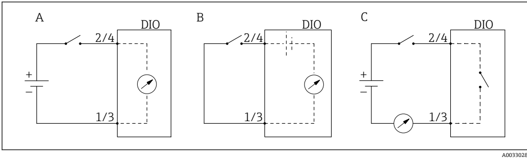
図 51 デジタル I/O モジュールの操作モード
