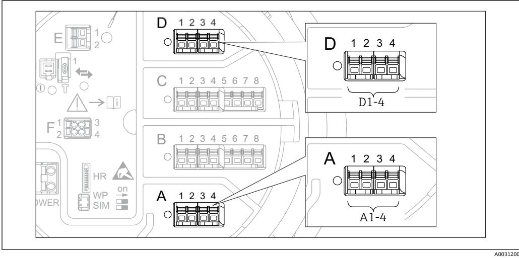
図 53 機器バージョンに応じて、「Modbus」、「V1」、「WM550」モジュール（例）がスロット B または C に対応する場合があります。
