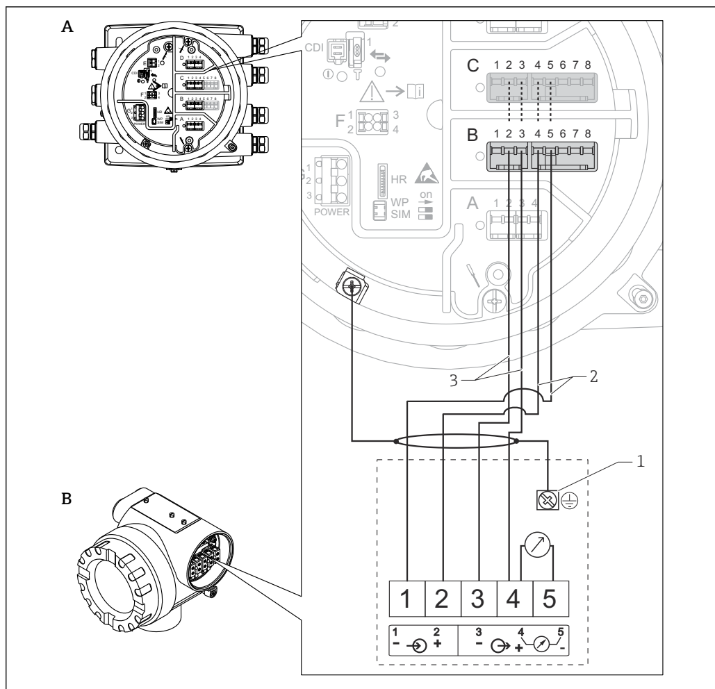
図 16 Tankside Monitor NRF81 のアナログ入力モジュールへの Micropilot S FMR5xx の接続
