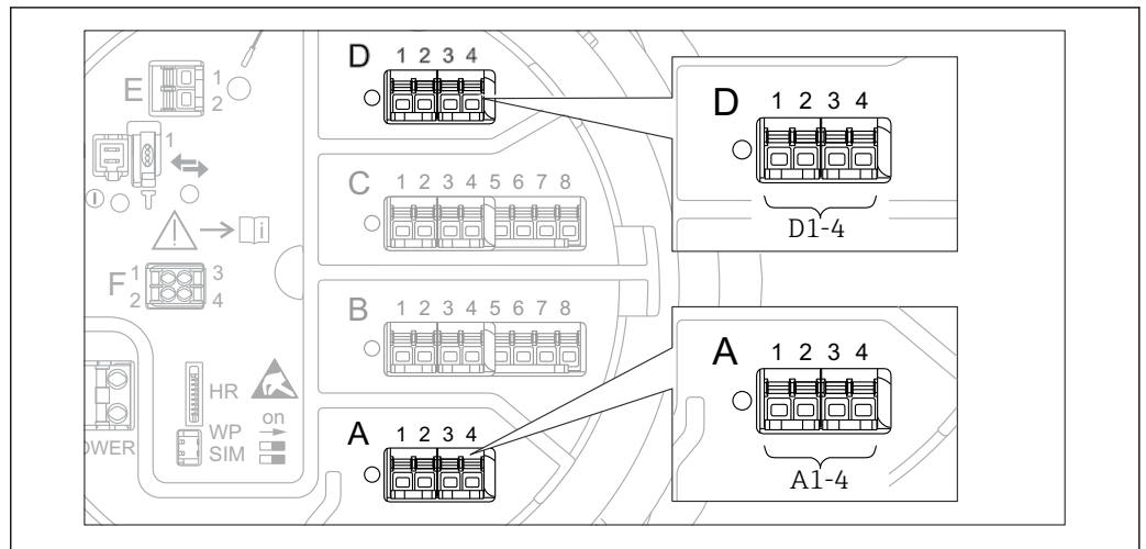
図 9 機器バージョンに応じて、「Modbus」、「V1」、「WM550」モジュール（例）がスロット B または C に対応する場合があります。
