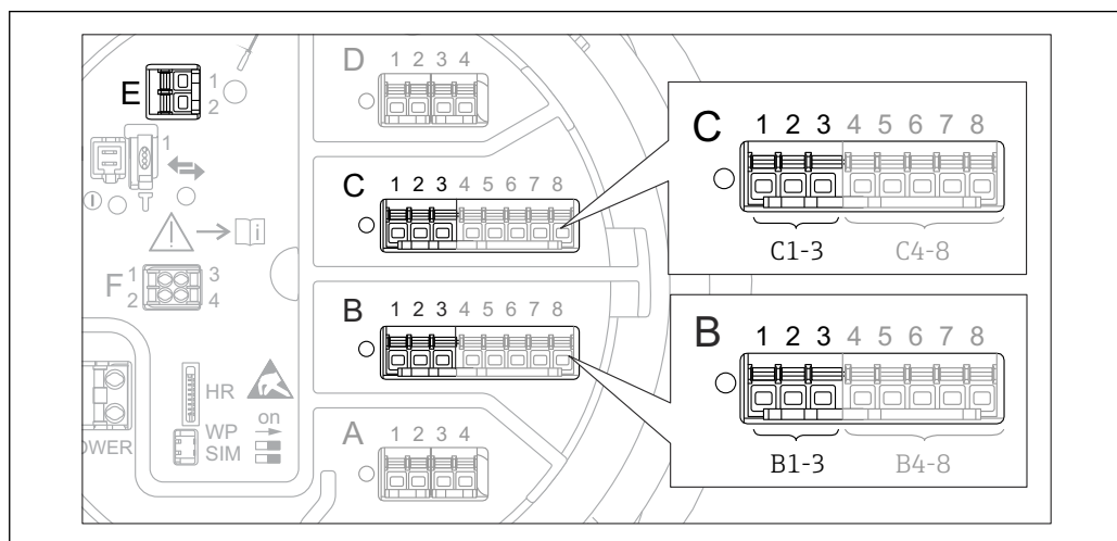
図 27 HART ループに使用可能な端子
