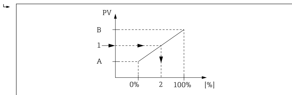
図 40 割合へのタンク変数のスケーリング
