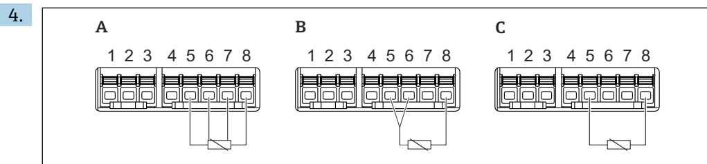
図 33 測温抵抗体の接続タイプ
