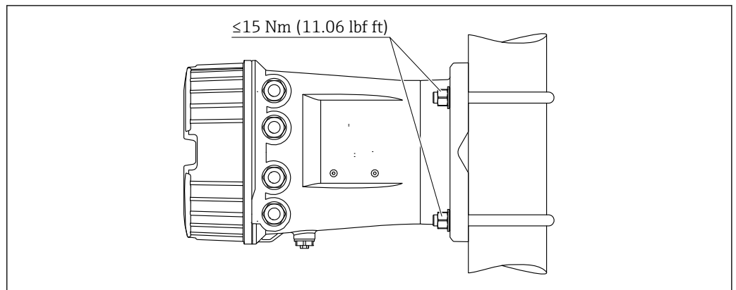
図 4 Tankside Monitor の垂直パイプへの取付け
