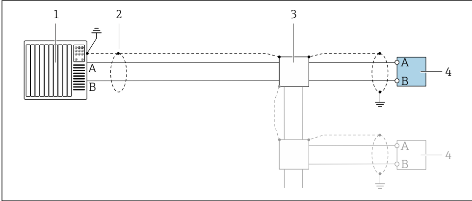
16 Kytkenäesimerkki Modbus RS485, ei-räjähdyksaarallinen tila ja alue 2/Div. 2
