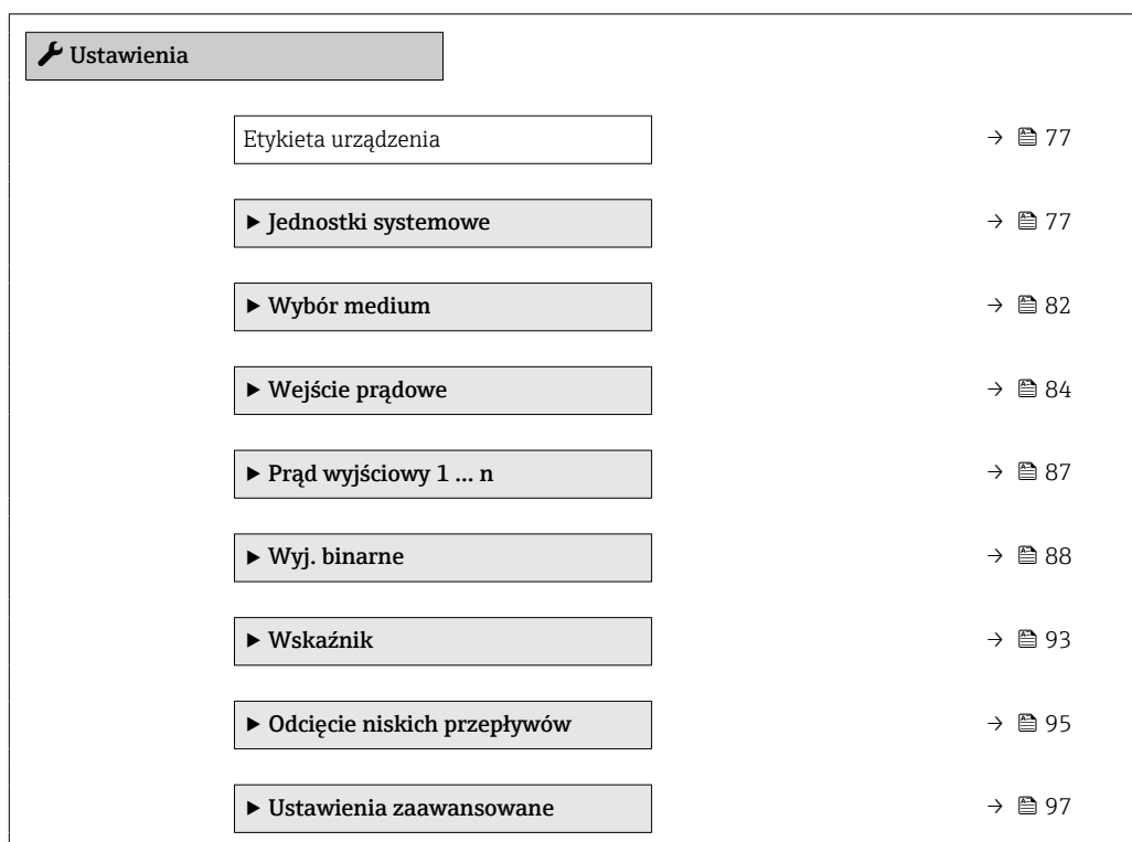
22 Przykład menu na wyświetlaczu lokalnym
