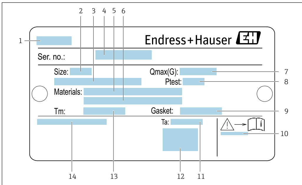
4 Przykładowa tabliczka znamionowa czujnika przepływu
