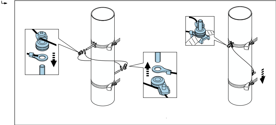
☐ 16 스트랩 밴드 배치(2 ~ 4단계)
