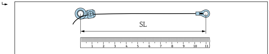
15 와이어 길이(SL)와 일치하는 거리의 픽서 및 케이블 러그
