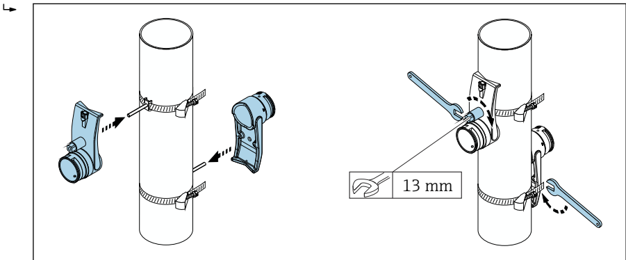
☐ 17 센서 홀더 설치
