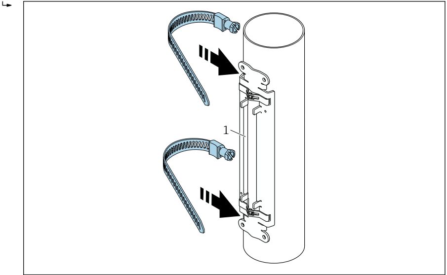
☞ 6 센서 홀더 배치 및 스트랩 밴드 설치
