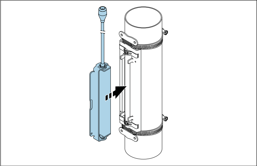
☐ 13 센서 하우징 설치
