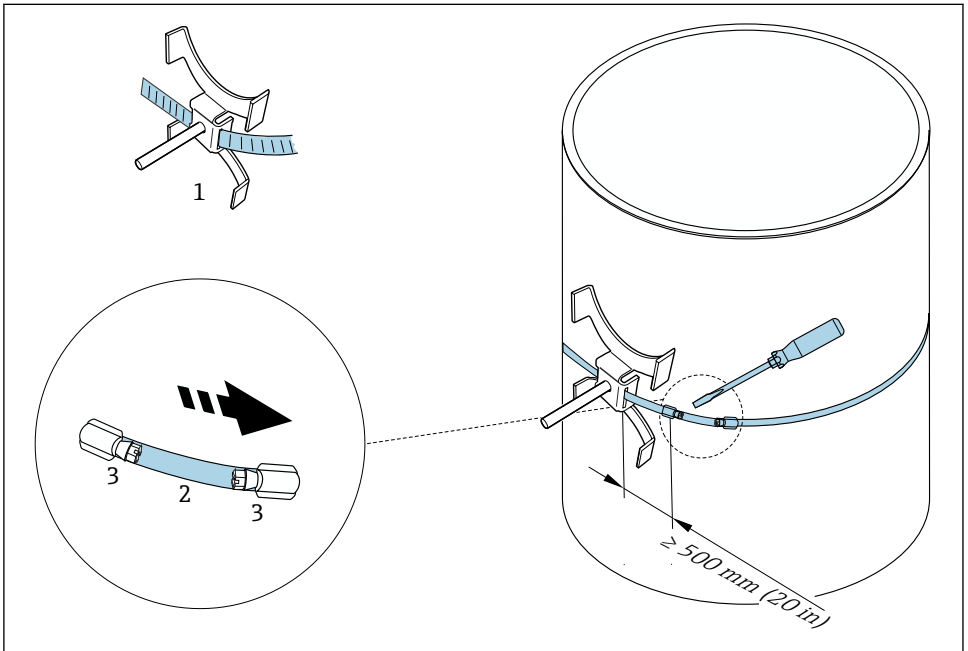
☞ 10 홀더 및 스트랩 밴드(큰 공칭 직경)
