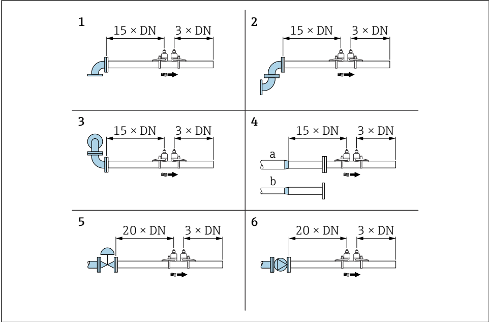
☐ 4 다양한 유량 방해가 발생하는 경우의 최소 전후단 직관부(FlowDC가 없고 센서 세트 1개 또는 2개가 있음)
