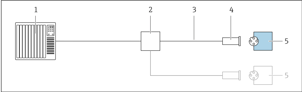
☐ 16 EtherNet/IP의 연결 예
