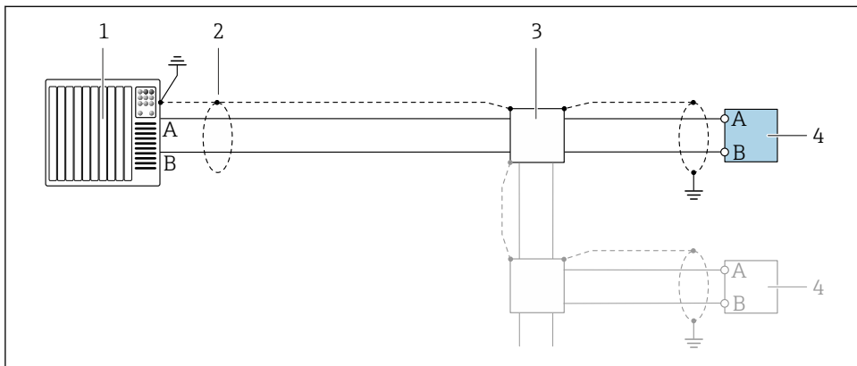
16 Exemplet de conexiune pentru Modbus RS485, zonă care nu prezintă pericol și zona 2/div. 2
