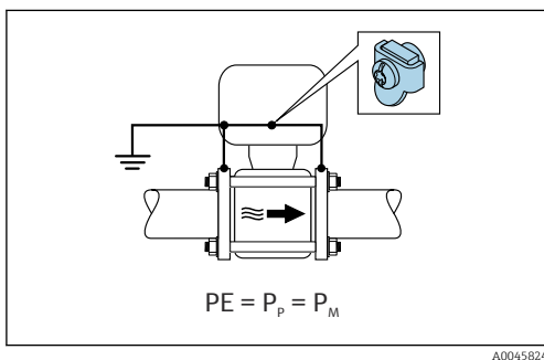
11 Promag D
