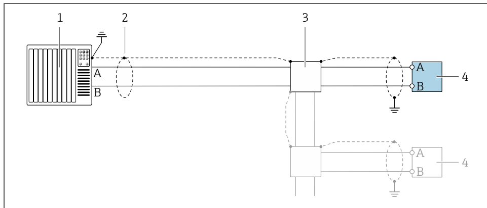
16 Esempio di connessione per Modbus RS485, area sicura e Zona 2/Div. 2
