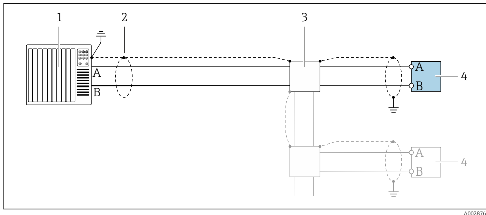
16 Esempio di connessione per PROFIBUS DP, area sicura e Zona 2/Div. 2
