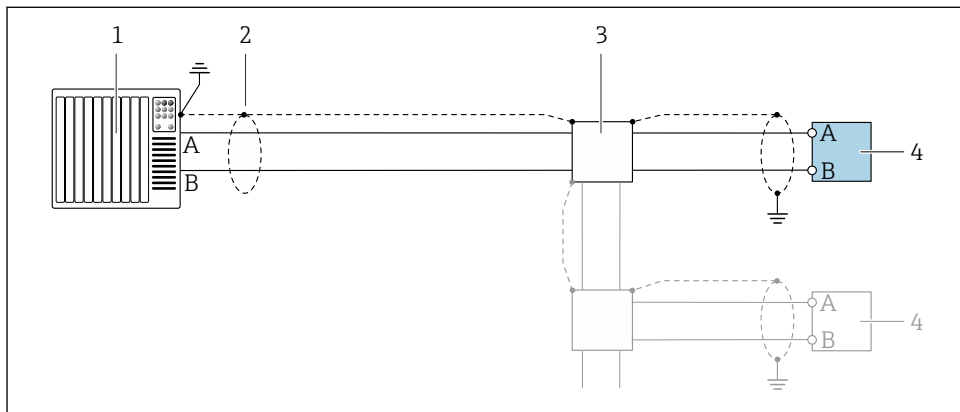
16 Exemplo de conexão para PROFIBUS DP, área não classificada e Zona 2/Div. 2
