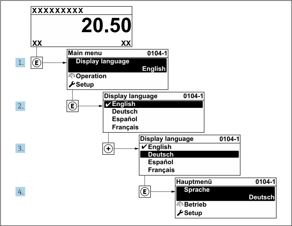
18 Uso do display local como exemplo
