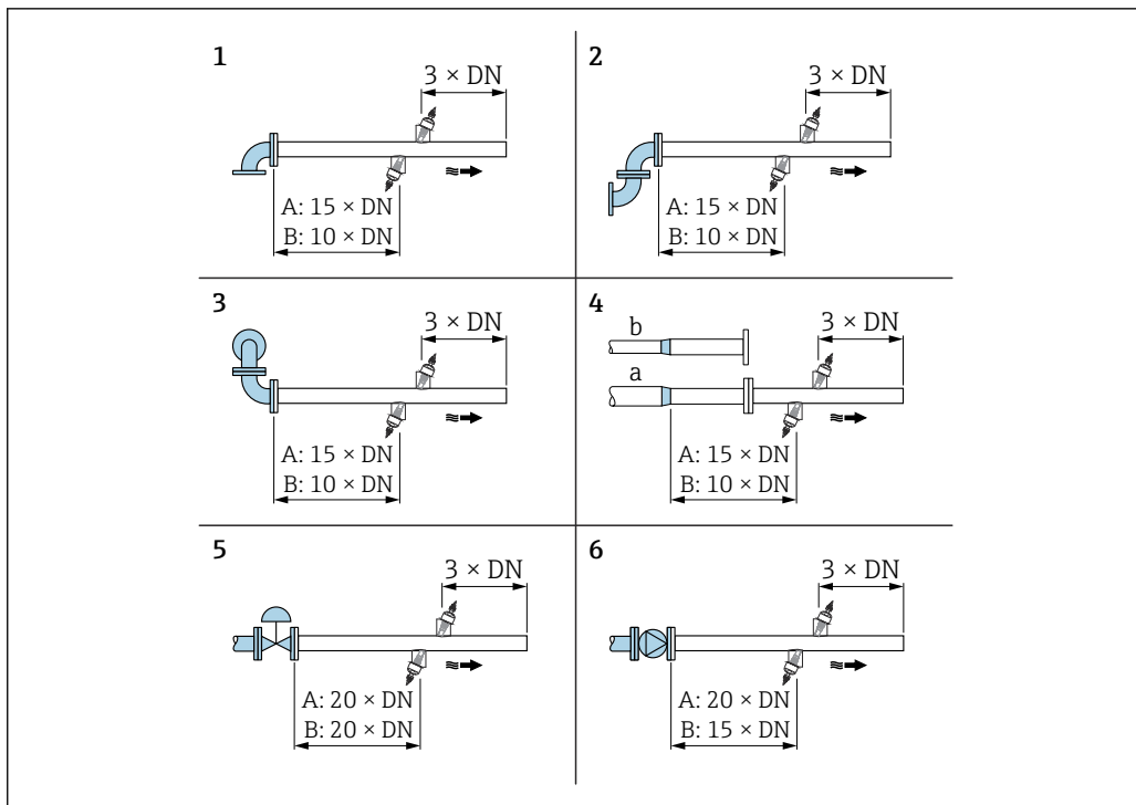
図 6 障害物が存在する場合の上流/下流側の必要直管長 (A : 1 測線計測、B : 2 測線計測) (DN : 配管径)
