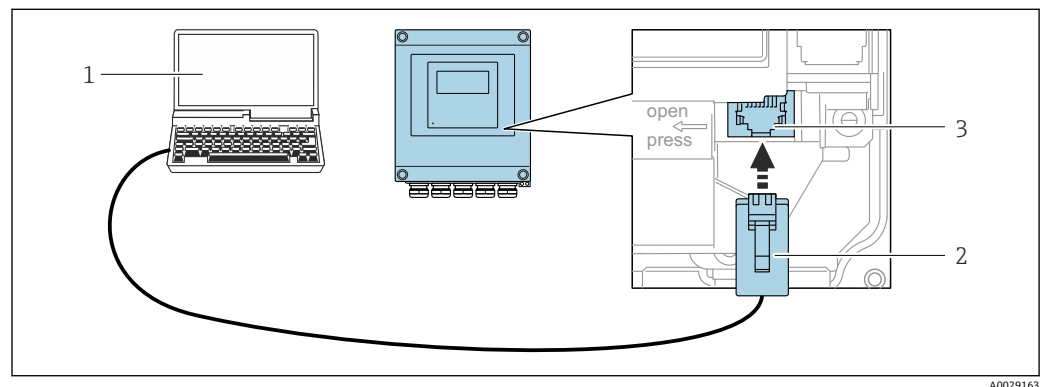
図 20 サービスインターフェイス (CDI-RJ45) 経由の接続
