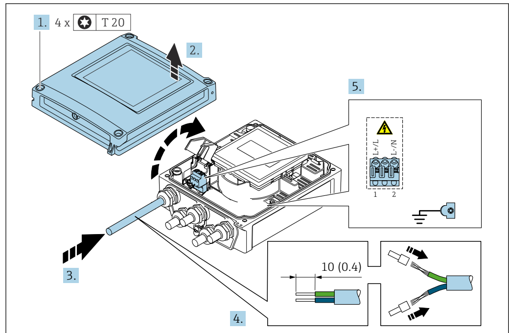
図 12 電源および 0~20 mA/4~20 mA HART の接続、追加の出力/入力付き
