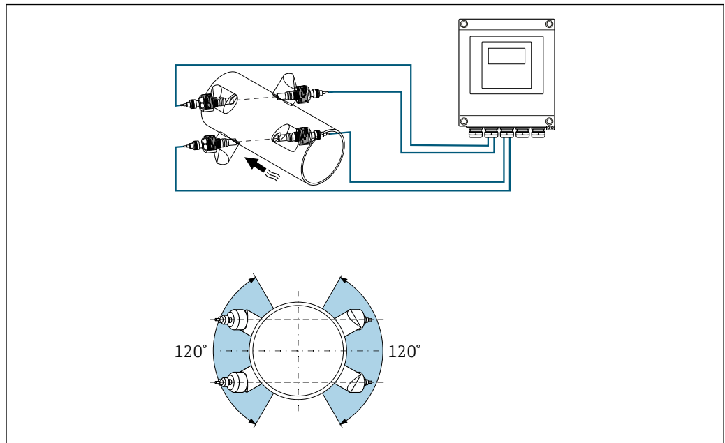
図 7 2 測線計測：測定点におけるセンサセット水平配置の例
