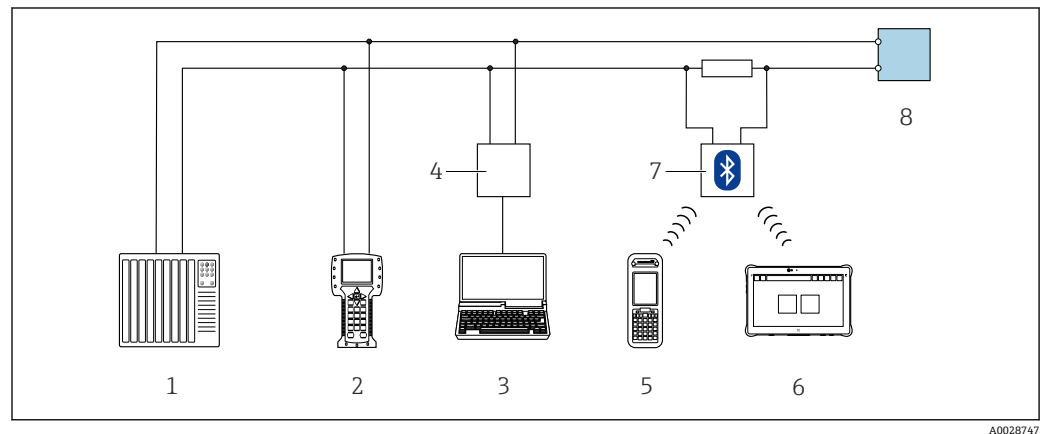
図 19 HART 経由のリモート操作オプション
