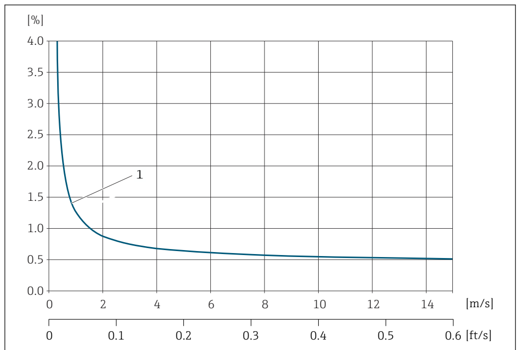
図 30 最大測定誤差の例 (体積流量) (% o.r.)
