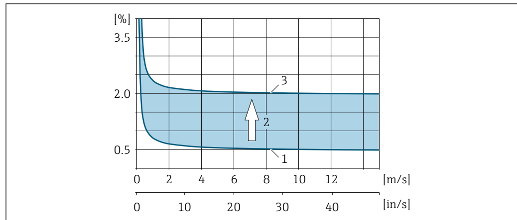
図 29 呼び口径 200A (8") 以上の配管における測定誤差の例
