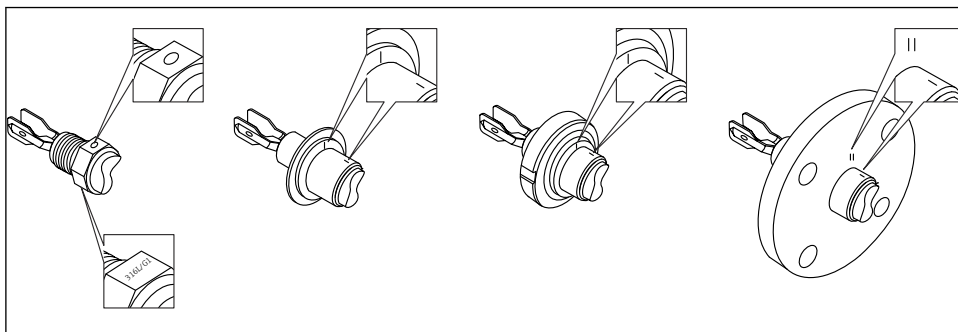
10 Označení pro zarovnání vibrační vidličky
