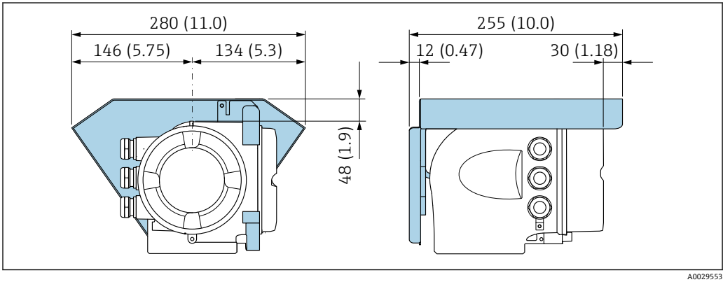
图 44 Proline 500（模拟）的防护罩
