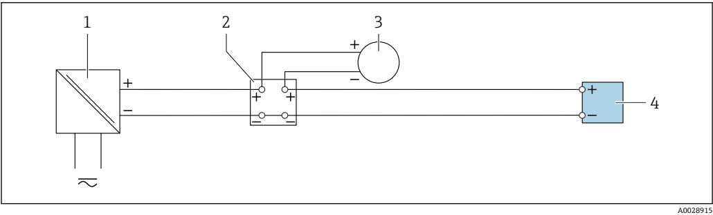
图 18 4...20 mA 电流输入的连接示例
