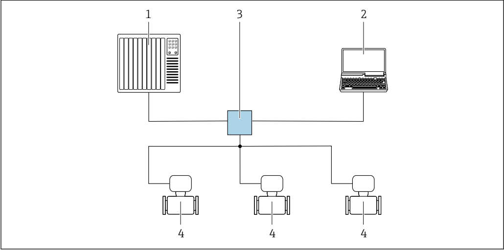
图 58 通过 PROFINET 网络实现远程操作：星形拓扑结构
