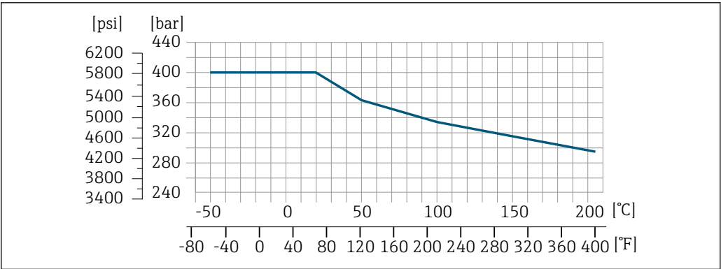
34 4-VCO-4 接头材质: 1.4539 (904L) ; ¼ NPT 螺纹接头材质: 1.4539 (904L) ; ¼"或⅛" SWAGELOK 接头材质: 1.4401 (316)
