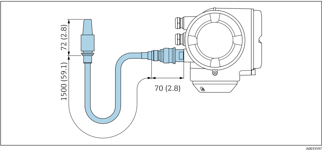
48 单位: mm (in)
