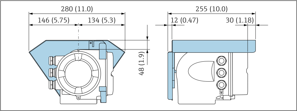
图 27 Proline 500（模拟）的防护罩
