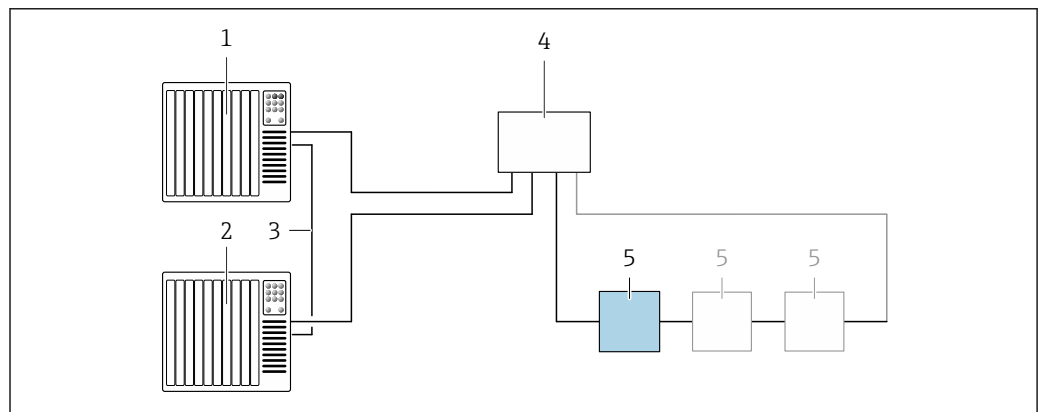
图 8 S2 系统冗余的连接示例
