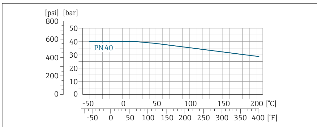
图 29 法兰材质: 1.4539 (904L)、Alloy C22 合金; 松套法兰材质 (不接液): 1.4404 (F316L)
