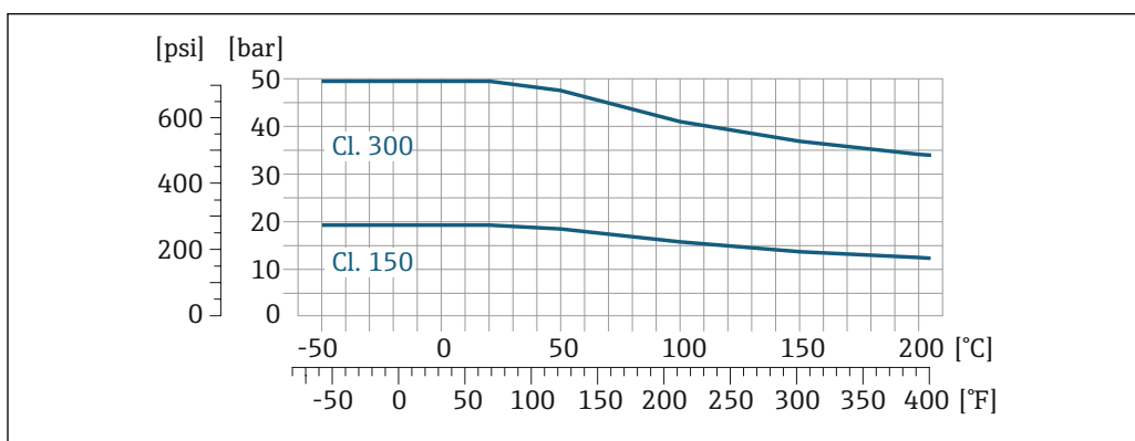
图 30 法兰材质: 1.4539 (904L)、Alloy C22 合金; 松套法兰材质 (不接液): 1.4404 (F316L)
