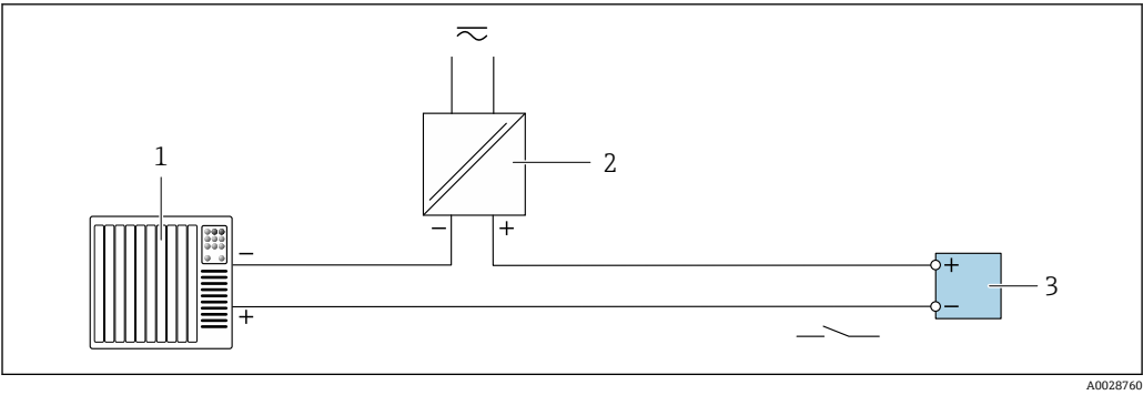
图 17 继电器输出的连接实例(无源)
