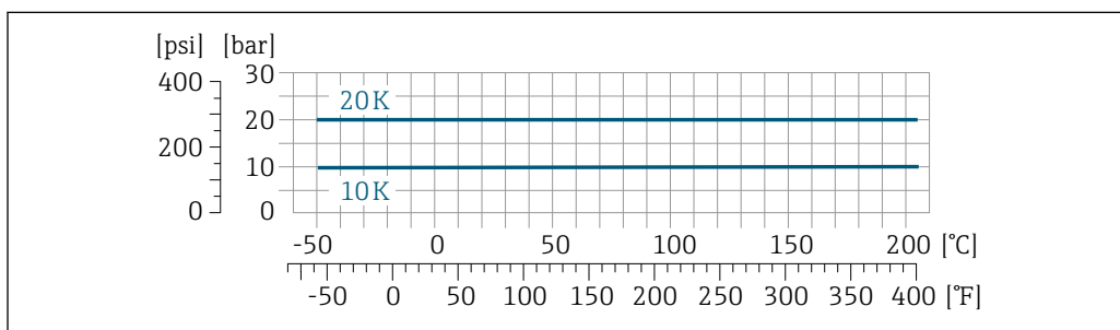
图 31 法兰材质: 1.4539 (904L)、Alloy C22 合金; 松套法兰材质 (不接液): 1.4404 (F316L)
