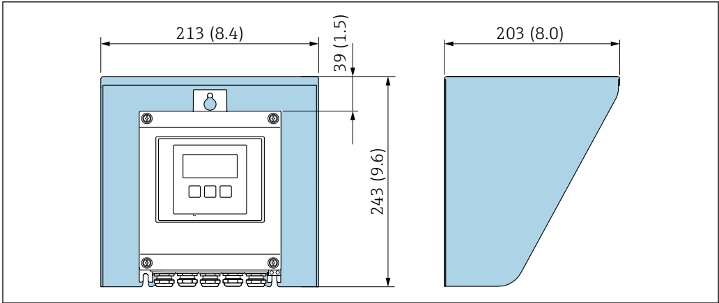
图 37 Proline 500（数字）的防护罩
