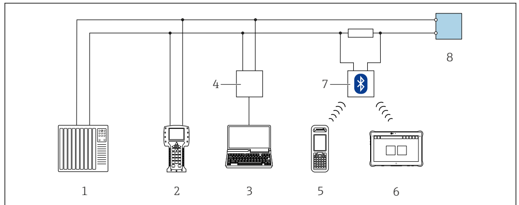
51 通过 HART 通信进行远程操作（有源信号）
