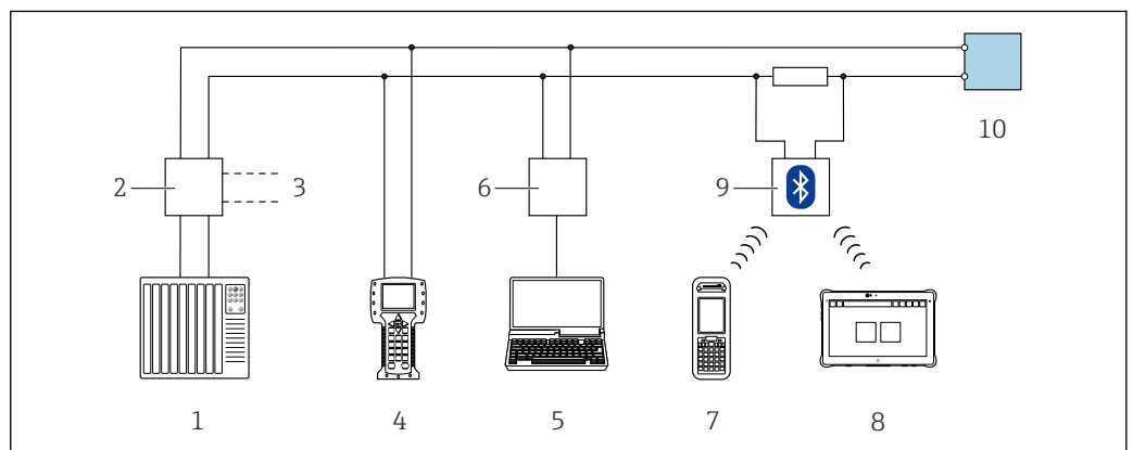
52 通过 HART 通信进行远程操作（无源信号）
