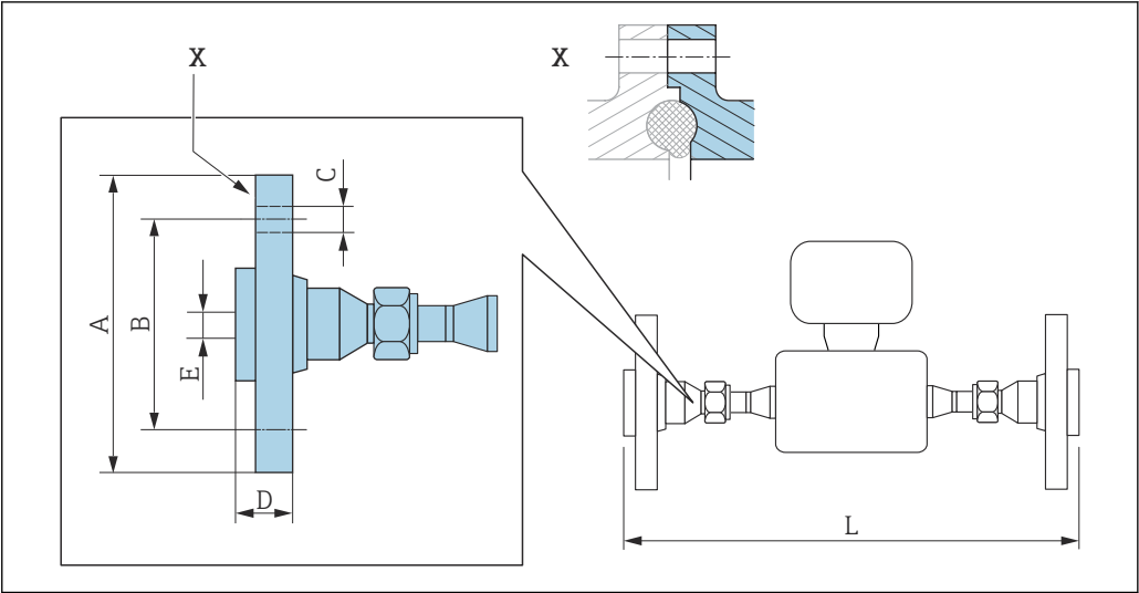
图 36 视图 X: 非对称过程连接; 蓝色部分由供应商提供
