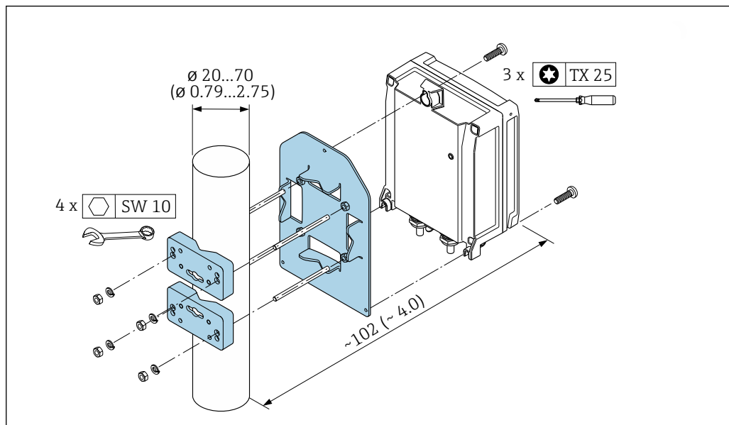
21 单位: mm (in)
