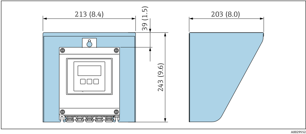
图 43 Proline 500（数字）的防护罩
