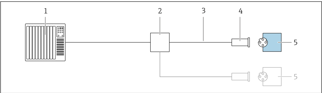
图 7 接线示例: PROFINET
