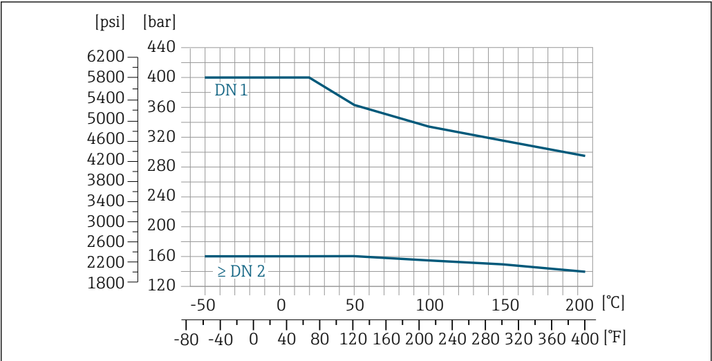
33 4-VCO-4 接头材质: Alloy C22 合金; ¼ NPT 螺纹接头材质: Alloy C22 合金; ¼"或⅛" SWAGELOK 接头材质: 1.4401 (316)
