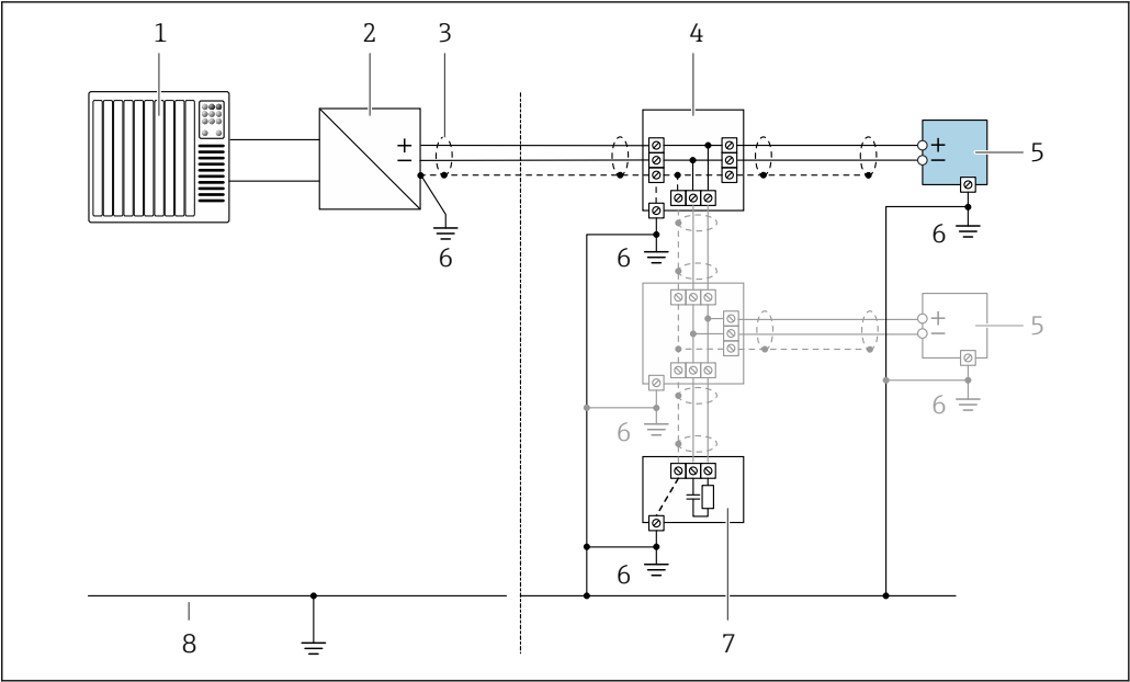
9 FOUNDATION Fieldbus 的连接实例
