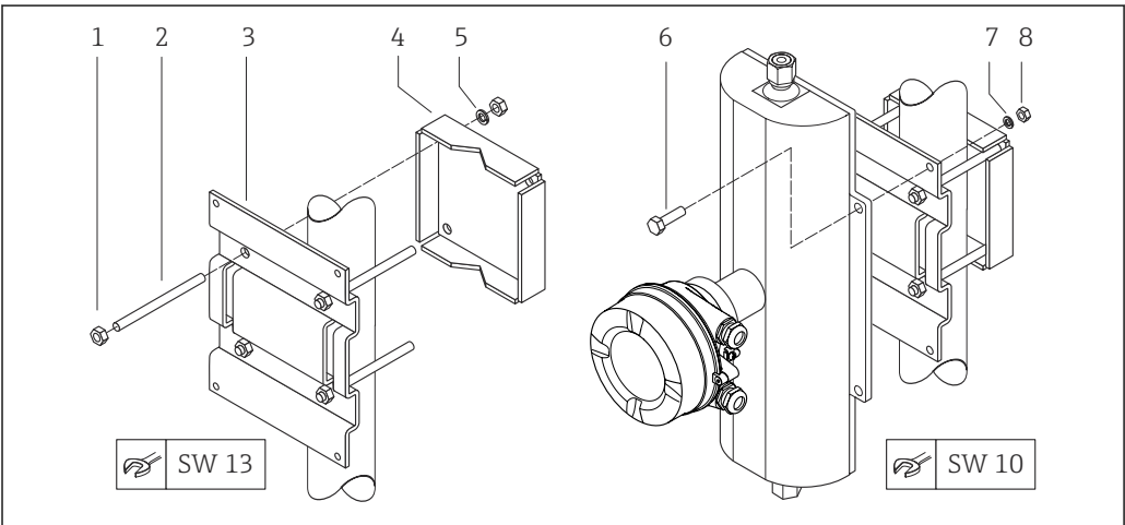
图 25 柱式安装套件
