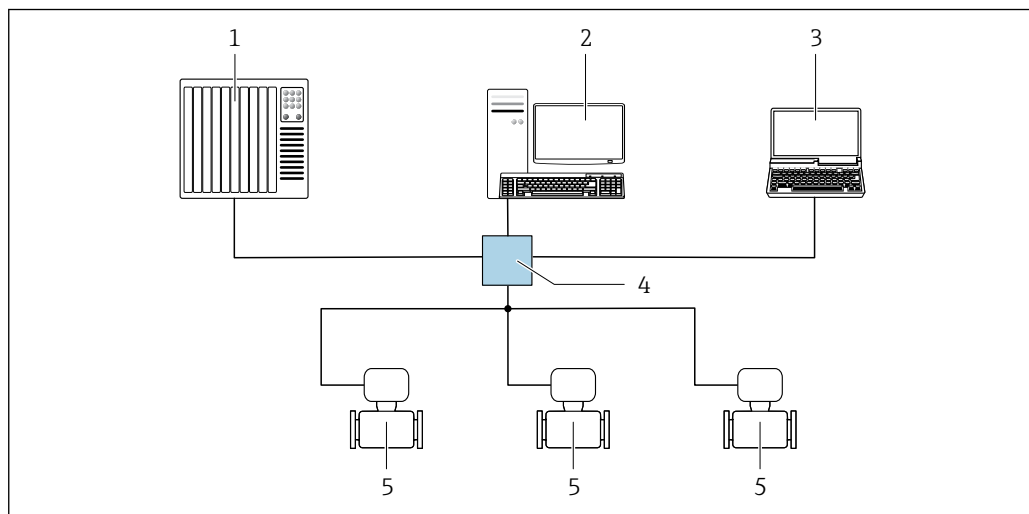
图 56 通过 Ethernet/IP 网络实现远程操作: 星形拓扑结构
