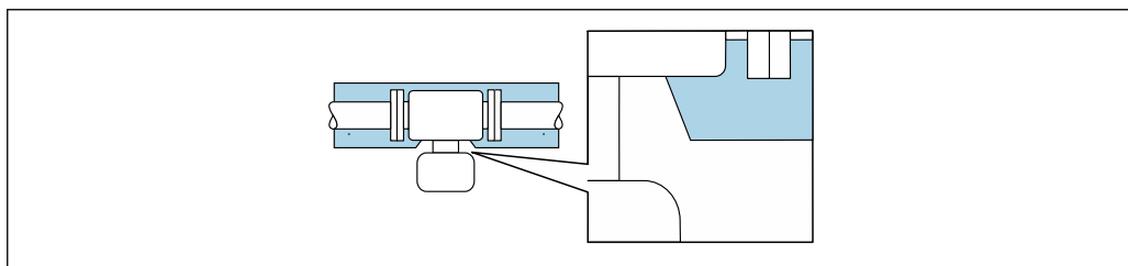
图 35 延长颈上无保温层覆盖
