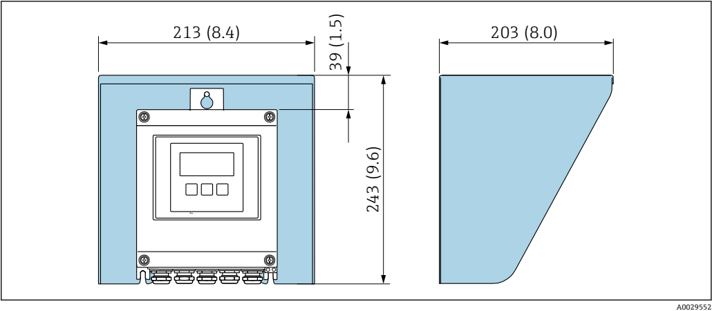
图 26 Proline 500（数字）的防护罩
