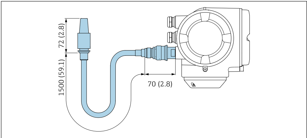
图 42 单位: mm (in)
