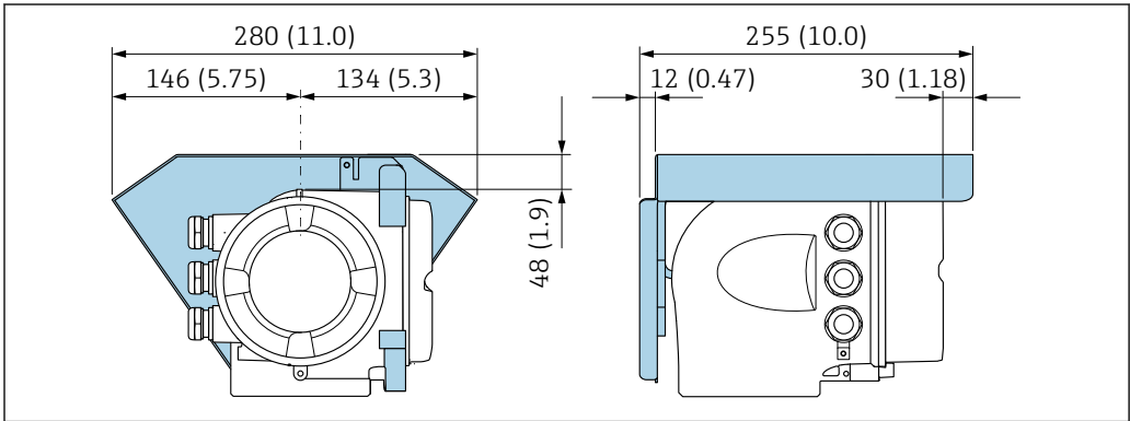
图 38 Proline 500（模拟）的防护罩
