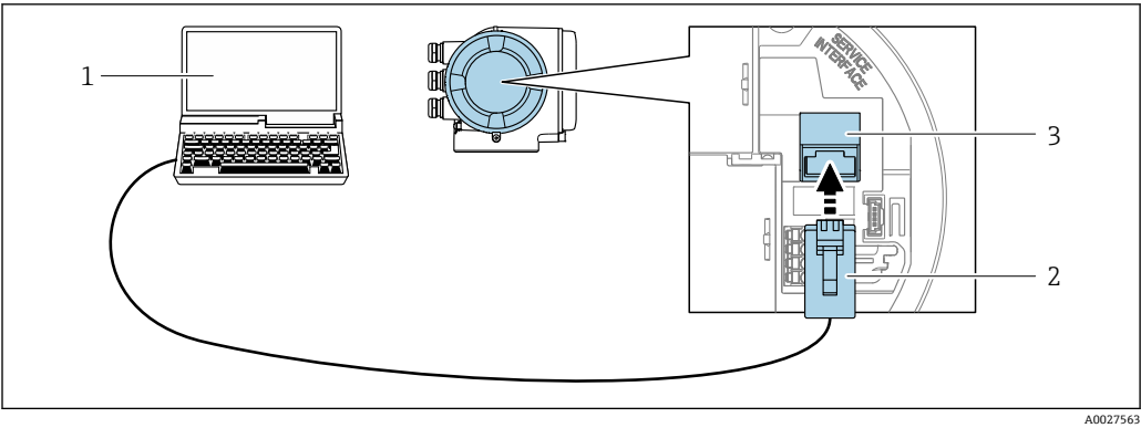
图 61 通过服务接口 (CDI-RJ45) 连接
