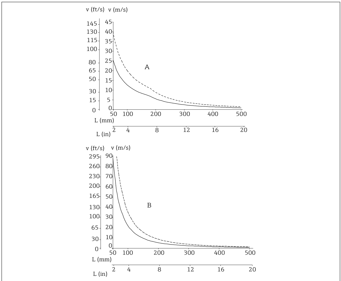
8 Velocità di deflusso in base alla lunghezza di immersione
