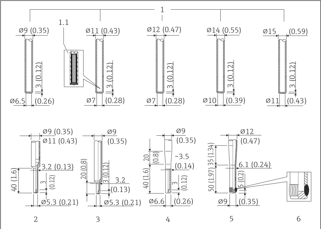
12 Puntali disponibili per i pozzetti (ridotto, rettilineo o rastremato). Rugosità massima Ra \leq 1,6 \mu m (62.9 \mu in )
