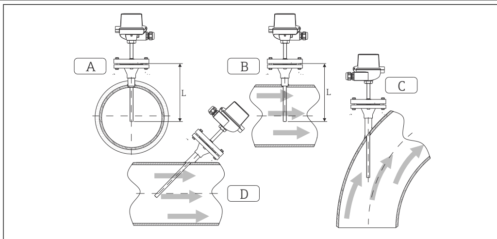
9 Esempi di installazione
