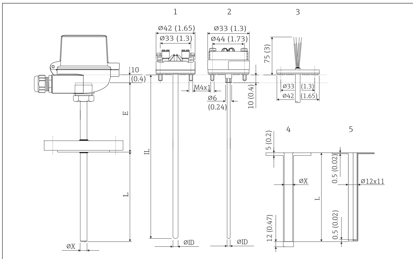
11 Dimensioni TR13 e TC13
