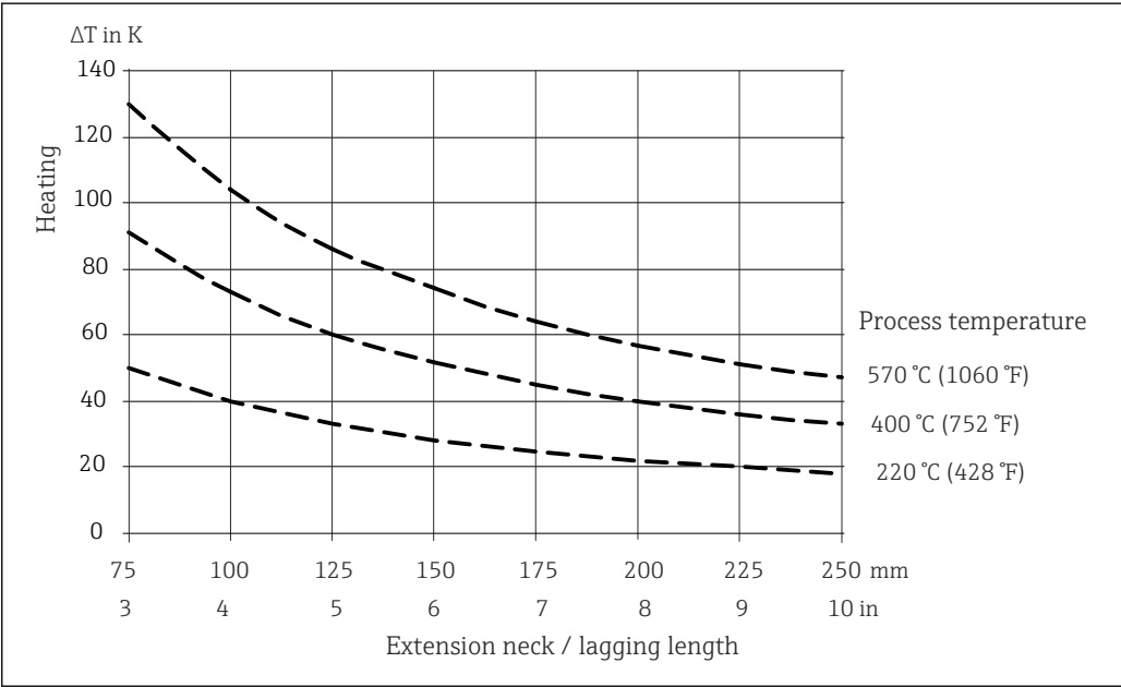
10 Riscaldamento della testa terminale in funzione della temperatura di processo. Temperatura nella testa terminale = temperatura ambiente 20 °C (68 °F) + ΔT
