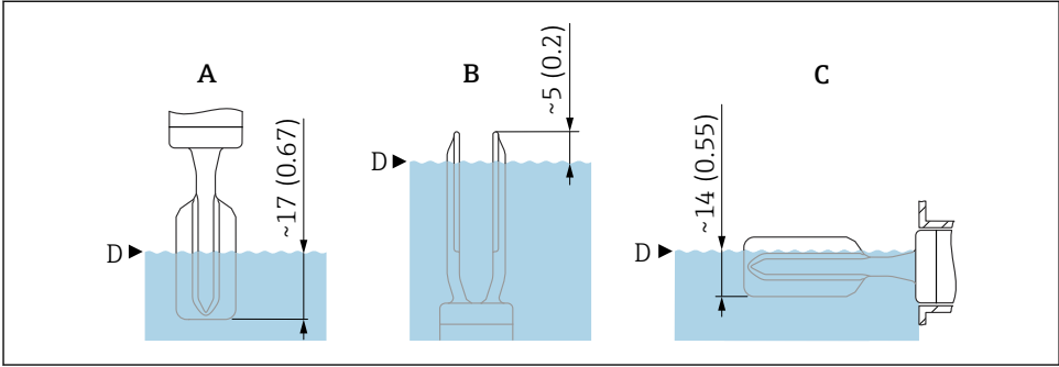
図 5 標準的なスイッチポイント、エナメルコーティング仕様の音叉部。測定単位 mm (in)
