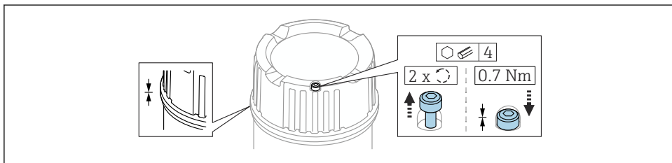
図 14 固定ネジ付きカバー
