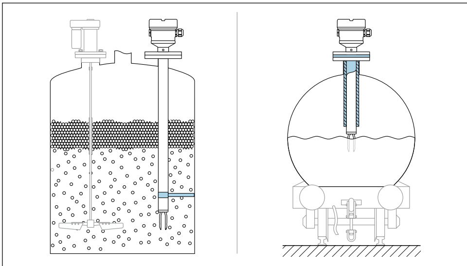
図 10 動的負荷が発生する場合の支持の例
