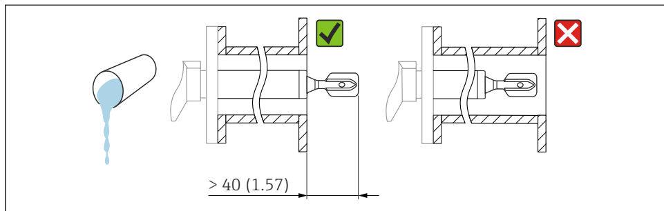
図 7 高粘度液体の設置例。測定単位 mm (in)
