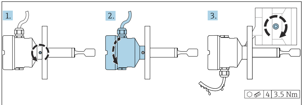
図 13 外部のロックネジおよびドリップループ付きハウジング
