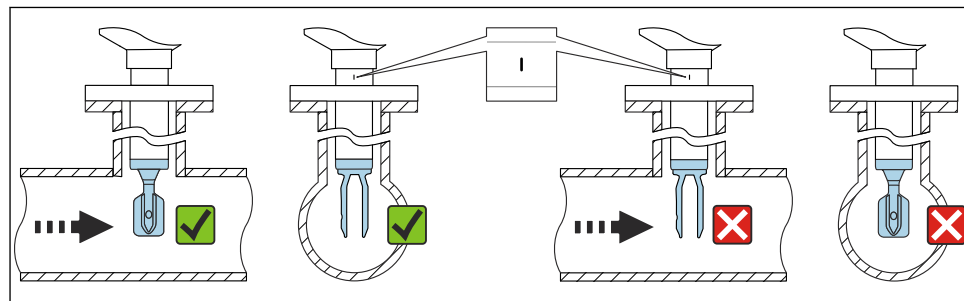
図 12 パイプへの設置（音叉部の位置とマークを考慮します）
