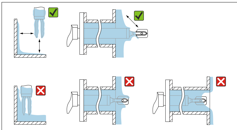
図 8 高粘度プロセス測定物の設置例
