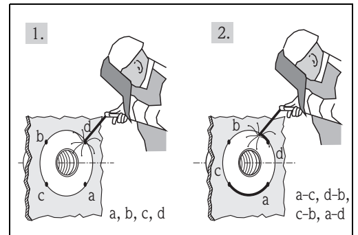
容器の溶接
