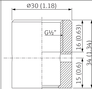
图 13 外形尺寸 (mm (in))
