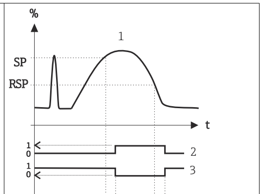
图 9 开关点 SP 和返回点 RSP
