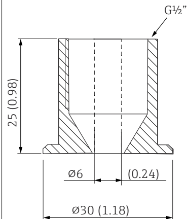
图 12 外形尺寸 (mm (in))
