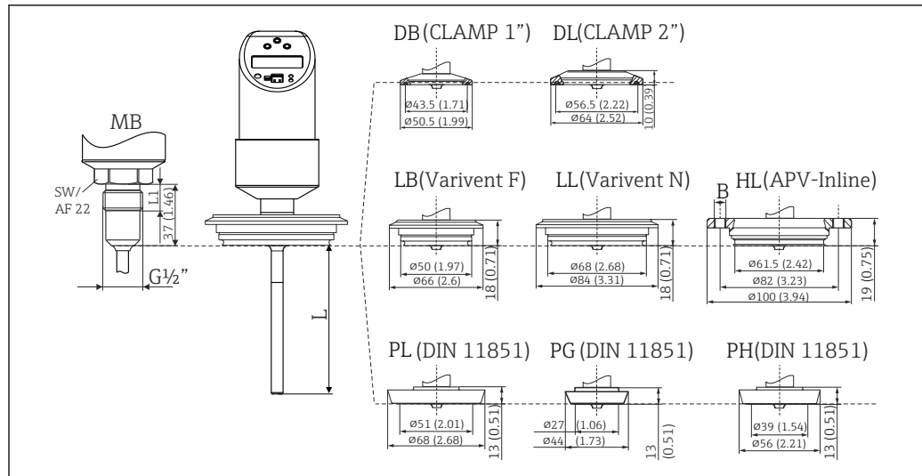
图 8 过程连接类型
