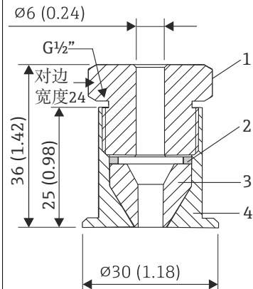
图 11 外形尺寸 (mm (in))
