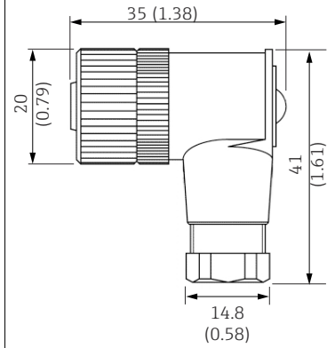
15 外形尺寸 (mm (in))
