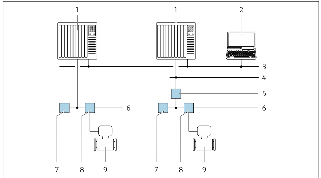
图 21 通过基金会现场总线(FF)网络进行远程操作
