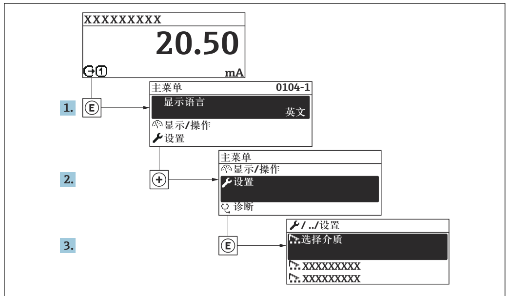
图 24 现场显示单元示例
