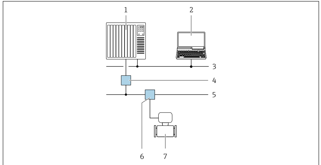
图 21 通过 PROFIBUS PA 网络进行远程操作
