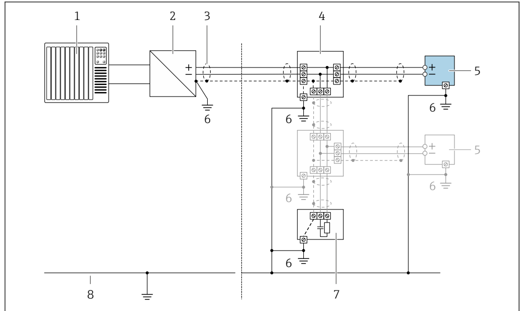
图 18 FOUNDATION Fieldbus 的连接实例
