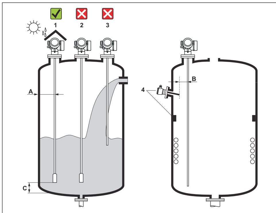
1 Montagebedingungen für Levelflex
