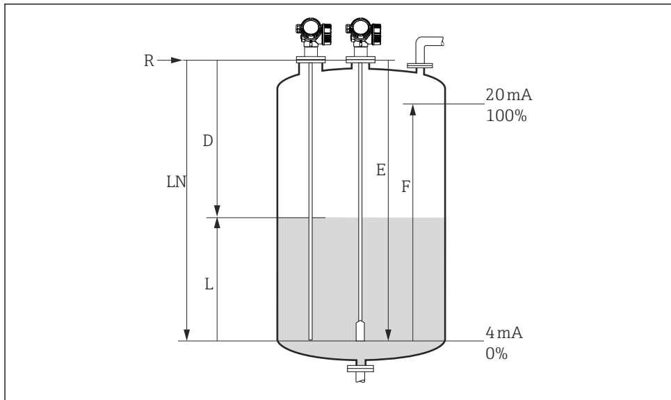
10 Konfigurationsparameter zur Füllstandmessung in Flüssigkeiten
