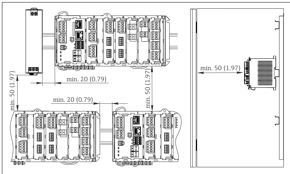
3 Minimum afstand in mm (in)
