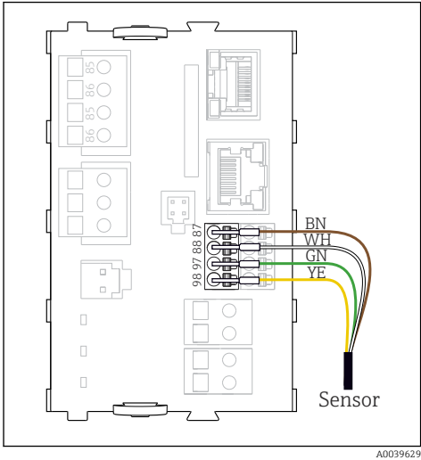
29 Memosens-sensoren zonder extra voedingsspanning
