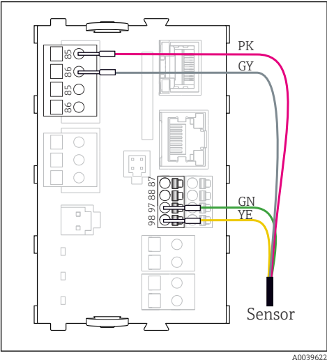
30 Memosens-sensoren met extra voedingsspanning
