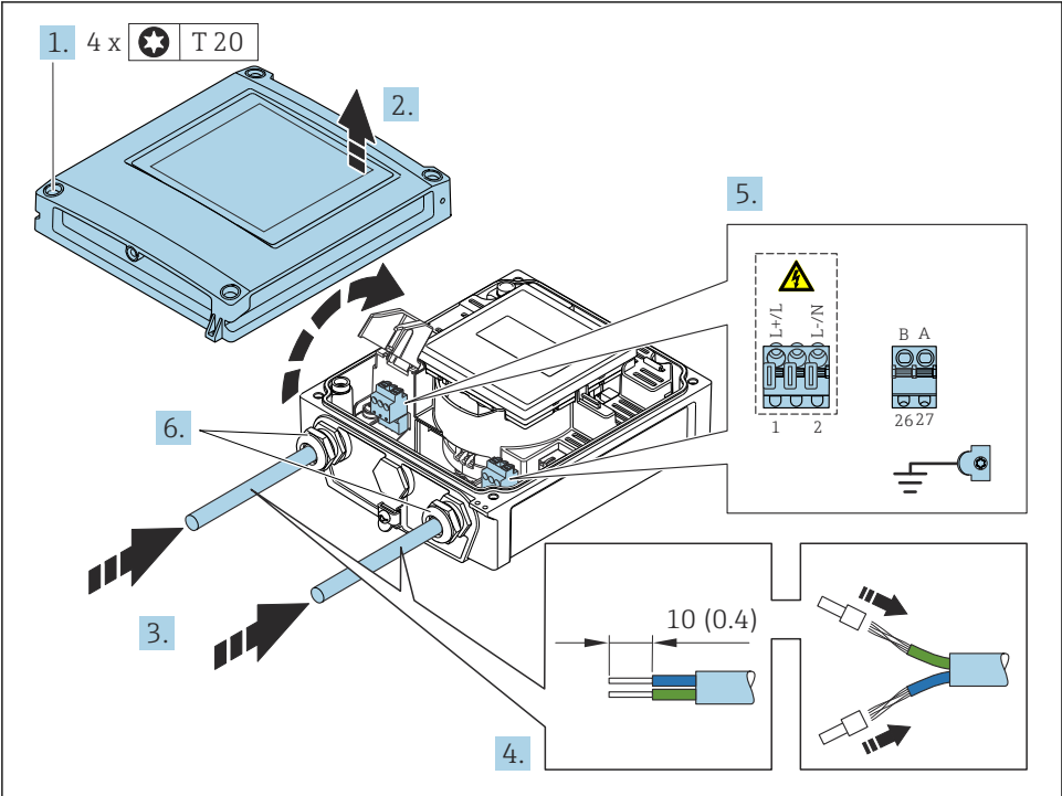
6 连接电源和 PROFIBUS DP
