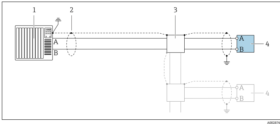
图 16 接线示例：PROFIBUS DP，非危险区和 Zone 2 / Div. 2 防爆场合
