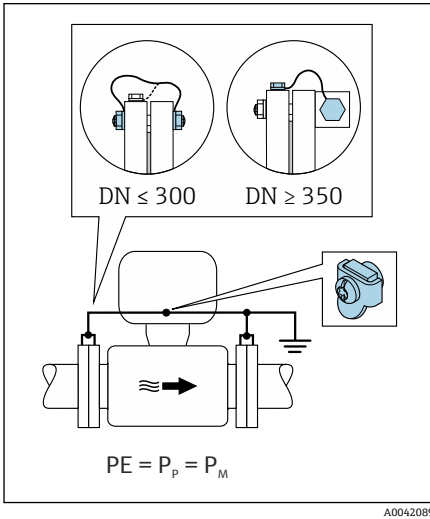
图 9 Promag L、W
