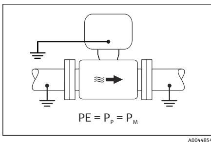
7 Promag L, W
