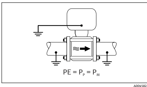
8 Promag D
