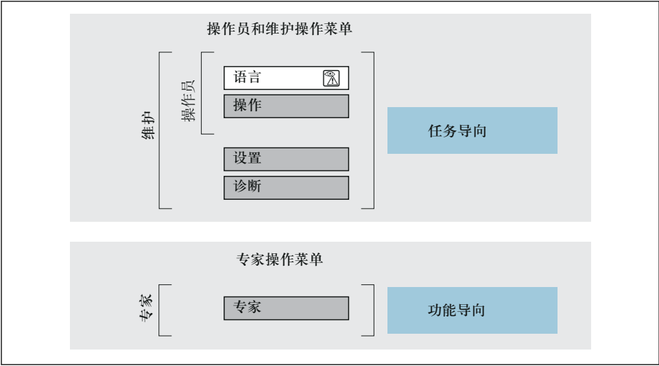
17 操作菜单的结构示意图
