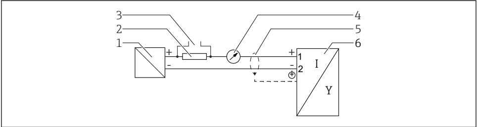
☐ 3 계통도, 2선식: 4~20 mA HART
