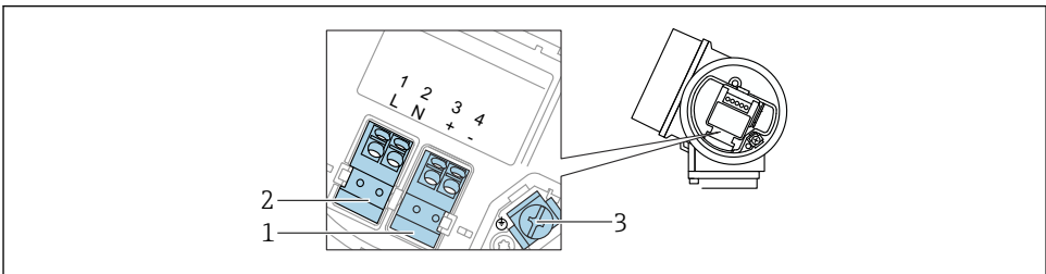
☐ 10 단자 할당, 4선식: 4~20 mA HART(90~253 V AC )
