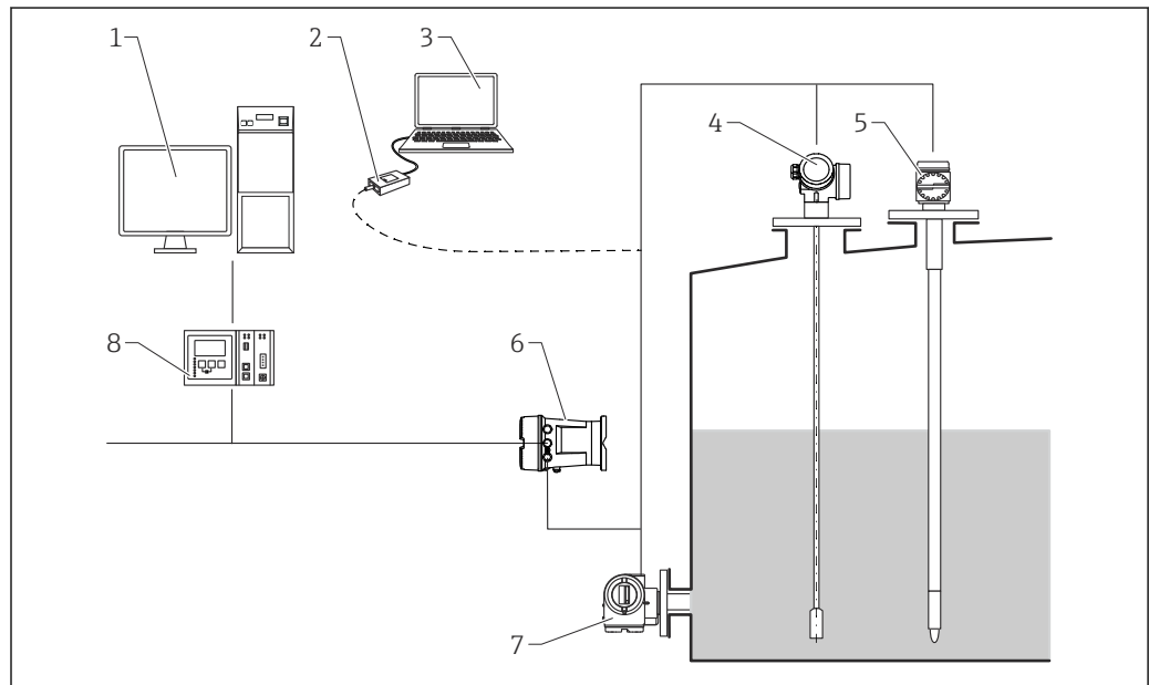
57 Die komplette Messeinrichtung besteht aus:
