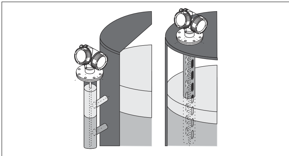
1 Levelflex FMP55 rögzítési helye
