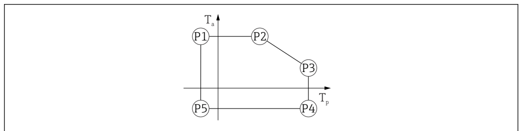
29 Gehäusematerial 316L; Prozesstemperaturbereich: -40 \dots +150 \text{ °C} ( -40 \dots +302 \text{ °F} )
