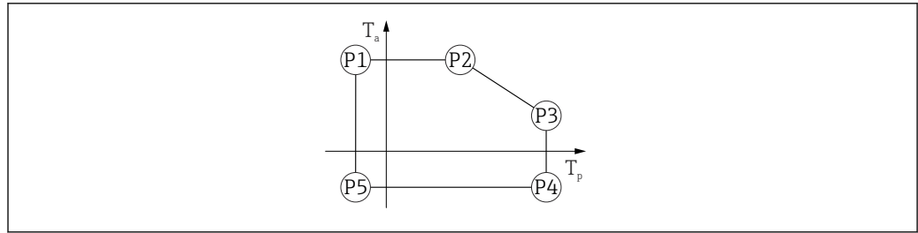
24 Gehäusematerial Aluminium; Prozesstemperaturbereich: -20 \dots +200 \text{ °C} ( -4 \dots +392 \text{ °F} )
