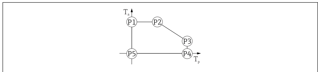
20 Gehäusematerial Kunststoff; Prozesstemperaturbereich: 0 \dots +150 \text{ °C} ( +32 \dots +302 \text{ °F} ) bei CSA C/US Zulassung
