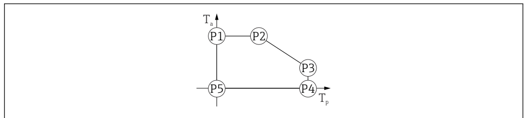
18 Gehäusematerial Kunststoff; Prozesstemperaturbereich: 0 ... +200 °C (+32 ... +392 °F) bei CSA C/US Zulassung
