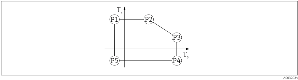
30 Gehäusematerial 316L; Prozesstemperaturbereich: -40 ... +200 °C (-40 ... +392 °F)
