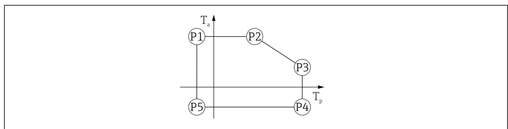
26 Gehäusematerial Aluminium; Prozesstemperaturbereich: -40 \dots +200 \text{ °C} ( -40 \dots +392 \text{ °F} )
