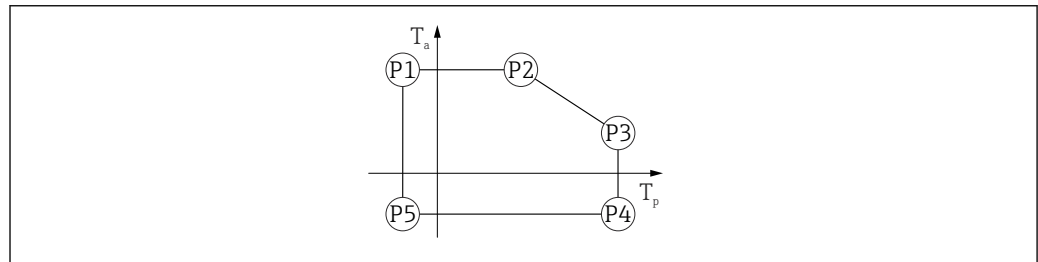
15 Gehäusematerial Kunststoff; Prozesstemperaturbereich: -20 ... +150 °C (-4 ... +302 °F)
