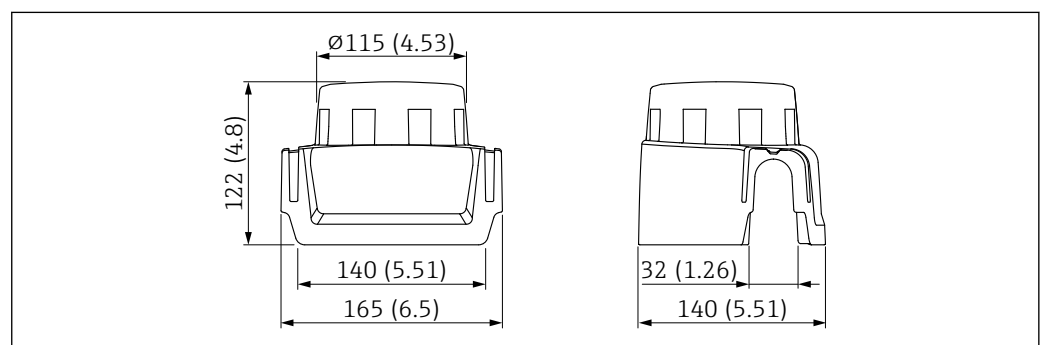
14 Abmessungen. Maßeinheit mm (in)
