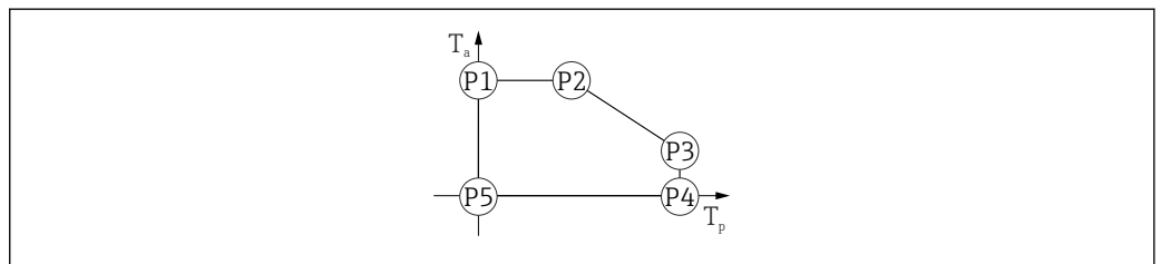
22 Gehäusematerial Kunststoff; Prozesstemperaturbereich: 0 \dots +200 \text{ }^{\circ}\text{C} ( +32 \dots +392 \text{ }^{\circ}\text{F} ) bei CSA C/US Zulassung
