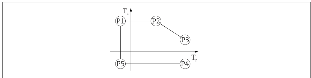
25 Gehäusematerial Aluminium; Prozesstemperaturbereich: -40 \dots +150 \text{ °C} ( -40 \dots +302 \text{ °F} )
