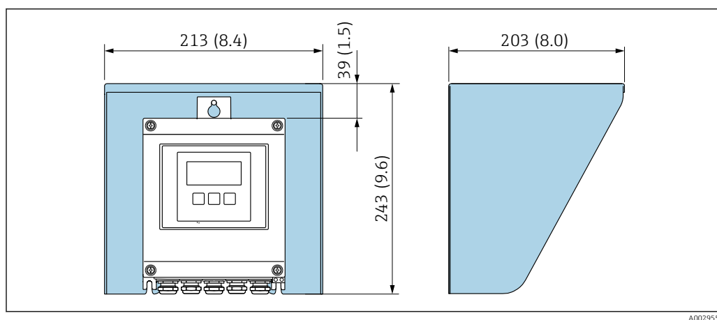
64 Wetterschutzhaube Proline 500 – digital; Maßeinheit mm (in)
