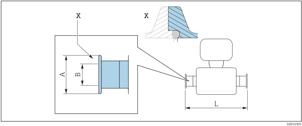
61 Detail X: Asymmetrischer Prozessanschluss, der blau markierte Teil ist lieferseitig.
