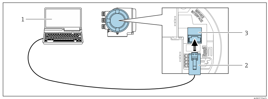
84 Anschluss via Serviceschnittstelle (CDI-RJ45)
