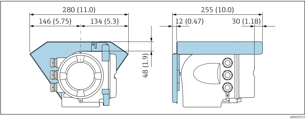
29 Wetterschutzhaube Proline 500; Maßeinheit mm (in)
