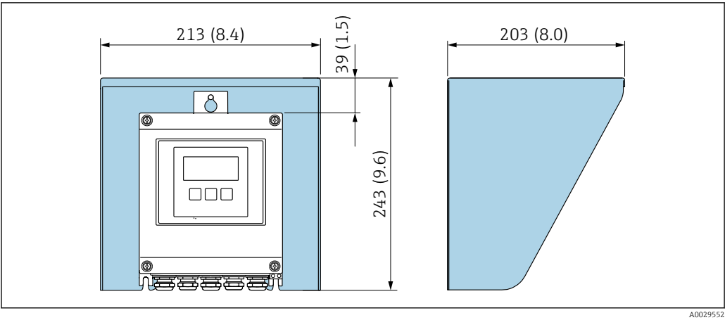
28 Wetterschutzhaube Proline 500 – digital; Maßeinheit mm (in)
