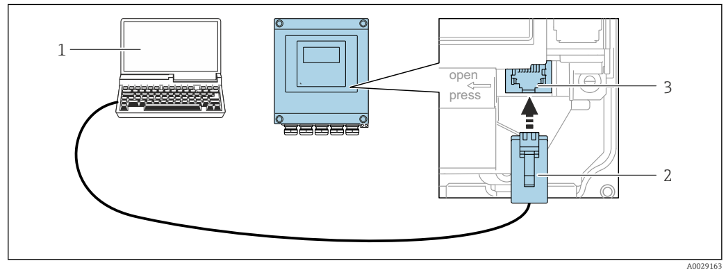
83 Anschluss via Service-Schnittstelle (CDI-RJ45)
