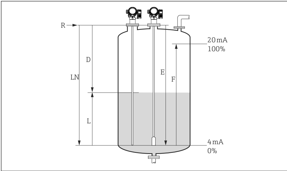
10 Parámetros de configuración para la medición de nivel en líquidos
