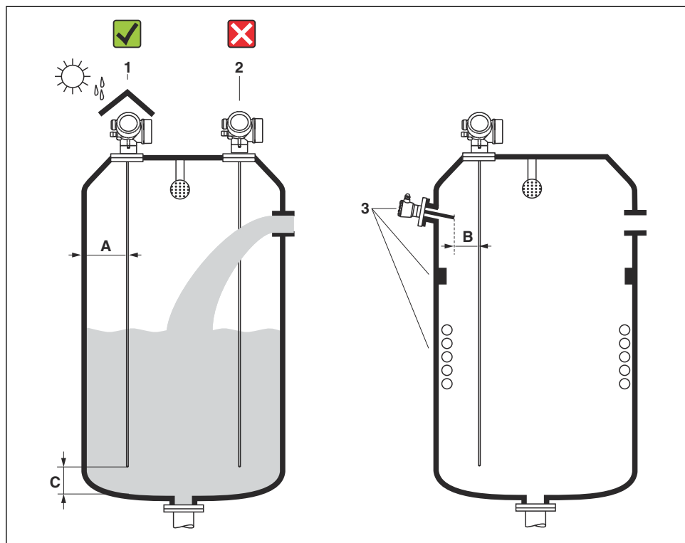
1 Conditions de montage pour le Levelflex
