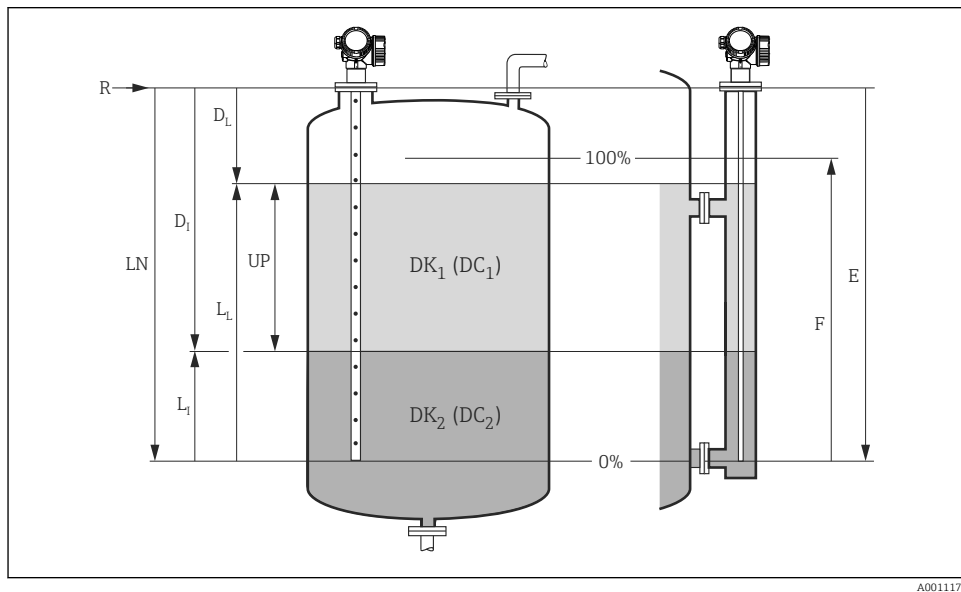
11 Parámetros de configuración para la medición de la interfase
