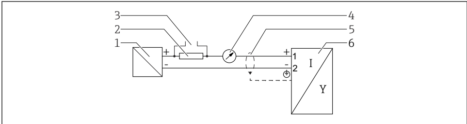
☐ 4 계통도, 2선식: 4~20 mA HART
