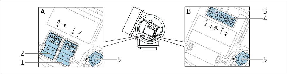
☐ 7 단자 할당, 2선식: 4~20 mA HART, 4~20 mA
