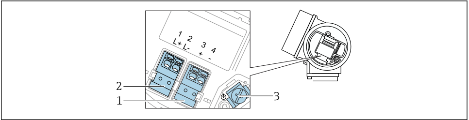
☐ 9 단자 할당, 4선식: 4~20 mA HART(10.4~48 V DC )
