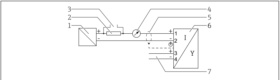
☐ 6 계통도, 2선식: 4~20 mA HART, 스위치 출력
