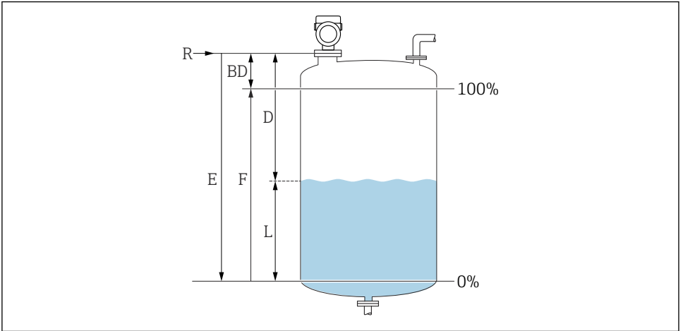
☐ 21 액체 레벨 측정 구성 파라미터
