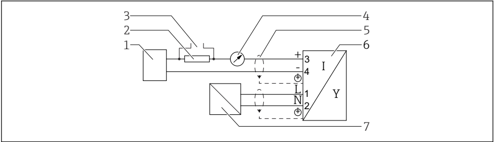
12 계통도, 4선식: 4~20 mA HART (90~253 V AC )
