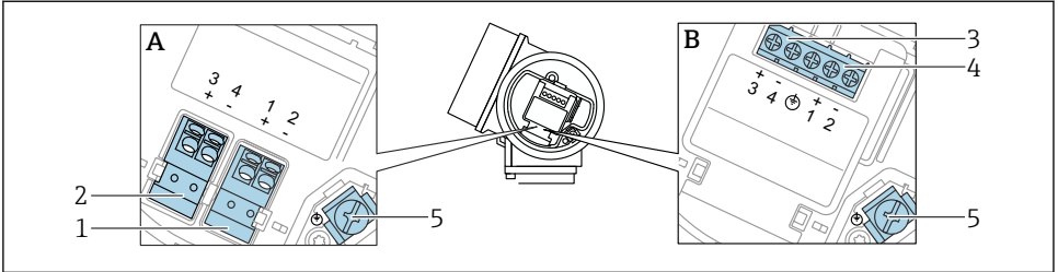
☐ 5 단자 할당, 2선식: 4~20 mA HART, 스위치 출력
