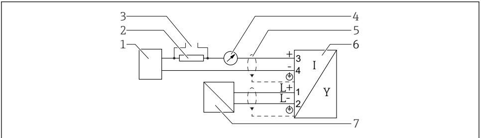
☐ 10 계통도, 4선식: 4~20 mA HART(10.4~48 V DC )
