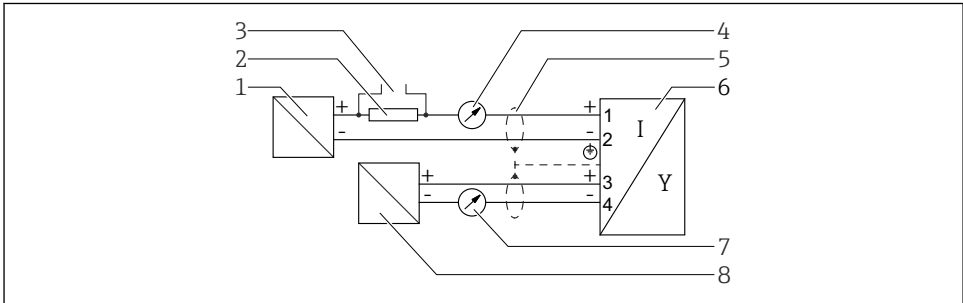
☐ 8 계통도, 2선식: 4~20 mA HART, 4~20 mA
