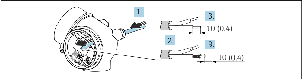
☞ 15 공학 단위: mm (in)
