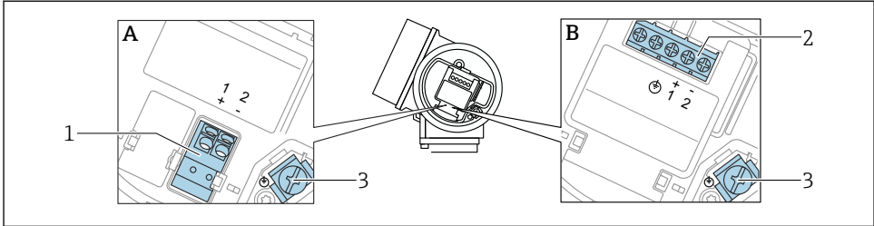
☐ 3 단자 할당, 2선식: 4~20 mA HART
