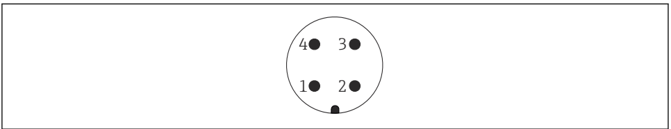
13 M12 플러그의 핀 할당
