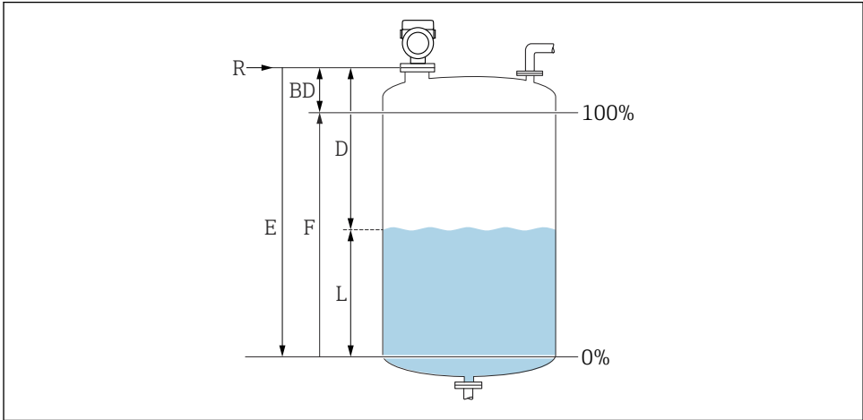
☐ 22 액체 레벨 측정 구성 파라미터
