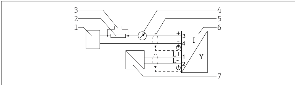
☐ 11 계통도, 4선식: 4~20 mA HART(10.4~48 V DC )
