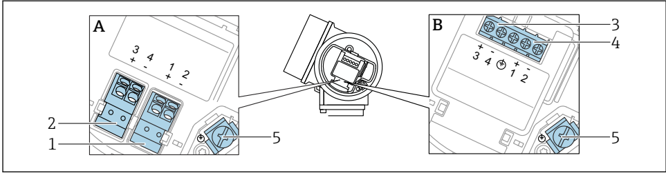
☐ 6 단자 할당, 2선식: 4~20 mA HART, 스위치 출력
