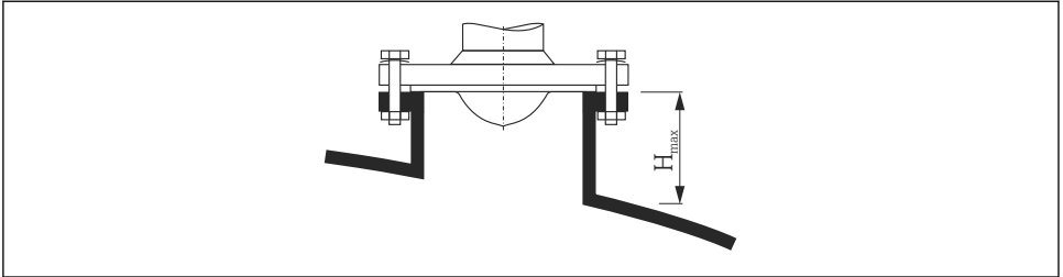
☐ 3 혼 안테나의 노즐 높이, 플러시 설치(FMR52)
