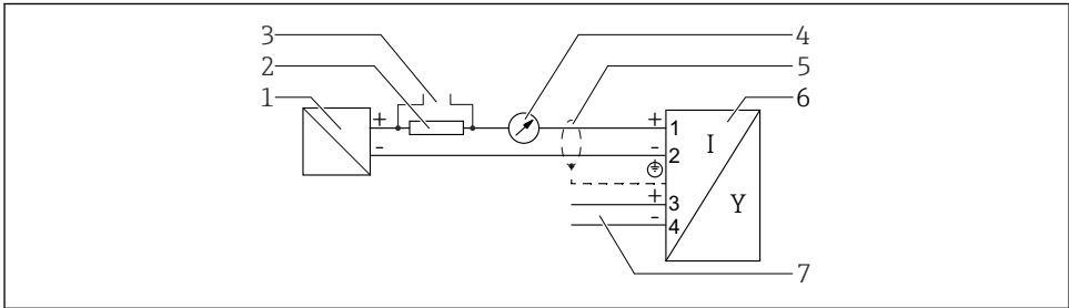
☐ 7 계통도, 2선식: 4~20 mA HART, 스위치 출력
