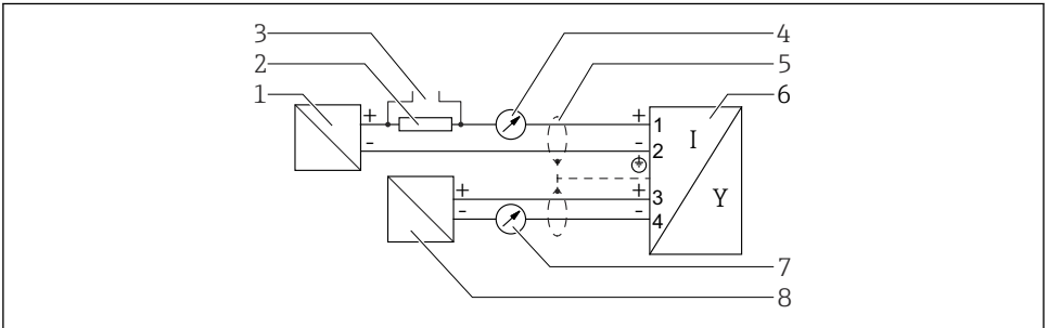
☐ 9 계통도, 2선식: 4~20 mA HART, 4~20 mA
