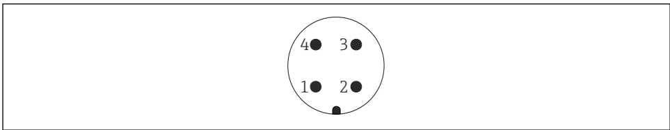
☐ 14 M12 플러그의 핀 할당
