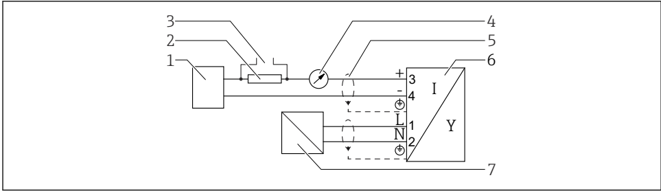
☐ 13 계통도, 4선식: 4~20 mA HART(90~253 V AC )
