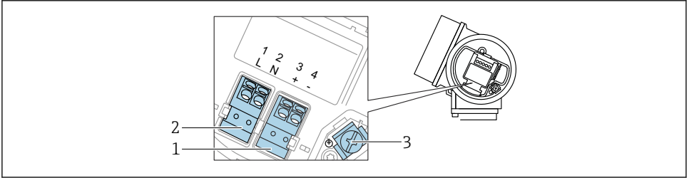
☐ 12 단자 할당, 4선식: 4~20 mA HART(90~253 V AC )
