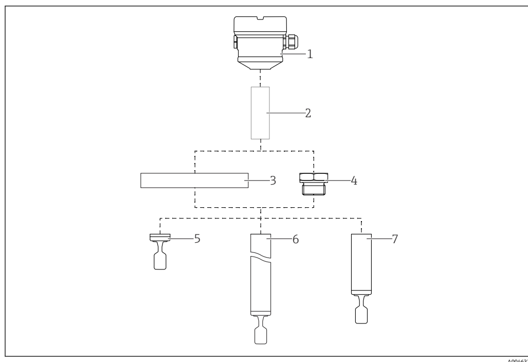
図 1 製品構成
