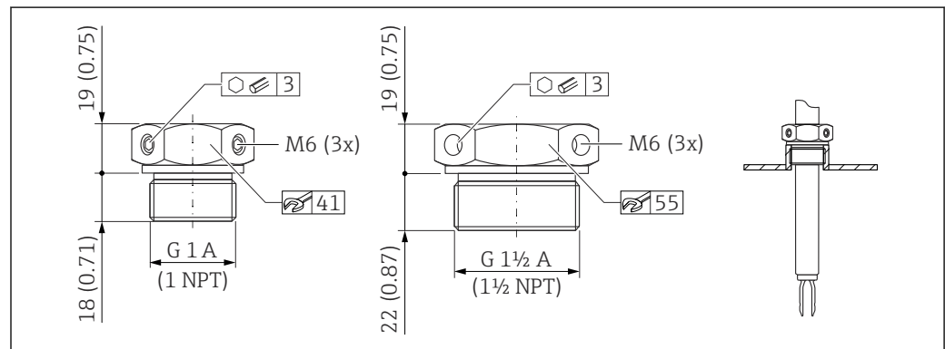
図 50 スライディングスリーブ (大気圧用： p_e = 0 \text{ MPa} (0 psi))。測定単位 mm (in)
