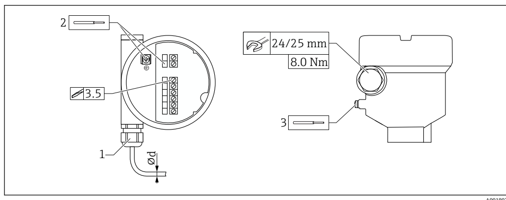
図 31 カップリングの例（電線管接続口、エレクトロニックインサートと端子）
