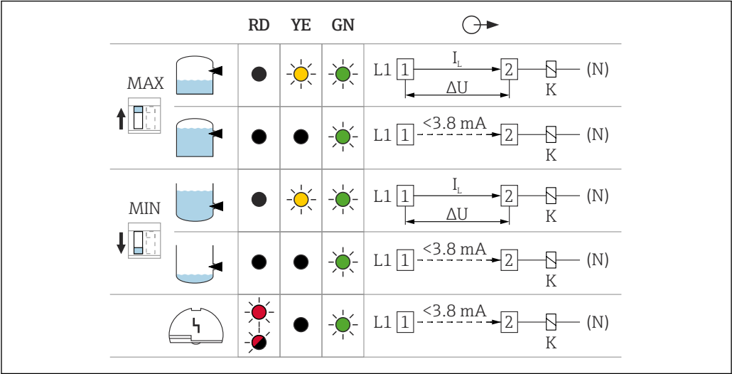
図 17 スwitch出力および信号伝達の動作、エレクトロニックインサート FEL61
