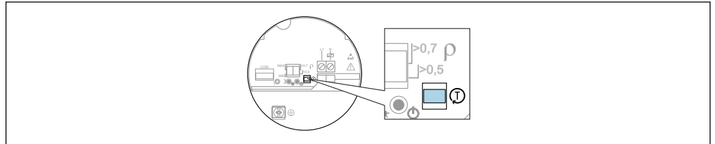
図 34 機能テスト用のキー (エレクトロニックインサート FEL61/62/64/64DC/67/68)
