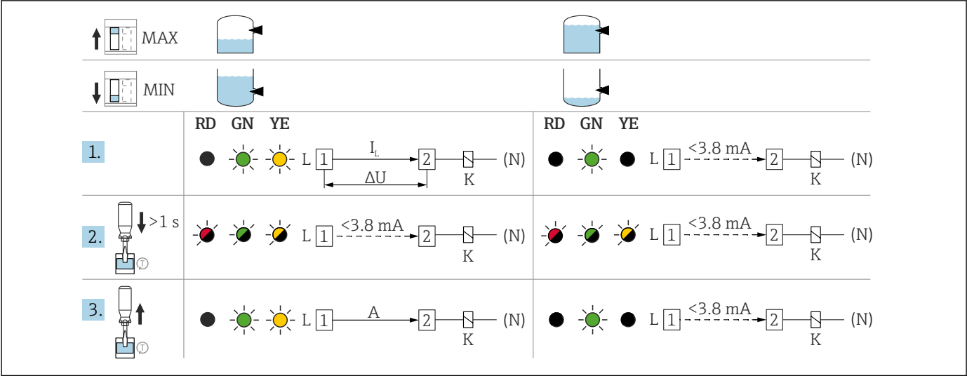
35 FEL61 スイッチング動作および信号伝達
