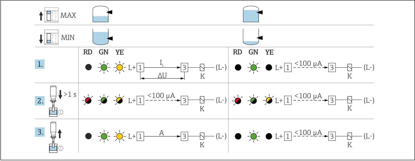
36 FEL62 スイッチング動作および信号伝達
