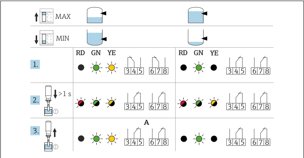
37 FEL64、FEL64DC スイッチング動作および信号伝達
