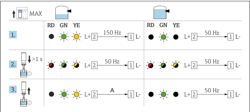
38 FEL67 上限 (MAX) スイッチング動作および信号伝達
