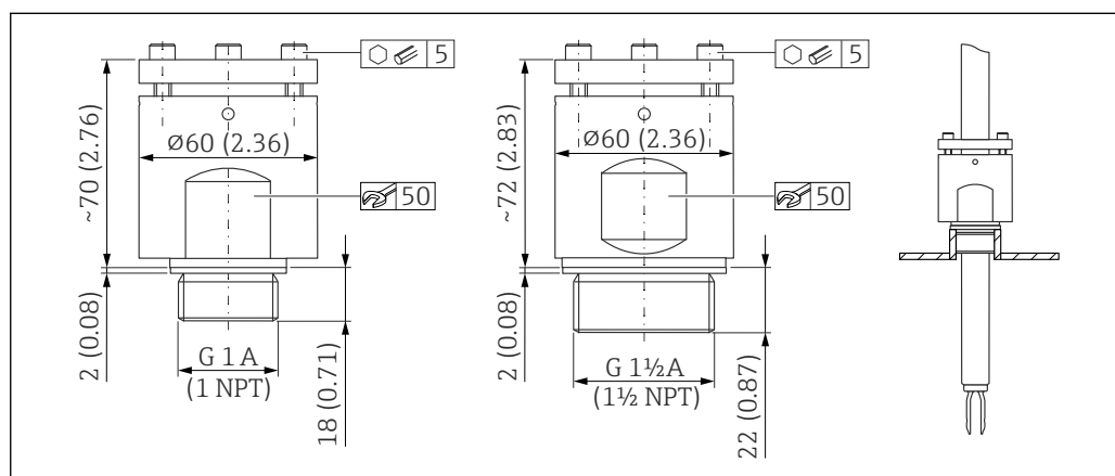
図 51 高圧用スライディングスリーブ。測定単位 mm (in)
