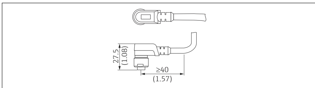
47 プラグコネクタ M12 IP67。測定単位 mm (in)
