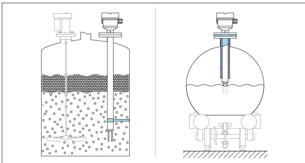
図 9 動的負荷が発生する場合の支持の例
