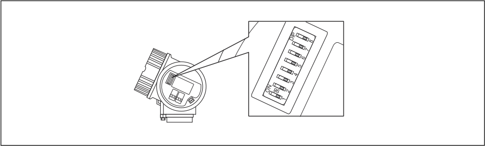
9 Interruptor de dirección en el compartimento de conexiones
