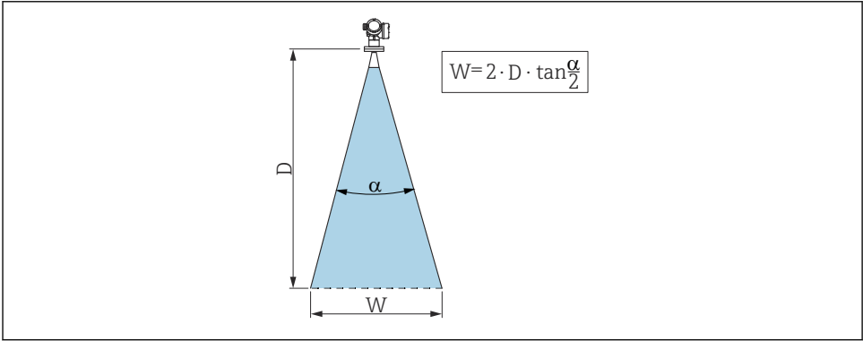
1 Relación entre ángulo de abertura del haz \alpha , distancia D y diámetro del haz W
