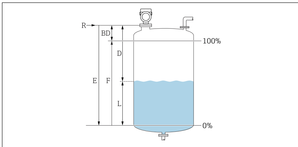
16 Parámetros de configuración para la medición de nivel en líquidos
