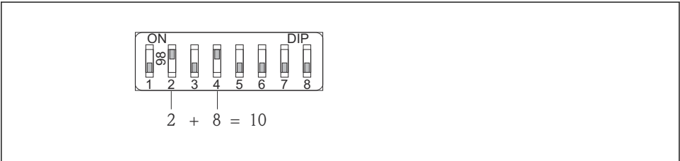
10 Ejemplo de un ajuste de dirección mediante hardware; microinterruptor 8 en posición "OFF" y los microinterruptores 1 a 7 definen la dirección.
