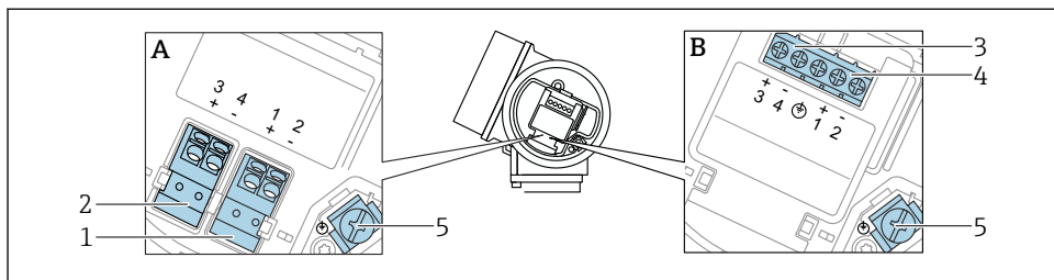
4 Esquema de ligação elétrica PROFIBUS PA / FOUNDATION Fieldbus
