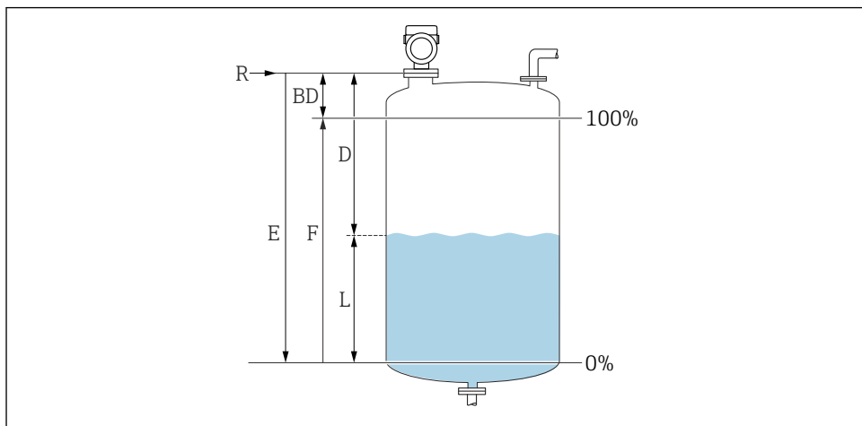
16 Parâmetros de configuração para as medições de nível em líquidos
