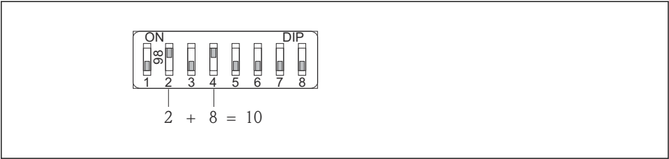
10 Exemplo de endereçamento de hardware: a seletora 8 é definida na posição "OFF"; as seletoras 1 a 7 definem o endereço.
