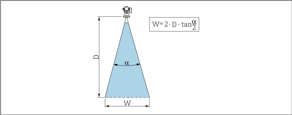
1 Relação entre o ângulo do feixe \alpha , a distância D e o diâmetro da largura do feixe W
