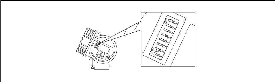
図 13 端子部のアドレススイッチ
