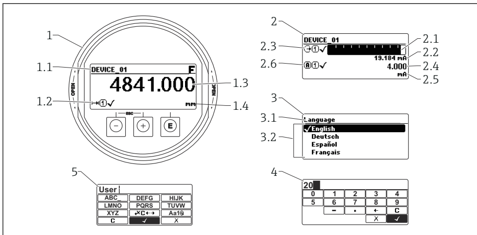
図 17 表示モジュールおよび操作モジュールの表示形式
