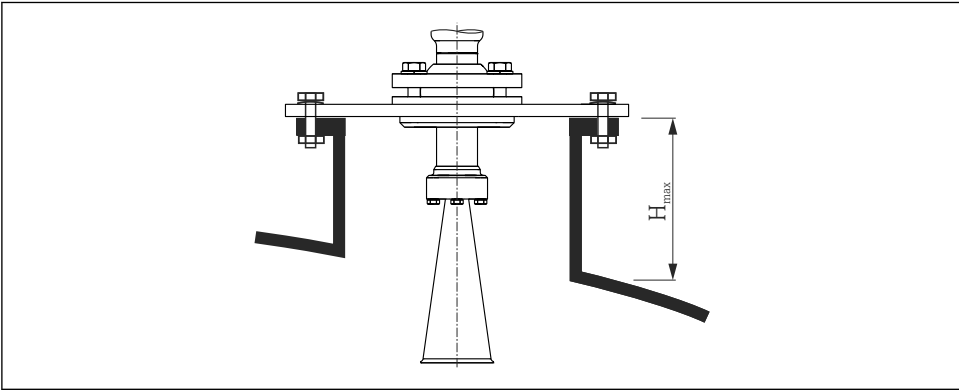
図 4 ホーンアンテナのノズル高 (FMR57)
