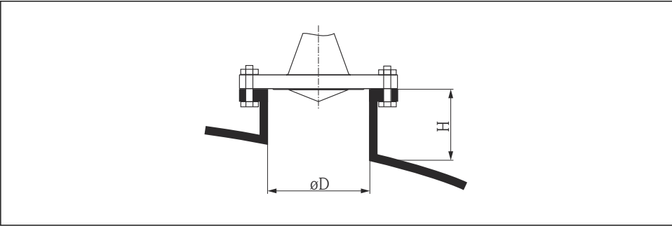
2 スリップオンフランジ付きホーンアンテナのノズル直径とノズル高
