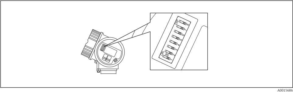
13 Microinterruttore dell'indirizzo nel vano connessioni
