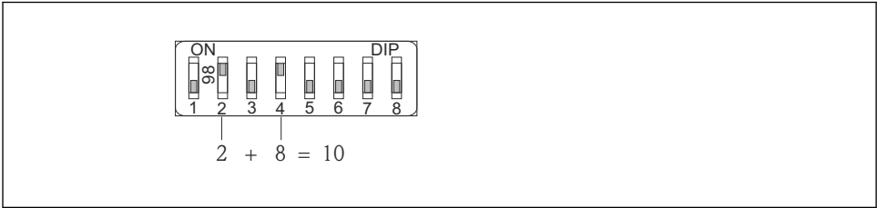
14 Esempio di indirizzamento hardware: il microinterruttore 8 è in posizione "OFF"; i microinterruttori 1...7 definiscono l'indirizzo.
