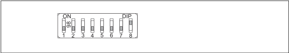
15 Esempio di indirizzamento software; il microinterruttore 8 è in posizione "ON"; l'indirizzo è definito nel menu operativo (Configurazione → Indirizzo dispo.).
