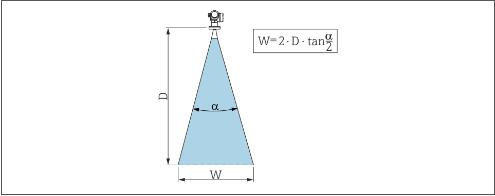
1 Взаимосвязь между углом расхождения луча \alpha , расстоянием D и диаметром луча W
