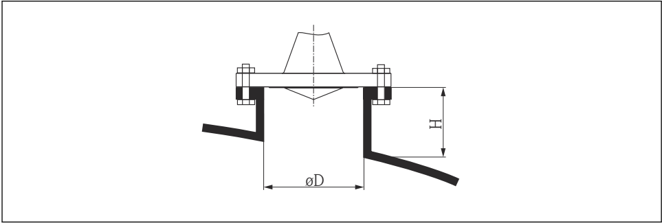
2 Высота и диаметр штуцера для рупорной антенны с накидным фланцем
