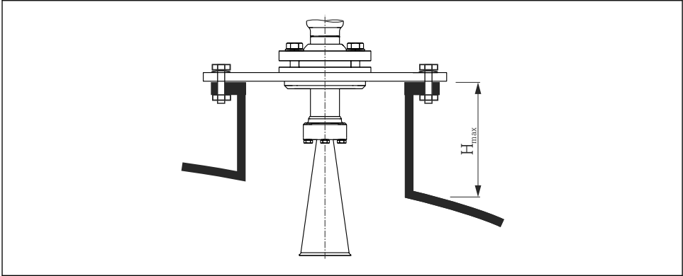
4 Высота штучера для рупорной антенны (FMR57)
