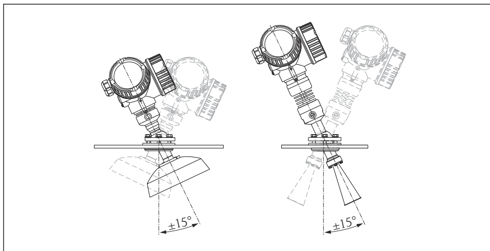
6 Прибор Micropilot FMR57 с приспособлением для выравнивания
