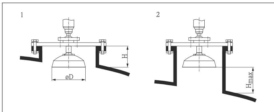
5 Монтаж Micropilot FMR57 с параболической антенной в штупер
