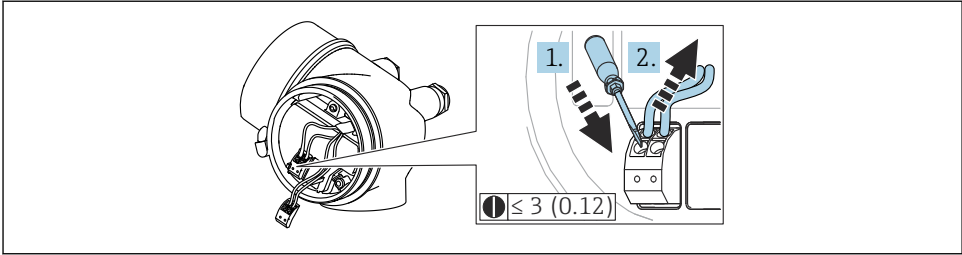
12 Единица измерения: мм (дюйм)
