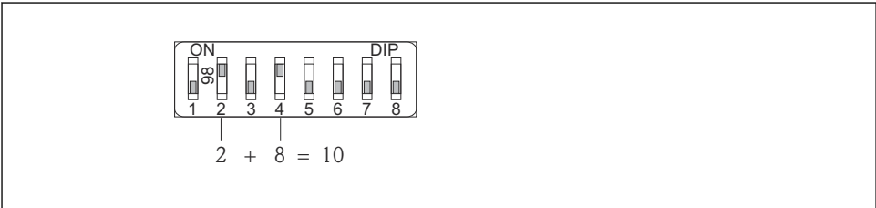
14 Ejemplo de un ajuste de dirección mediante hardware; microinterruptor 8 en posición "OFF" y los microinterruptores 1 a 7 definen la dirección.
