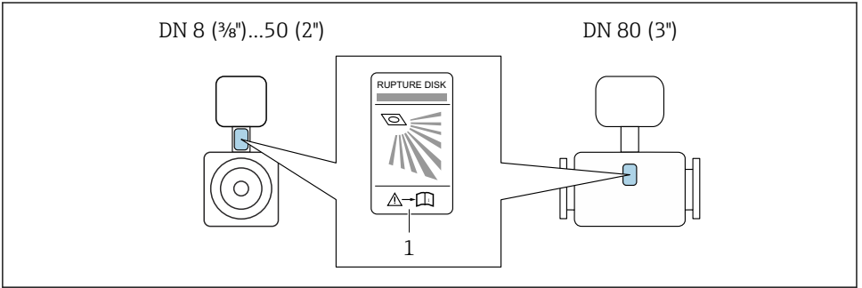
1 파열판 라벨
