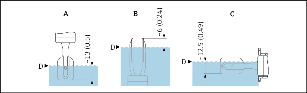
5 塑料涂层叉体的常见开关点。测量单位 mm (in)
