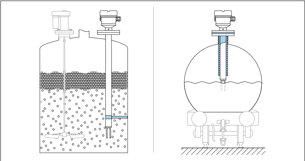
图 11 存在动态负载时，支撑设备的实例
