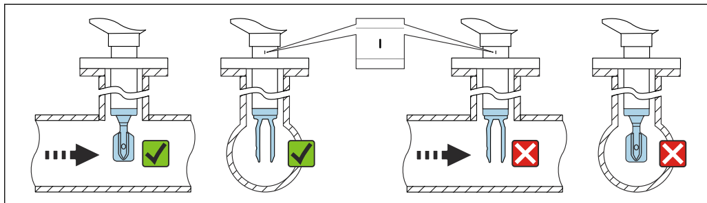
图 13 安装在管道内（根据叉体的位置和标记安装）
