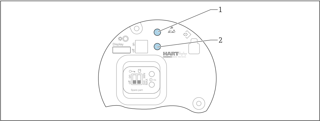
图 26 电子插件上的操作按键
