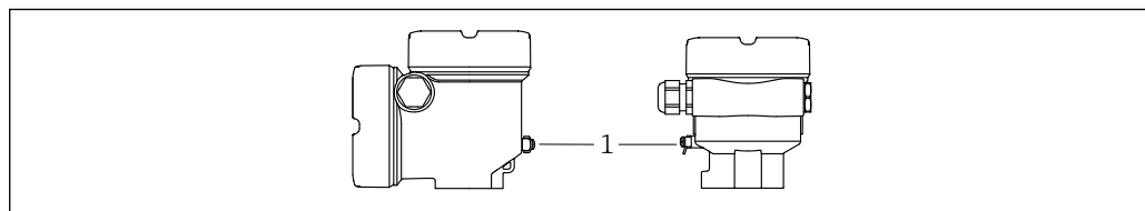
1 接地端，连接等电势线
