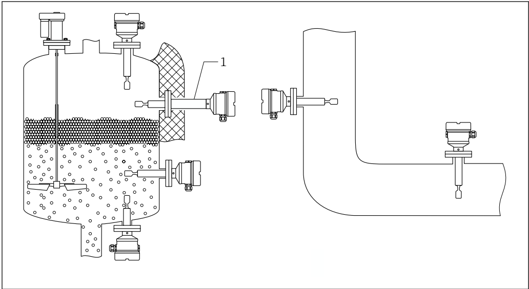
3 安装在容器、管道或罐体中使用的实例
