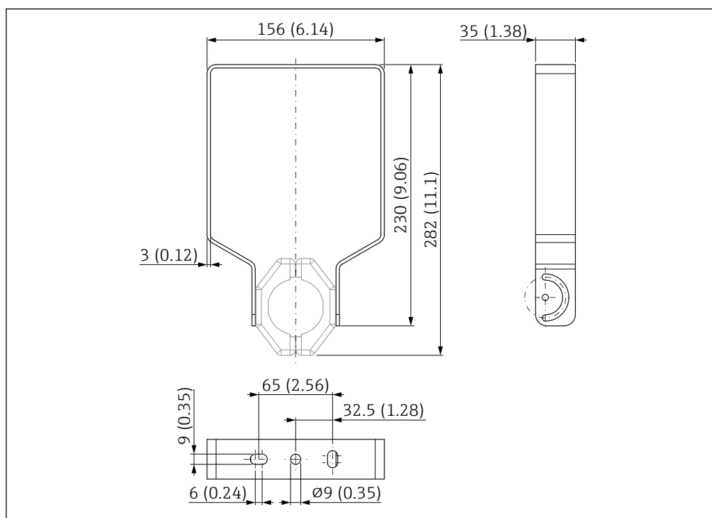
36 Dimensions de l'étrier de montage. Unité de mesure mm (in)
