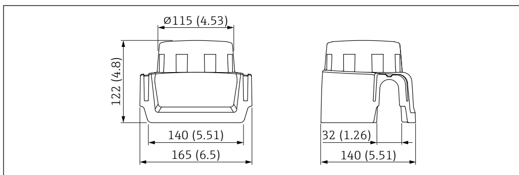
34 Dimensions. Unité de mesure mm (in)
