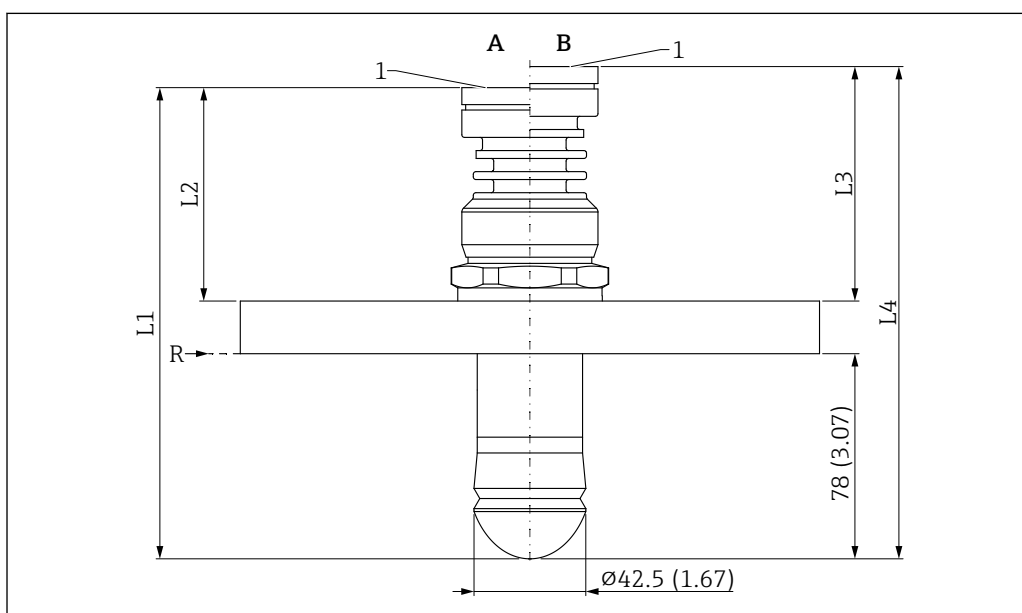
■ 25 Dimensions de l'antenne drip-off 50 mm (2 in), bride UNI raccord process. Unité de mesure mm (in)
