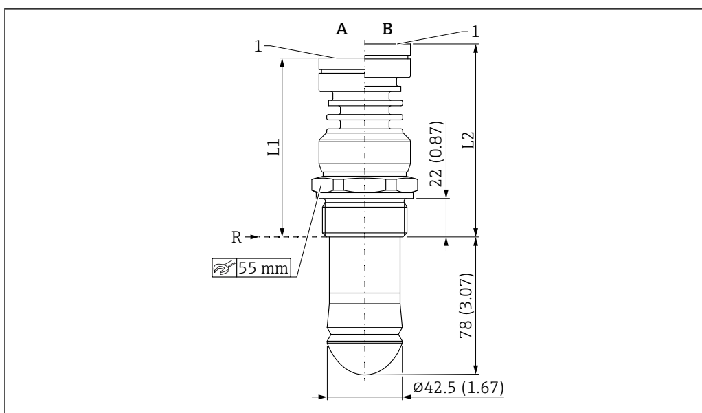
■ 24 Dimensions de l'antenne drip-off 50 mm (2 in), raccord process fileté. Unité de mesure mm (in)
