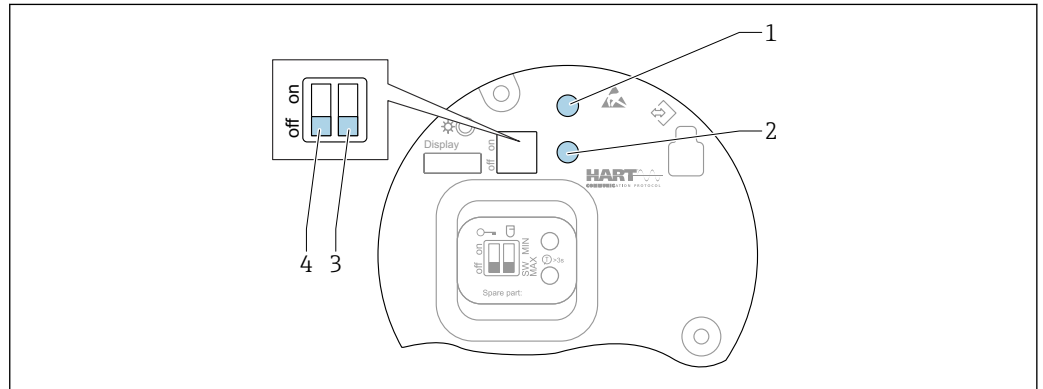
31 Touches de configuration et commutateurs DIP sur l'électronique HART
