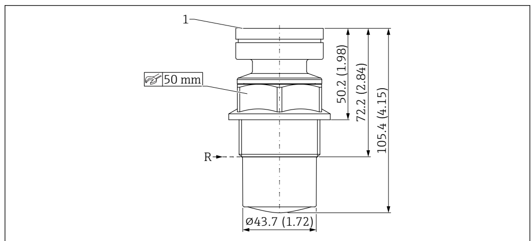
19 Dimensions de l'antenne encapsulée, PVDF, 40 mm (1,5 in). Unité de mesure mm (in)
