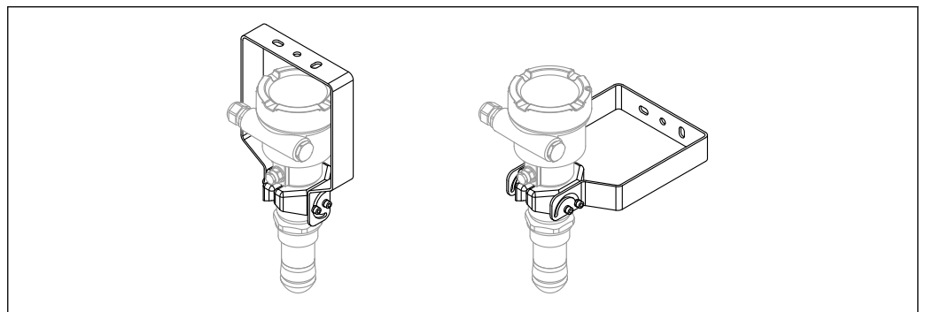
35 Montage sur plafond ou paroi
