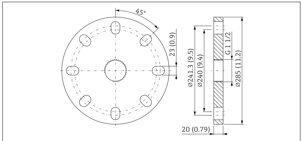
23 Dimensions de la bride UNI 6"/DN150/150A. Unité de mesure mm (in)
