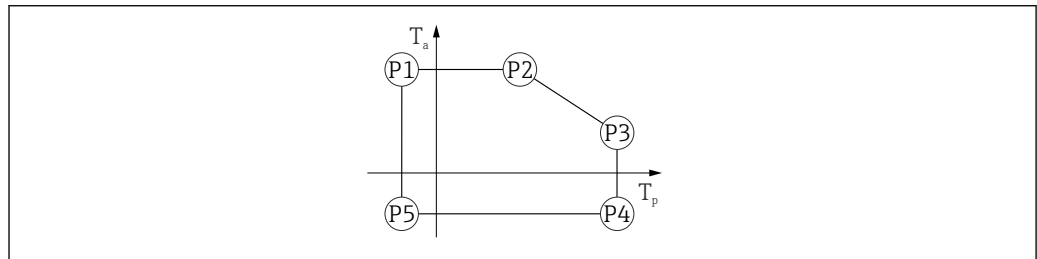
図 14 ハウジング材質：SUS 316L 相当；プロセス温度範囲：-40～+80 °C (-40～+176 °F)
