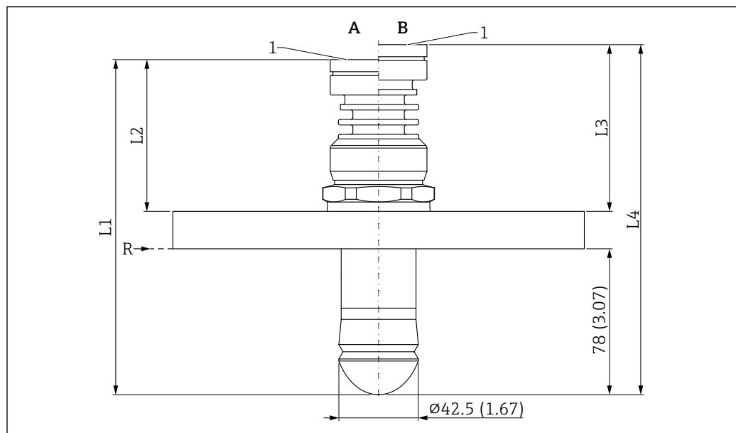
図 25 ドリップオフアンテナ 50 mm (2 in) (UNI フランジプロセス接続) の寸法。測定単位 mm (in)
