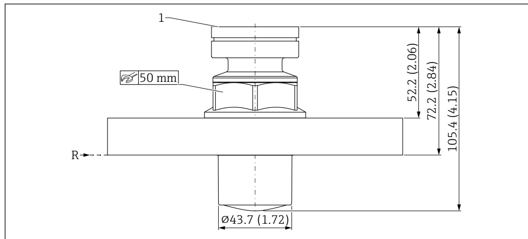
図 20 被覆アンテナ (PVDF、40 mm (1.5 in)、プロセス接続 UNI フランジ) の寸法。測定単位 mm (in)
