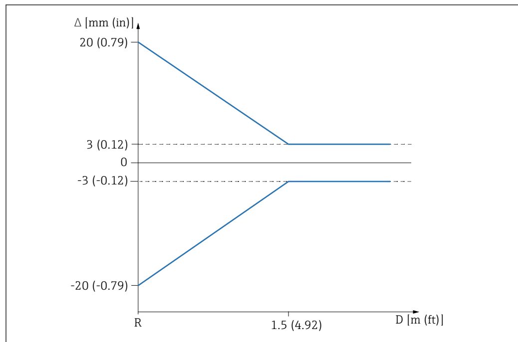
図 6 近範囲アプリケーションにおける最大測定誤差
