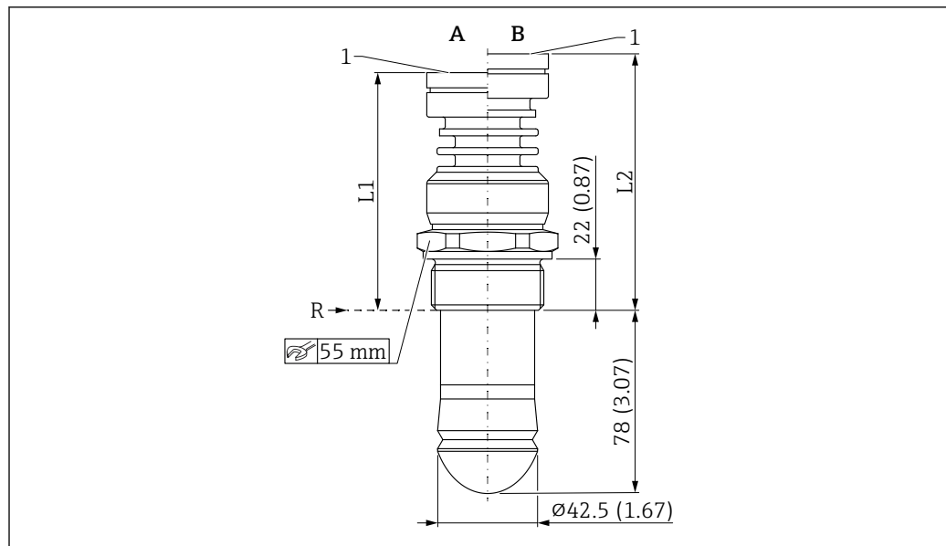
図 24 ドリップオフアンテナ 50 mm (2 in) (ネジ込みプロセス接続) の寸法。測定単位 mm (in)
