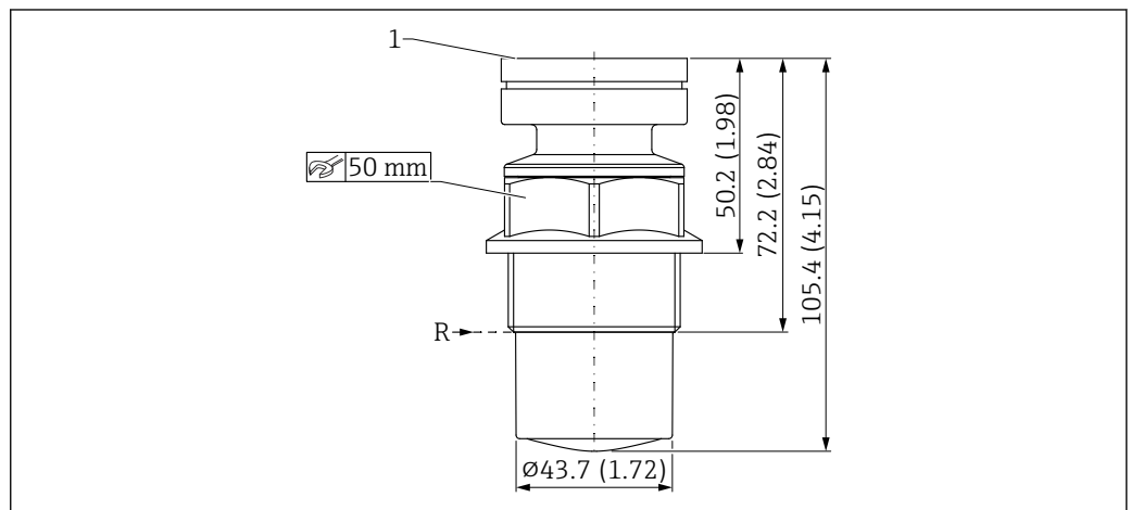
■ 19 被覆アンテナ（PVDF、40 mm (1.5 in)）の寸法。測定単位 mm (in)
