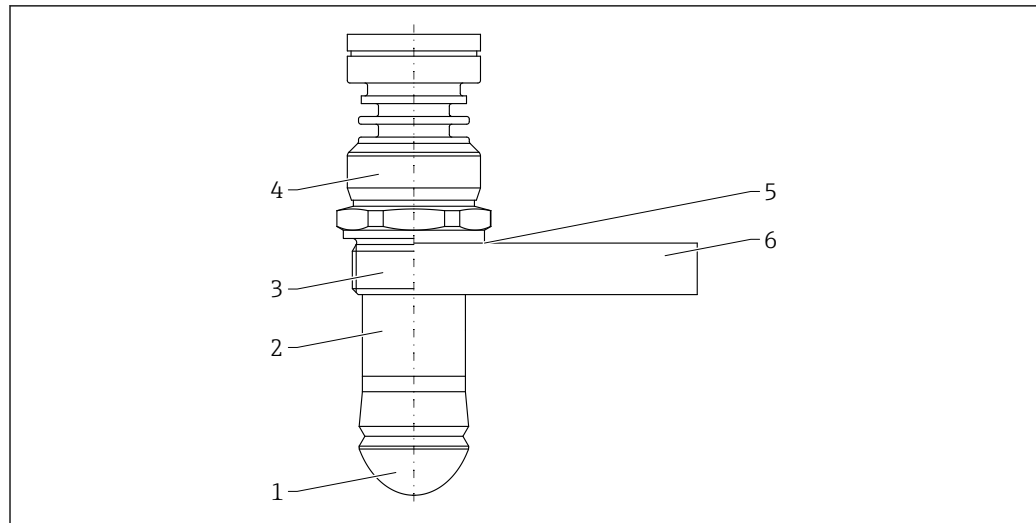
図 30 材質；ドリップオフアンテナ 50 mm (2 in)
