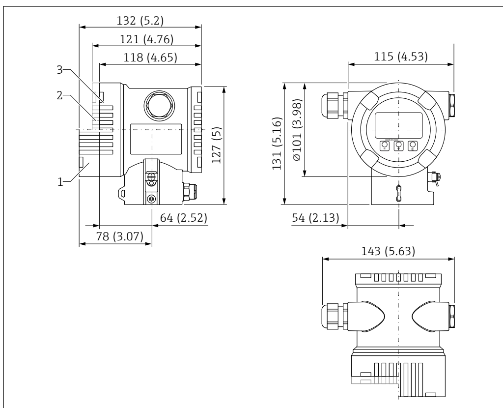
図 17 デュアル端子箱部の寸法
