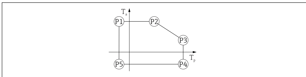
■ 10 ハウジング材質：プラスチック；プロセス温度範囲：-40～+130 °C (-40～+266 °F)
