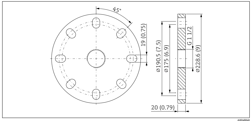
22 UNI フランジ 4"/DN100/100A の寸法。測定単位 mm (in)
