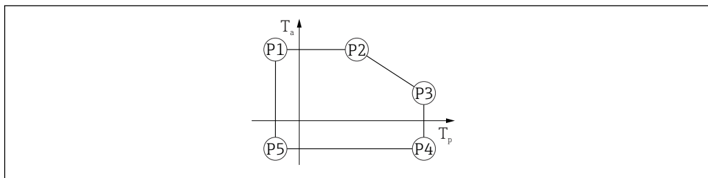
■ 12 ハウジング材質：アルミニウム；プロセス温度範囲：-40～+80 °C (-40～+176 °F)
