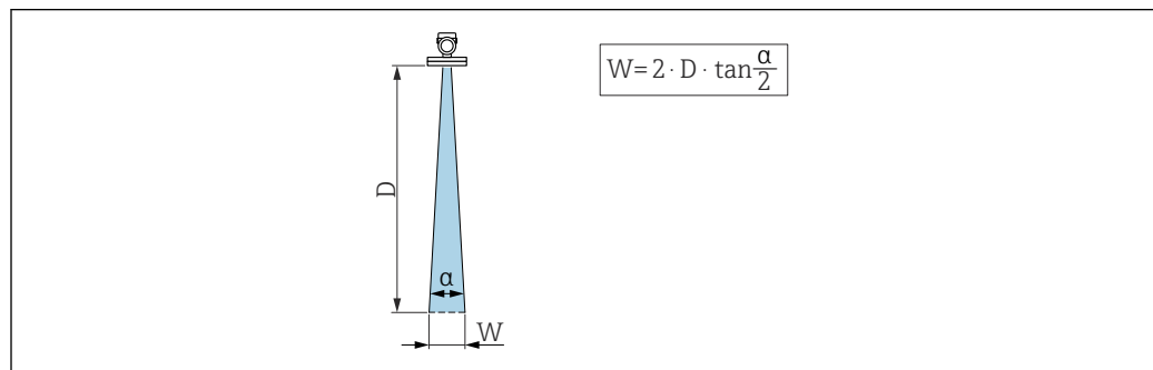
図 7 ビーム放射角 \alpha 、距離 D 、ビーム幅 W の関係
