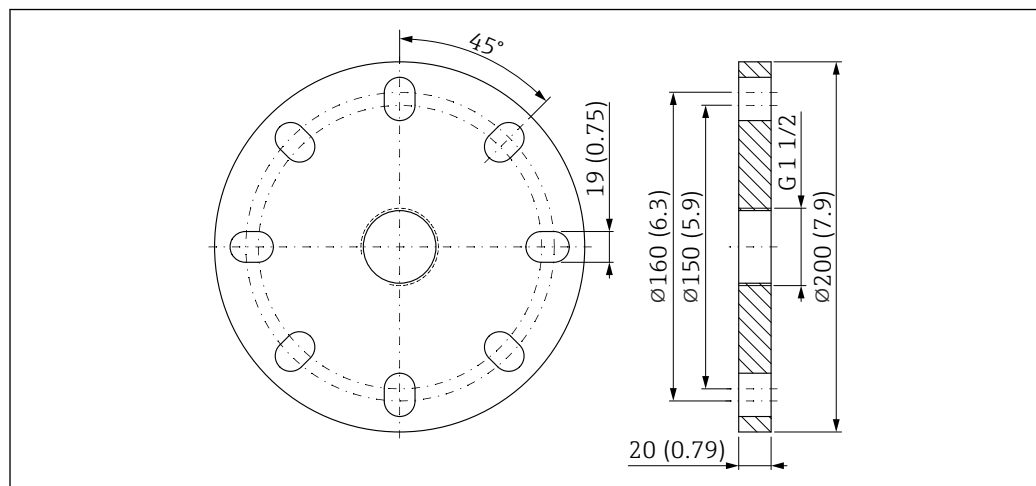
図 21 UNI フランジ 3"/DN80/80A の寸法。測定単位 mm (in)
