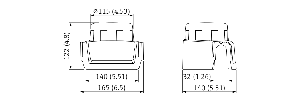
図 34 寸法。測定単位 mm (in)
