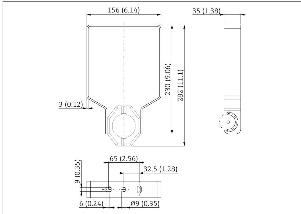
図 36 取付ブラケットの寸法。測定単位 mm (in)
