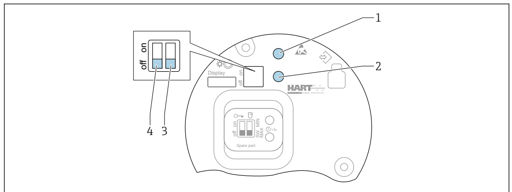
図 31 HART エレクトロニクスインサート上の操作キーおよび DIP スイッチ
