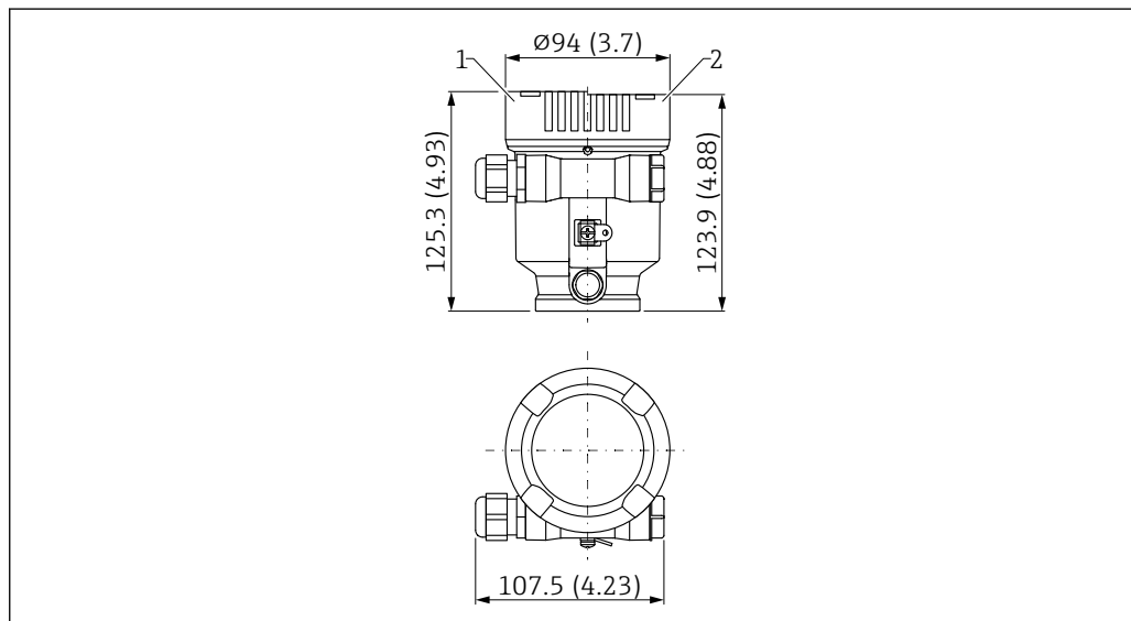
図 15 シングル端子箱部（プラスチック（PBT））の寸法
