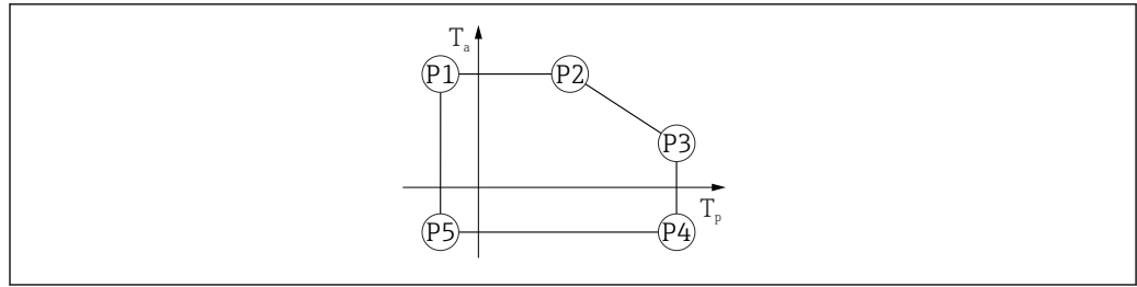
図 13 ハウジング材質：アルミニウム；プロセス温度範囲：-40～+130 °C (-40～+266 °F)
