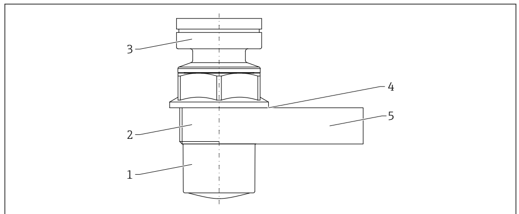
図 29 材質；被覆アンテナ、PVDF、40 mm (1.5 in)
