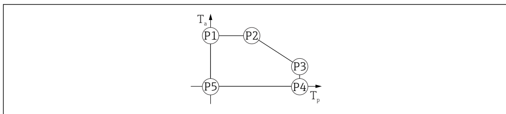
■ 11 ハウジング材質：プラスチック；プロセス温度範囲：0～+130 °C (+32～+266 °F)、CSA C/US 認定付き
