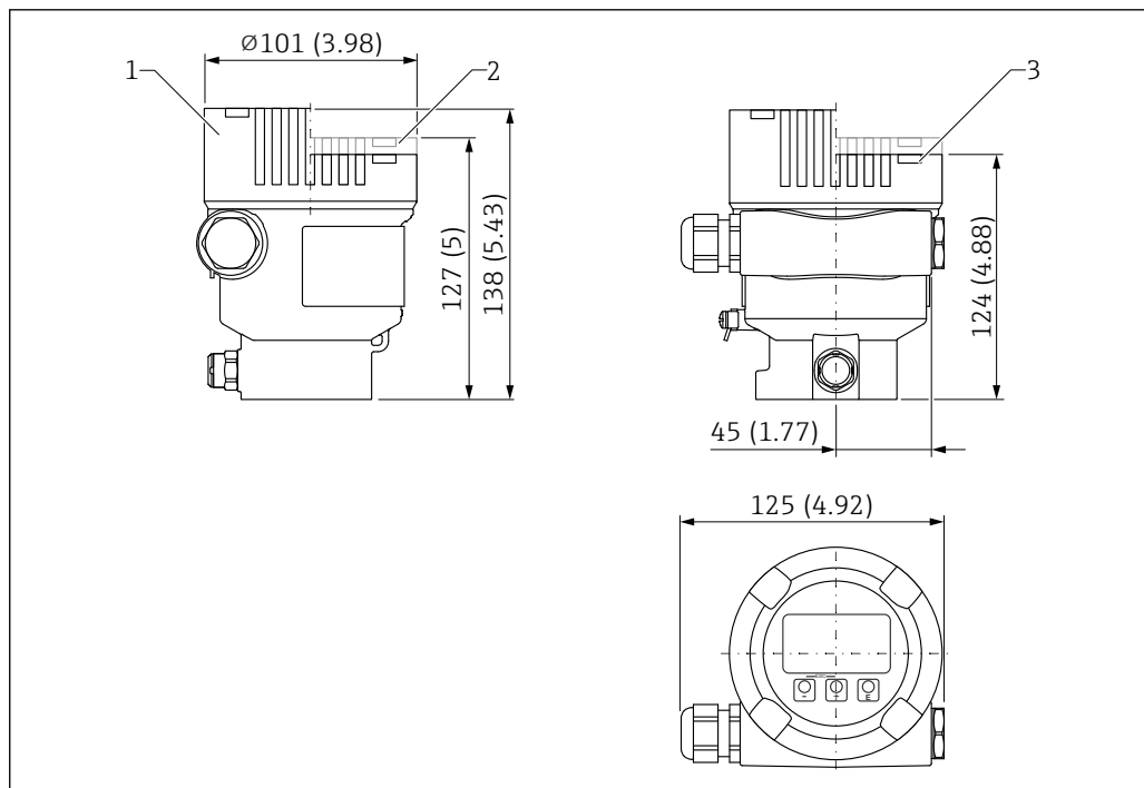
図 16 アルミニウムシングル端子箱部の寸法
