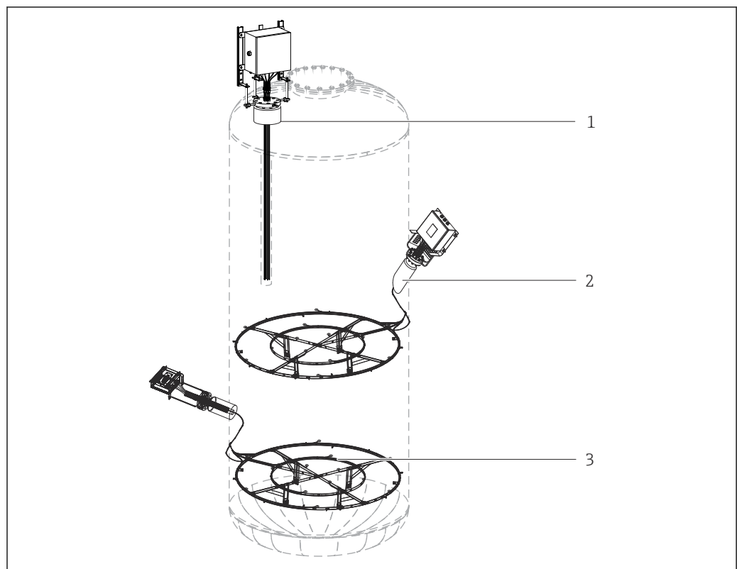
図 10 取付例 - 取付方向に制約なし
