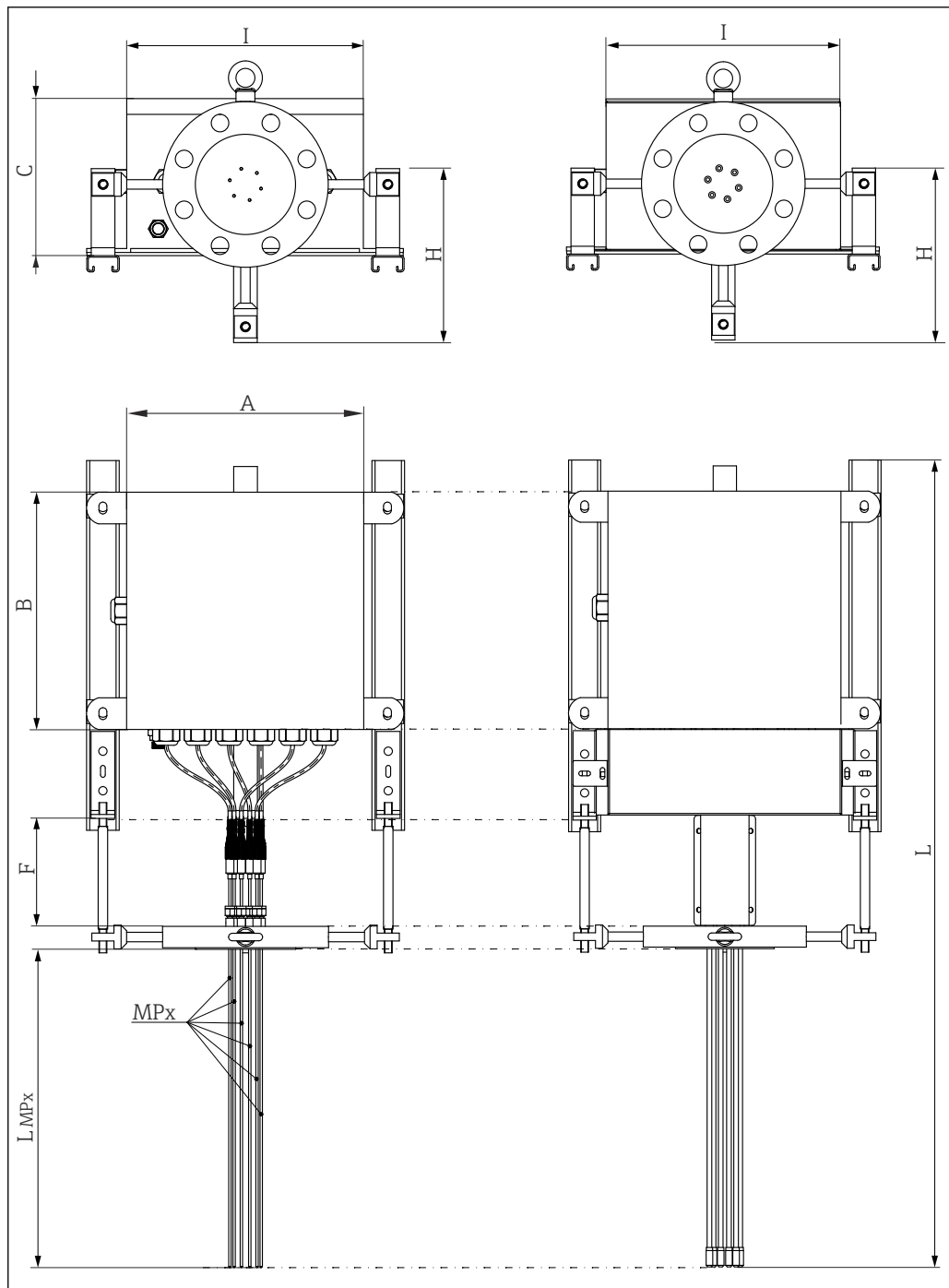
図 12 モジュラー式マルチポイント温度計の構成は、フレームのネックが左側ですが、フレームのネックにカバーがある構成の場合は右側です。全寸法単位は mm (in) です。
