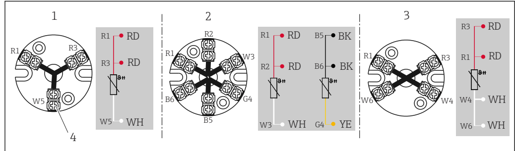
図 3 端子台
