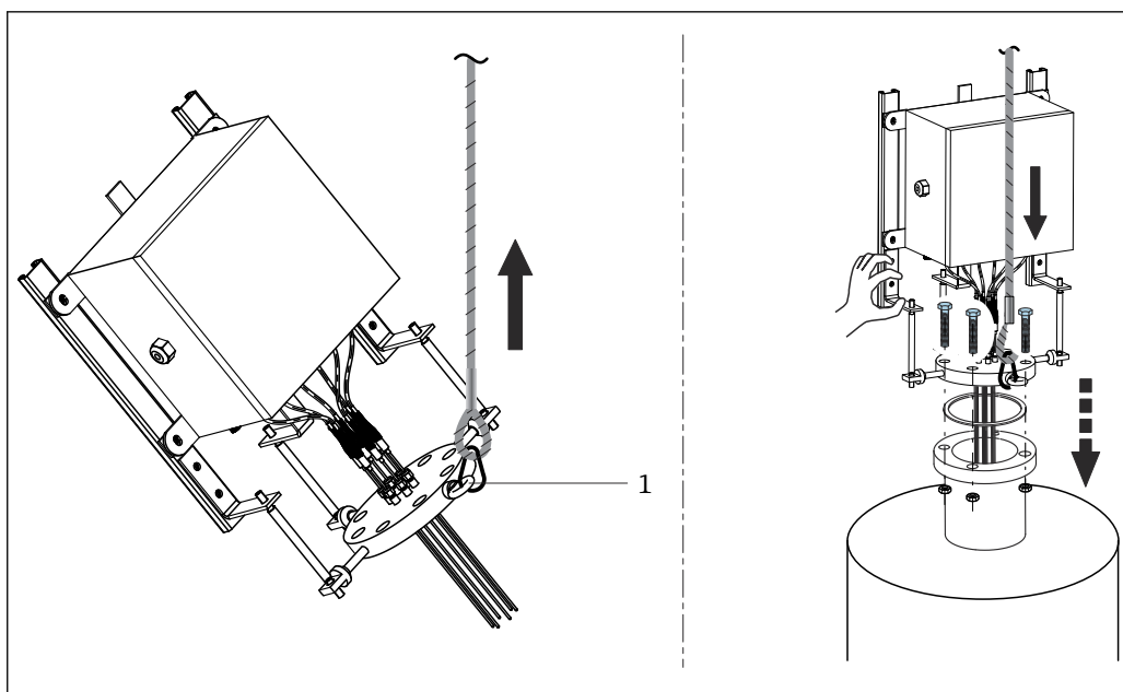
図 11 マルチポイント温度計を、フランジプロセス接続でリアクターノズルに取り付けること。
