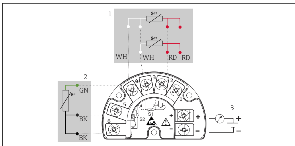
図 7 TMT162 (2 センサ入力)
