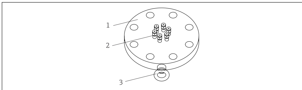
図 13 プロセス接続フランジ
