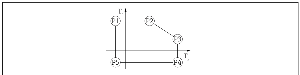
28 Matériau du boîtier alu ; gamme de température de process : -40 \dots +80 \text{ }^{\circ}\text{C} ( -40 \dots +176 \text{ }^{\circ}\text{F} )
