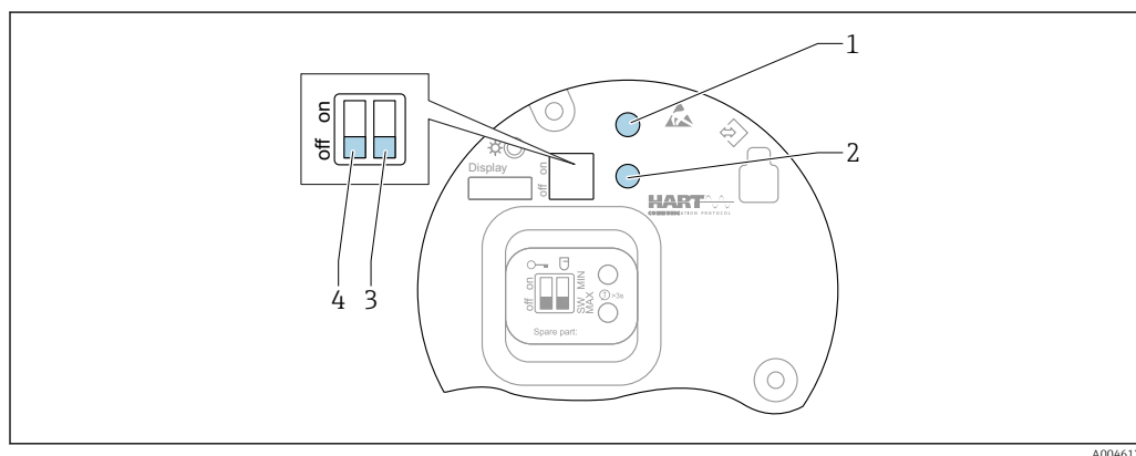
10 Touches de configuration et commutateurs DIP sur l'électronique HART
