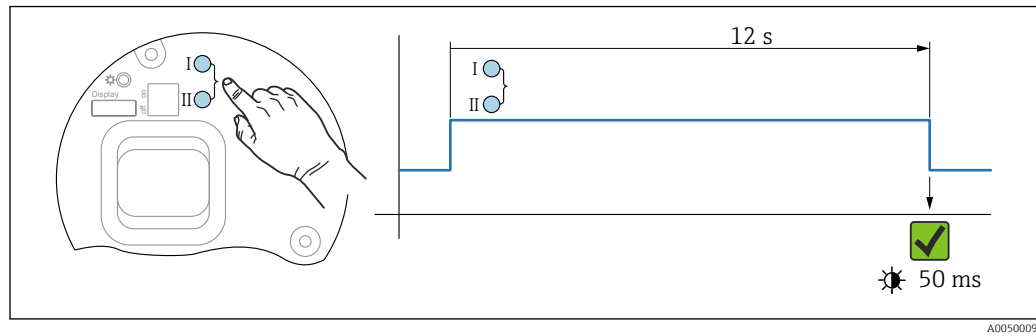
15 Touches de configuration sur l'électronique
