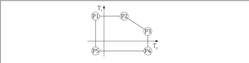
36 Matériau du boîtier 316L ; gamme de température de process : -40 ... +280 °C (-40 ... +536 °F)
