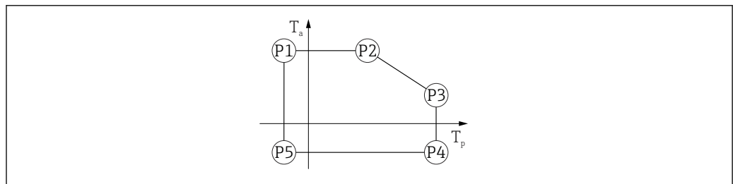
31 Matériau du boîtier alu ; gamme de température de process : -40 ... +280 °C (-40 ... +536 °F)
