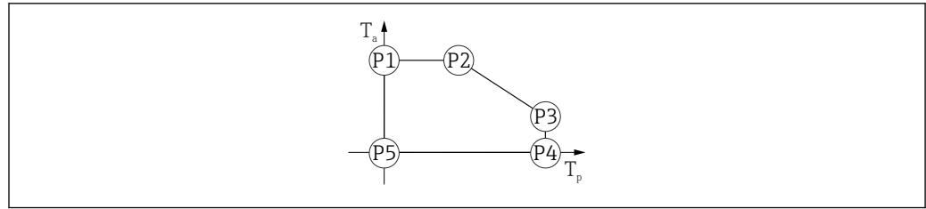
19 Matériau du boîtier plastique ; gamme de température de process : 0 ... +80 °C (+32 ... +176 °F) avec agrément CSA C/US
