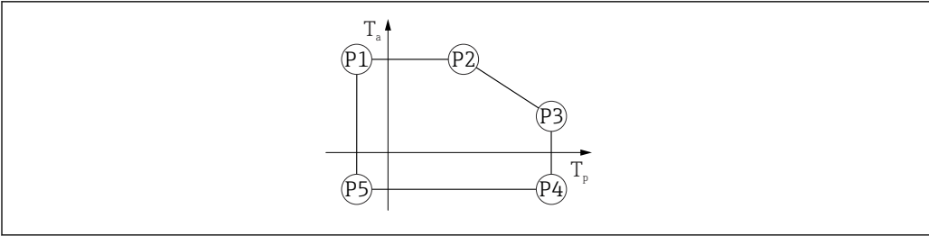
35 Matériau du boîtier 316L ; gamme de température de process : -40 ... +200 °C (-40 ... +392 °F)
