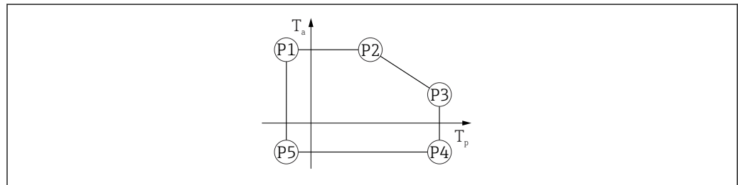
20 Matériau du boîtier plastique ; gamme de température de process : -40 ... +150 °C (-40 ... +302 °F)
