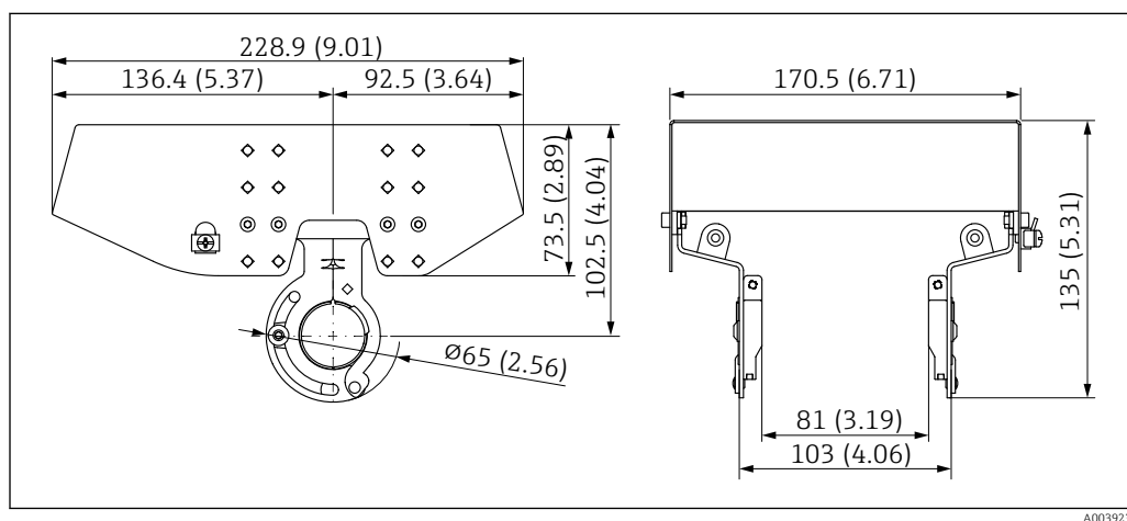
16 Dimensions. Unité de mesure mm (in)
