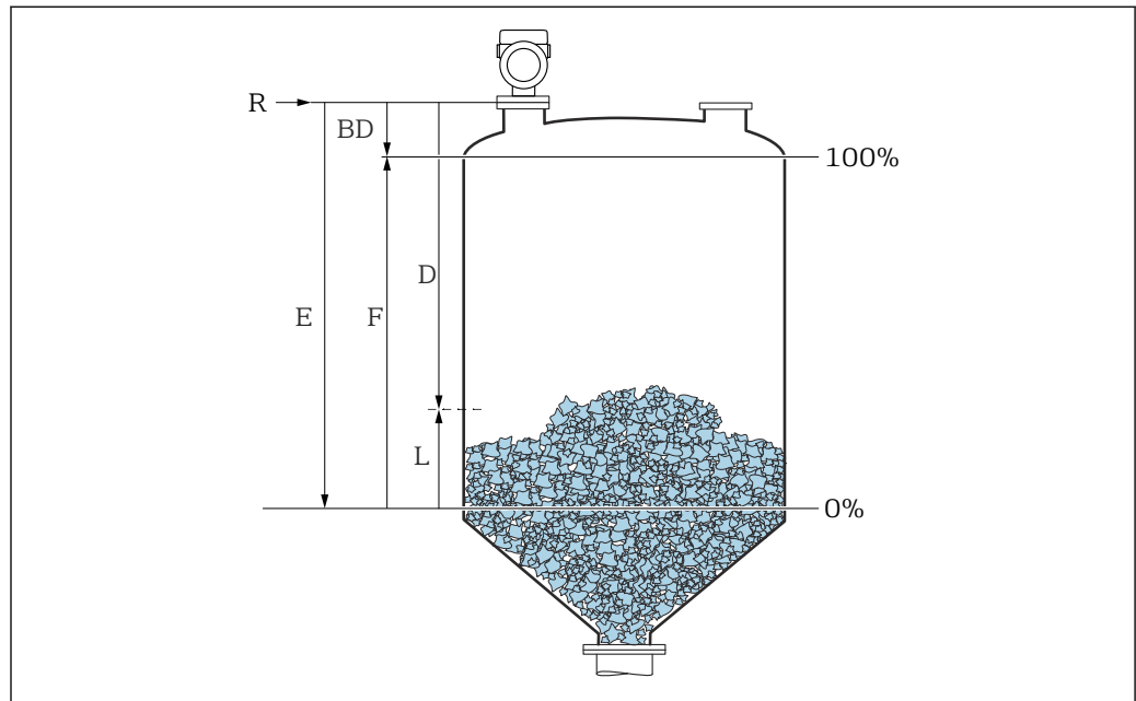
13 Paramètres de configuration pour la mesure de niveau dans les solides en vrac
