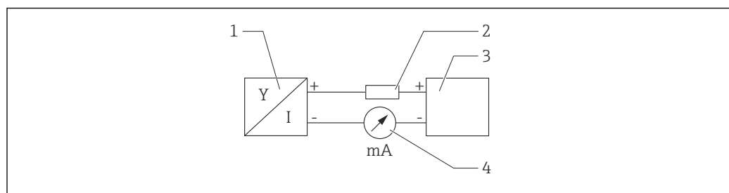
6 Schéma de principe du raccordement HART
