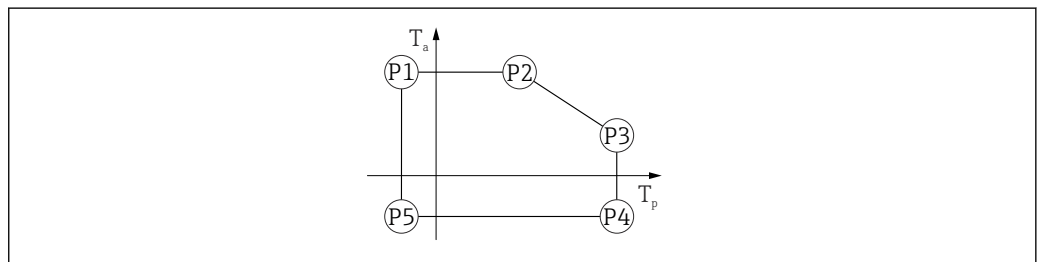
34 Matériau du boîtier 316L ; gamme de température de process : -40 \dots +150 \text{ °C} ( -40 \dots +302 \text{ °F} )
