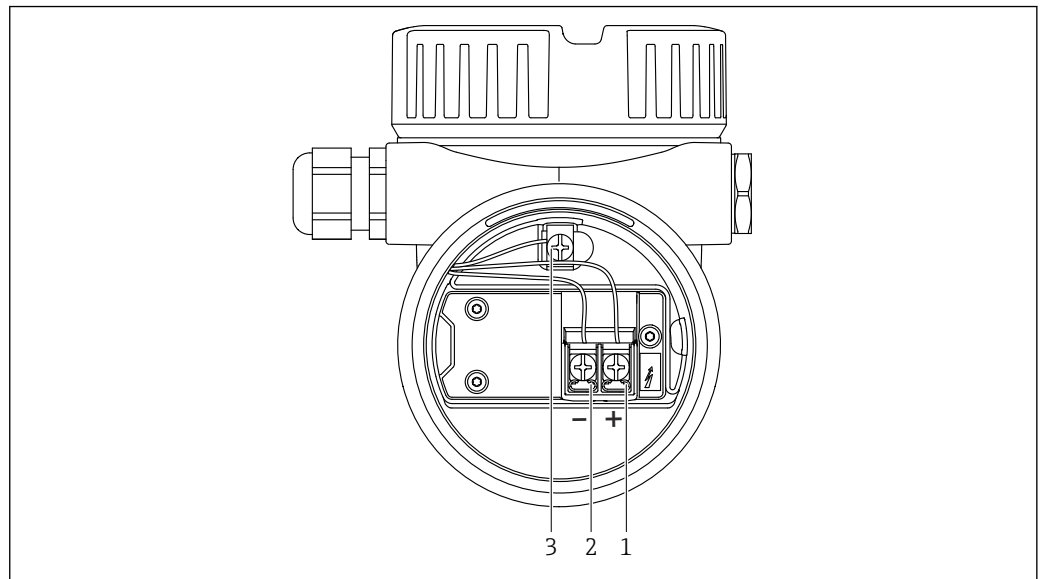
9 Bornes de raccordement et borne de terre dans le compartiment de raccordement
