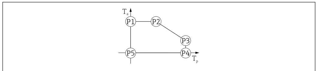
23 Matériau du boîtier plastique ; gamme de température de process : 0 \dots +200 \text{ °C} ( +32 \dots +392 \text{ °F} ) avec agrément CSA C/US
