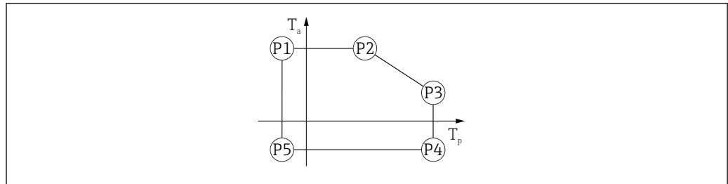
30 Matériau du boîtier alu ; gamme de température de process : -40 ... +200 °C (-40 ... +392 °F)
