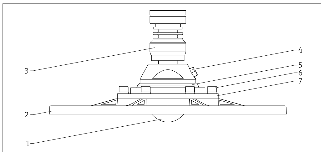
59 Matériau, antenne affleurante, 80 mm (3 in), avec bride UNI, dispositif d'orientation et raccord d'air de purge
