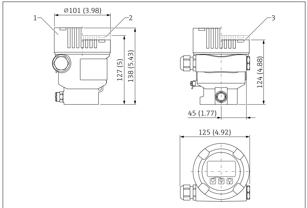
32 Dimensions du boîtier à simple compartiment en alu
