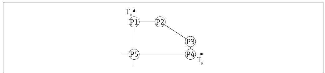
■ 16 Matériau du boîtier plastique ; gamme de température de process : 0 ... +200 °C (+32 ... +392 °F) avec agrément CSA C/US
