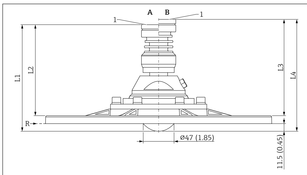
49 Dimensions de l'antenne affleurante, 80 mm (3 in), avec bride UNI, dispositif d'orientation et raccord d'air de purge. Unité de mesure mm (in)
