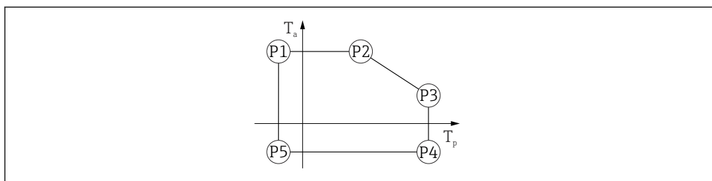
21 Matériau du boîtier alu ; gamme de température de process : -40 \dots +80 \text{ }^{\circ}\text{C} ( -40 \dots +176 \text{ }^{\circ}\text{F} )
