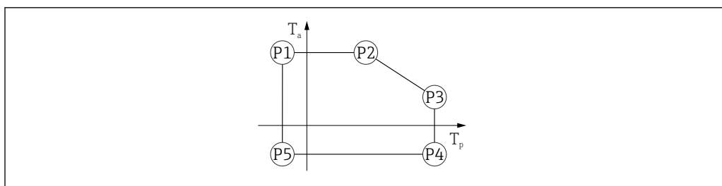
19 Matériau du boîtier plastique ; gamme de température de process : -40 \dots +450 \text{ }^{\circ}\text{C} ( -40 \dots +842 \text{ }^{\circ}\text{F} )
