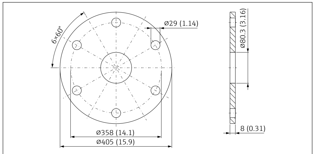
48 Dimensions de la bride UNI 10"/DN250/250A pour antenne DN80 avec raccord d'air de purge. Unité de mesure mm (in)
