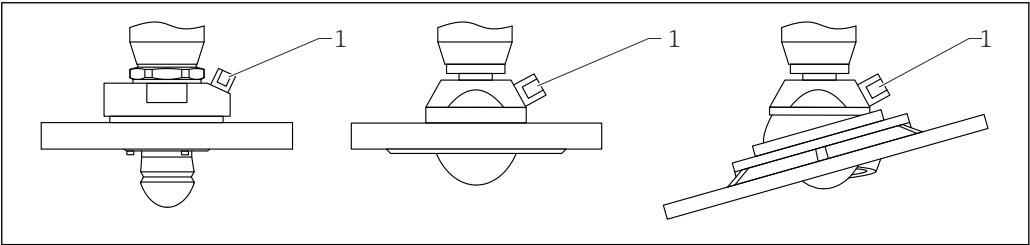
9 Antenne avec adaptateur d'air de purge
