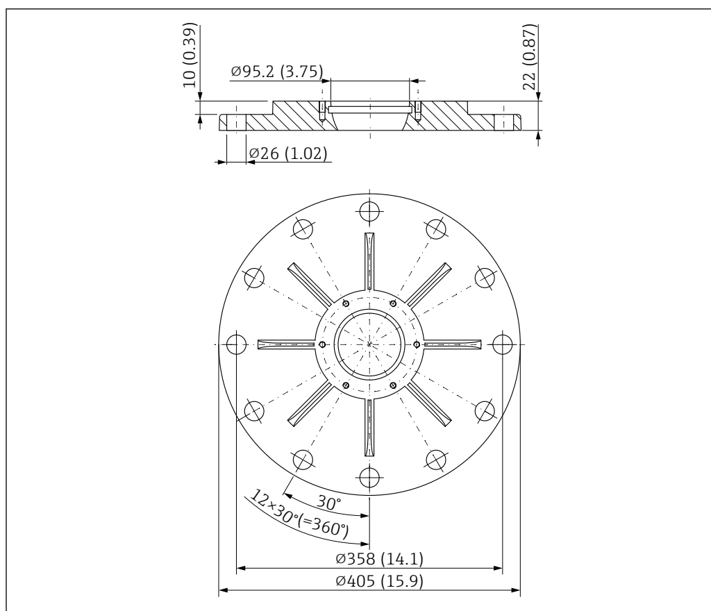
40 Dimensions de la bride UNI 10"/DN250/250A pour antennes avec dispositif d'orientation. Unité de mesure mm (in)
