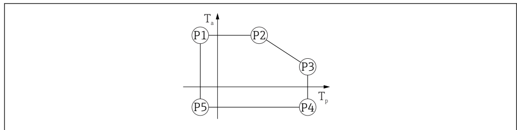
26 Matériau du boîtier 316L ; gamme de température de process : -40 \dots +80 \text{ °C} ( -40 \dots +176 \text{ °F} )
