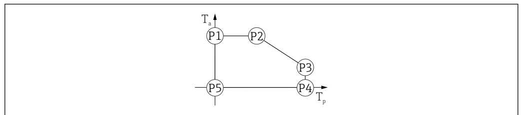
■ 18 Matériau du boîtier plastique ; gamme de température de process : 0 ... +280 °C (+32 ... +536 °F) avec agrément CSA C/US
