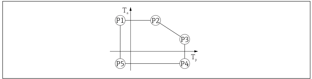
11 Matériau du boîtier plastique ; gamme de température de process : -40 \dots +80 \text{ }^{\circ}\text{C} ( -40 \dots +176 \text{ }^{\circ}\text{F} )
