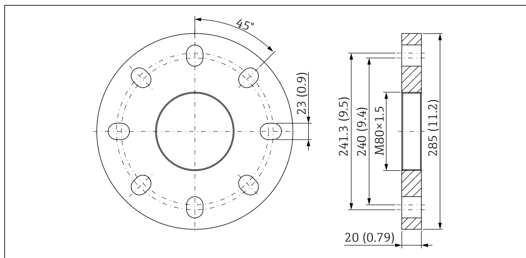
44 Bride UNI 6"/DN150/150A pour antenne drip-off, PTFE, 50 mm (2 in) avec raccord d'air de purge. Unité de mesure mm (in)
