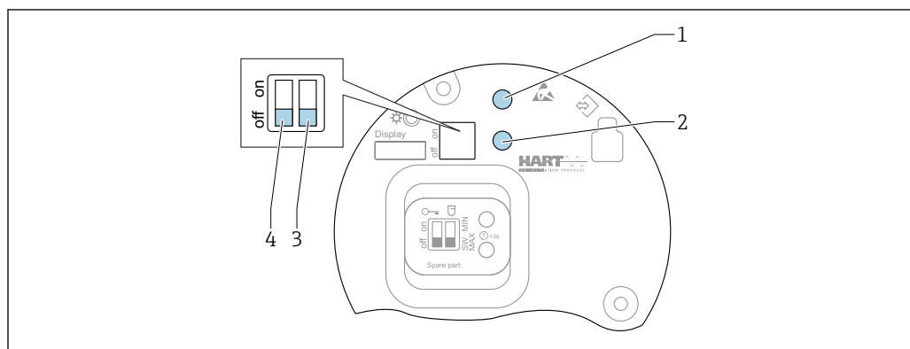
60 Touches de configuration et commutateurs DIP sur l'électronique HART
