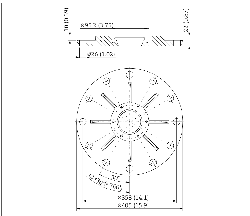
53 Dimensions de la bride UNI 10"/DN250/250A pour antennes avec dispositif d'orientation. Unité de mesure mm (in)
