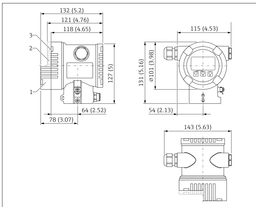
33 Dimensions du boîtier à double compartiment
