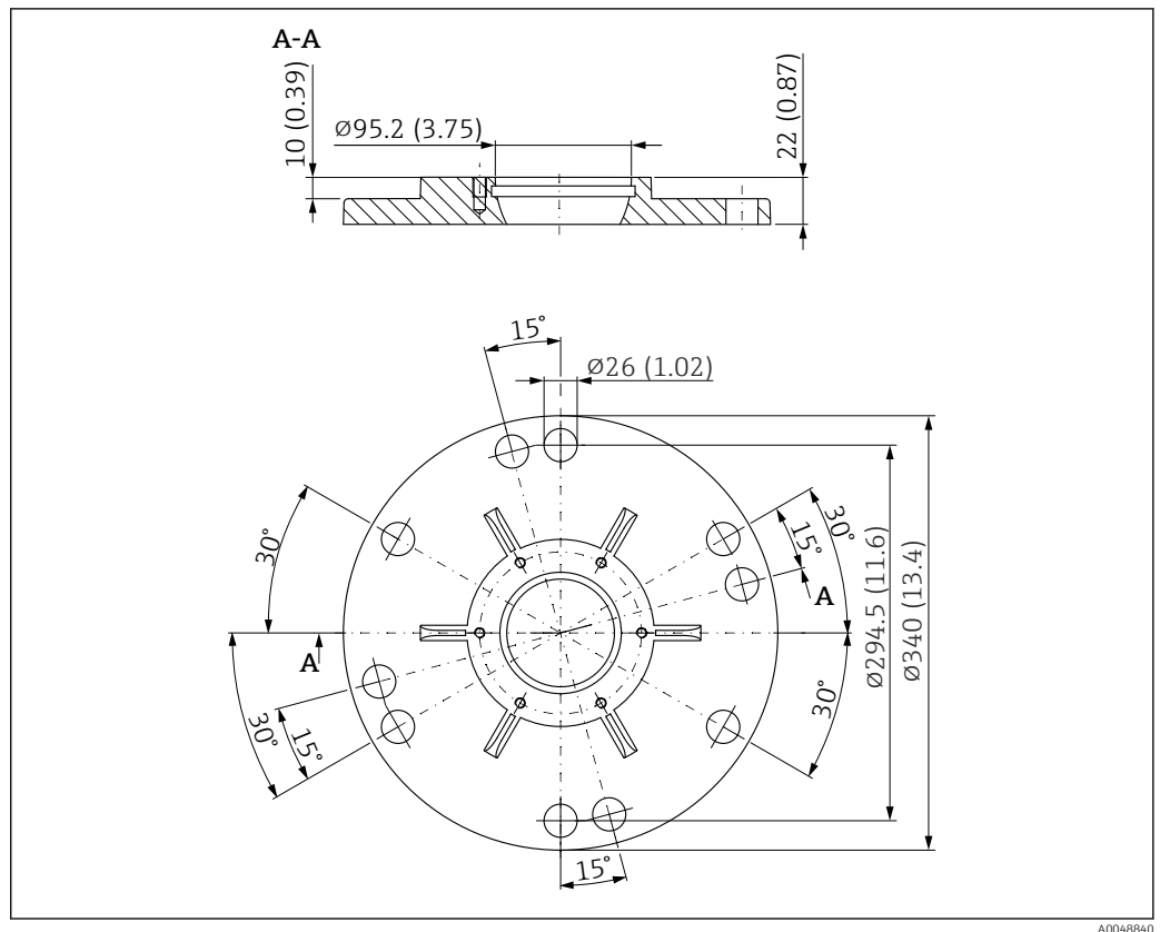
52 Dimensions de la bride UNI 8"/DN200/200A pour antennes avec dispositif d'orientation. Unité de mesure mm (in)
