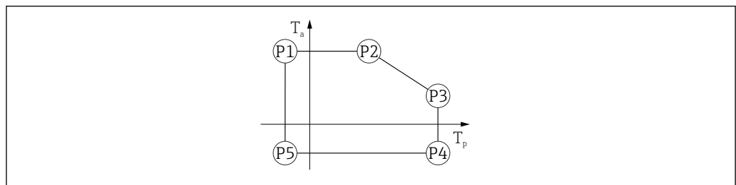
27 Matériau du boîtier 316L ; gamme de température de process : -40 \dots +150 \text{ °C} ( -40 \dots +302 \text{ °F} )
