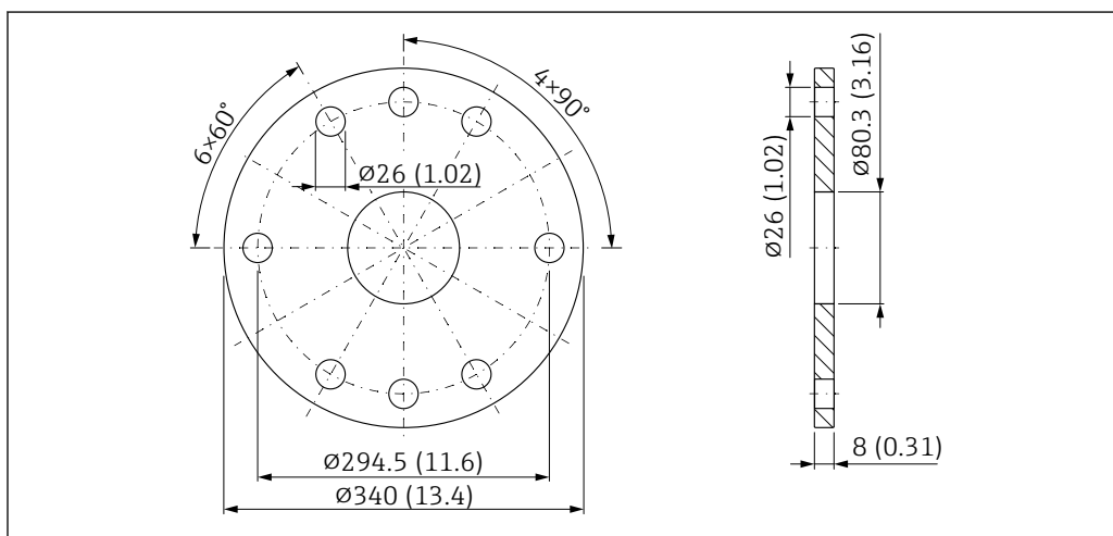
47 Dimensions de la bride UNI 8"/DN200/200A pour antenne DN80 avec raccord d'air de purge. Unité de mesure mm (in)
