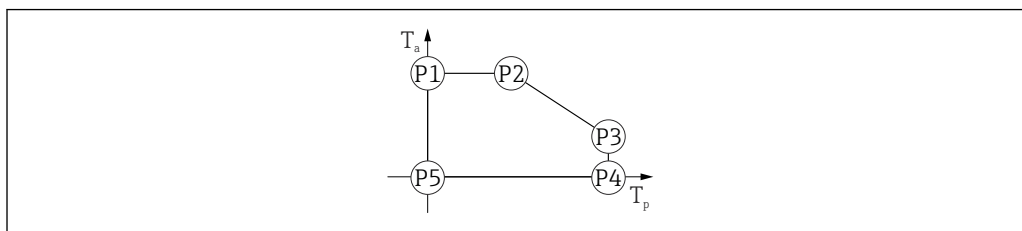
20 Matériau du boîtier plastique ; gamme de température de process : 0 \dots +450 \text{ }^{\circ}\text{C} ( +32 \dots +842 \text{ }^{\circ}\text{F} ) avec agrément CSA C/US
