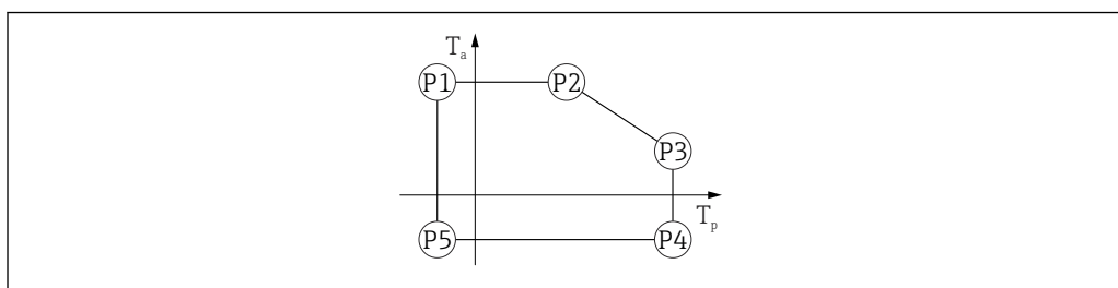
15 Matériau du boîtier plastique ; gamme de température de process : -40 \dots +200 \text{ }^{\circ}\text{C} ( -40 \dots +392 \text{ }^{\circ}\text{F} )
