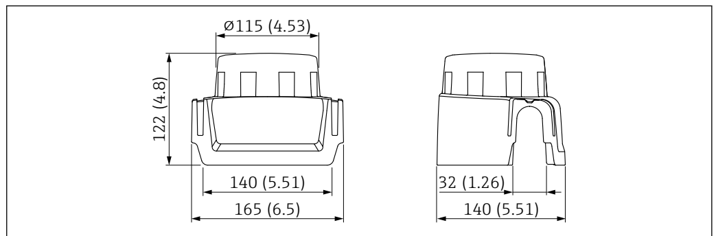
63 Dimensions. Unité de mesure mm (in)
