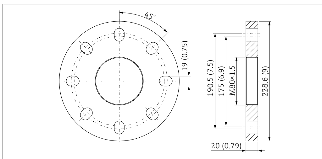
43 Bride UNI 4"/DN100/100A pour antenne drip-off, PTFE, 50 mm (2 in) avec raccord d'air de purge. Unité de mesure mm (in)
