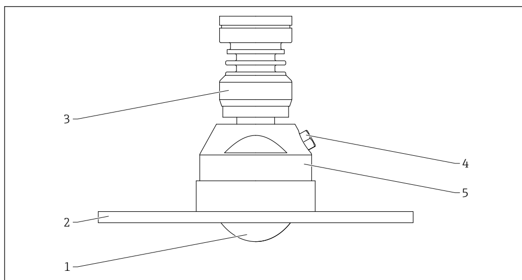
58 Matériau ; antenne affleurante, 80 mm (3 in), avec bride UNI et raccord d'air de purge. Unité de mesure mm (in)
