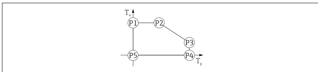
14 Matériau du boîtier plastique ; gamme de température de process : 0 \dots +150 \text{ }^{\circ}\text{C} ( +32 \dots +302 \text{ }^{\circ}\text{F} ) avec agrément CSA C/US
