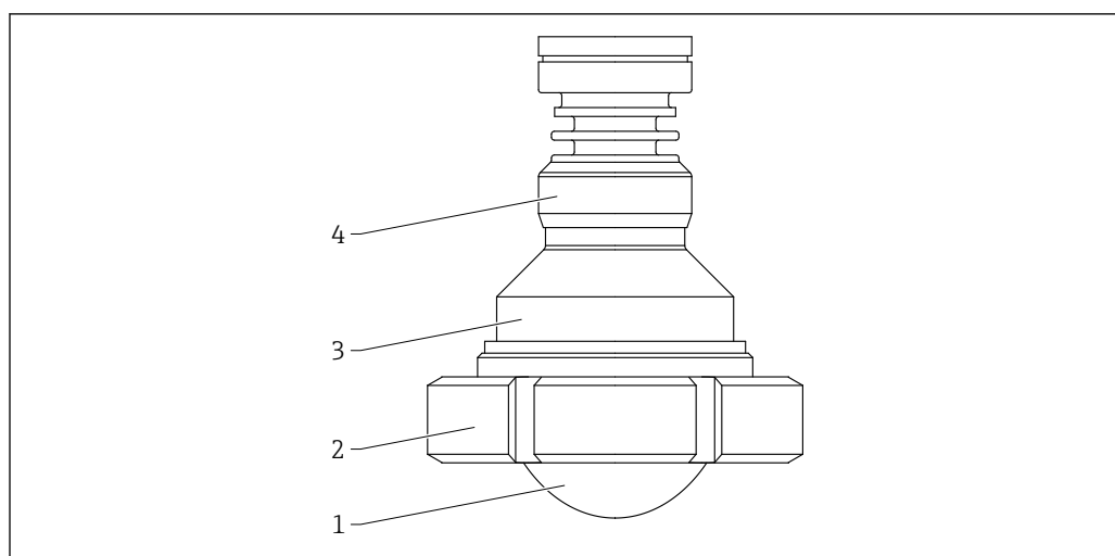
36 Matériau ; antenne, plaquée, affleurante, 80 mm (3 in), écrou fou DIN11851. Unité de mesure mm (in)
