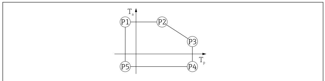
16 Matériau du boîtier alu ; gamme de température de process : -20 ... +150 °C (-4 ... +302 °F)
