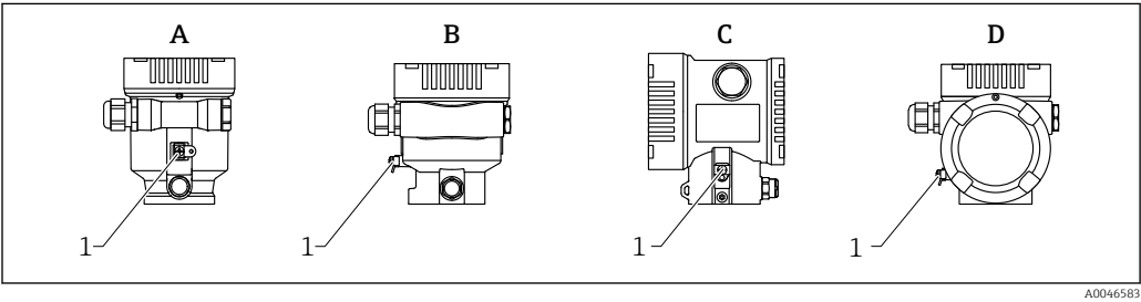
A Boîtier à compartiment unique, plastique B Boîtier à compartiment unique, aluminium C Boîtier à compartiment double D Boîtier à compartiment double, en L 1 Borne de terre pour le raccordement du câble d'équipotentialité
