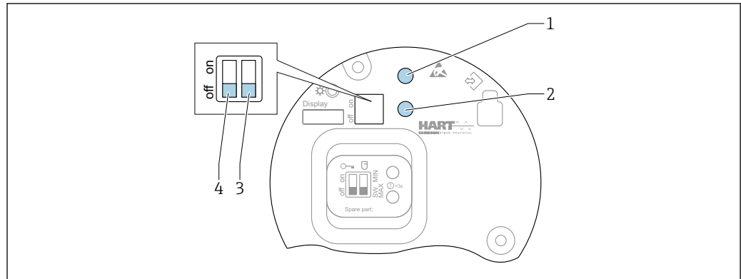
39 Touches de configuration et commutateurs DIP sur l'électronique HART
