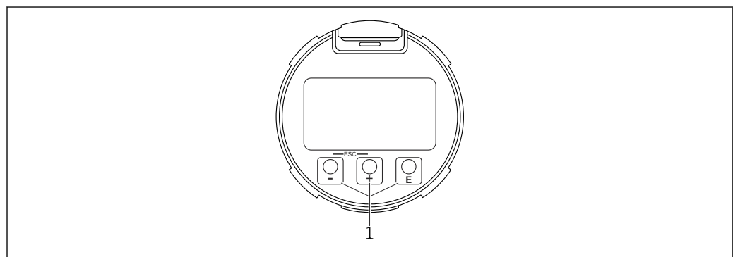
40 Affichage graphique avec touches de configuration optiques (1)
