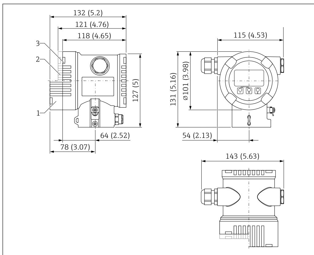
26 Dimensions du boîtier à double compartiment
