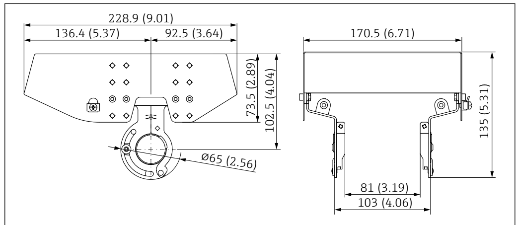
41 Dimensions. Unité de mesure mm (in)
