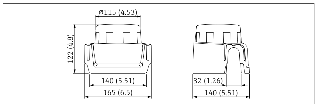
42 Dimensions. Unité de mesure mm (in)
