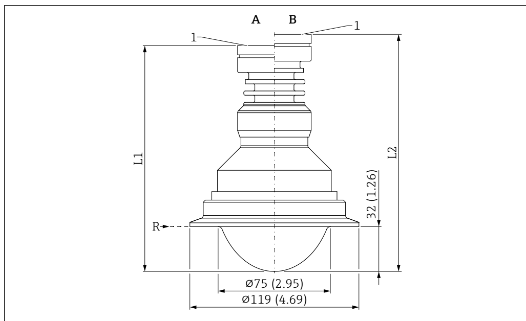
33 Dimensions de l'antenne, plaquée PTFE, affleurante, 80 mm (3 in), avec Tri-Clamp DN101.6 (4") ISO2852. Unité de mesure mm (in)
