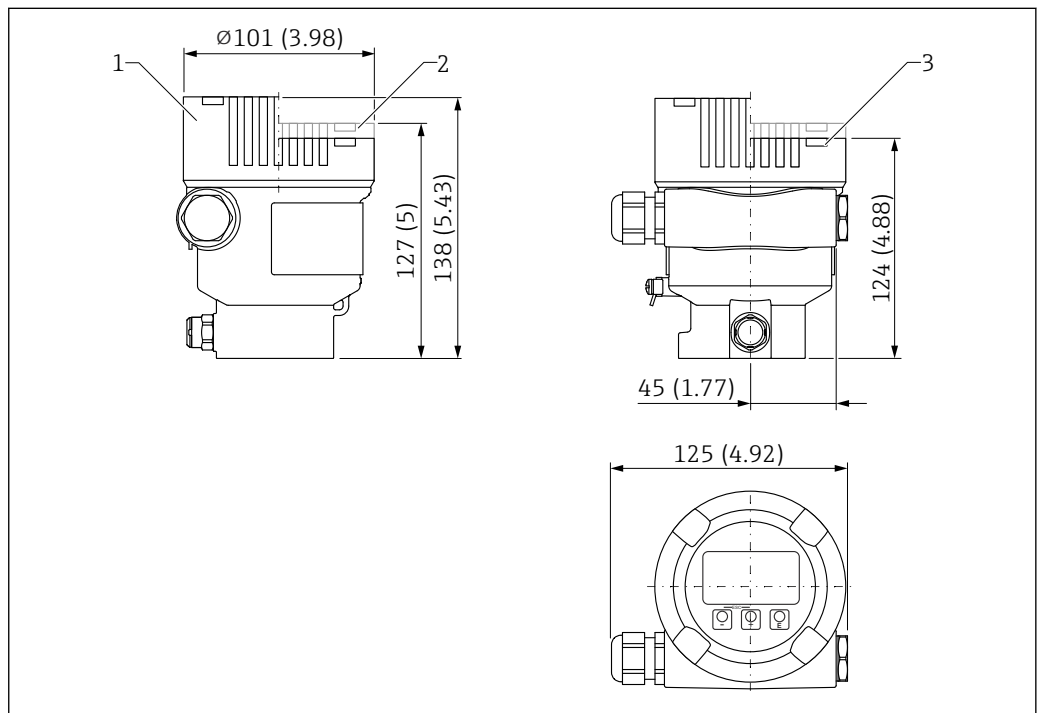
25 Dimensions du boîtier à simple compartiment en alu
