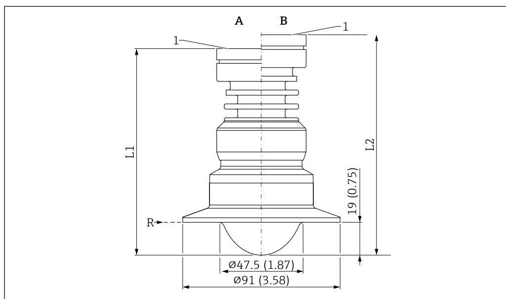
32 Dimensions de l'antenne, plaquée PTFE, affleurante, 50 mm (2 in), avec Tri-Clamp DN70-76.1 (3") ISO2852. Unité de mesure mm (in)
