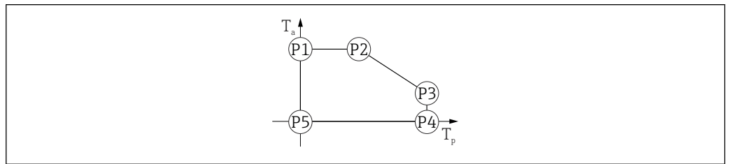
15 Matériau du boîtier plastique ; gamme de température de process : 0 ... +200 °C (+32 ... +392 °F) avec agrément CSA C/US
