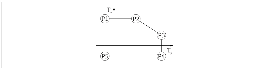
8 Matériau du boîtier plastique ; gamme de température de process : -20 \dots +150 \text{ }^{\circ}\text{C} ( -4 \dots +302 \text{ }^{\circ}\text{F} )
