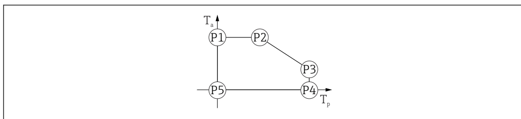
9 Matériau du boîtier plastique ; gamme de température de process : 0 \dots +150 \text{ }^{\circ}\text{C} ( +32 \dots +302 \text{ }^{\circ}\text{F} ) avec agrément CSA C/US
