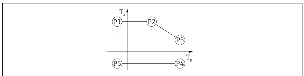
17 Matériau du boîtier alu ; gamme de température de process : -20 ... +200 °C (-4 ... +392 °F)
