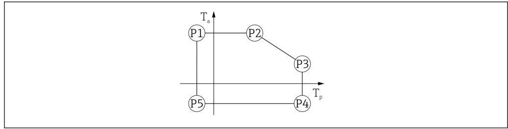
18 Matériau du boîtier alu ; gamme de température de process : -40 \dots +150 \text{ }^{\circ}\text{C} ( -40 \dots +302 \text{ }^{\circ}\text{F} )
